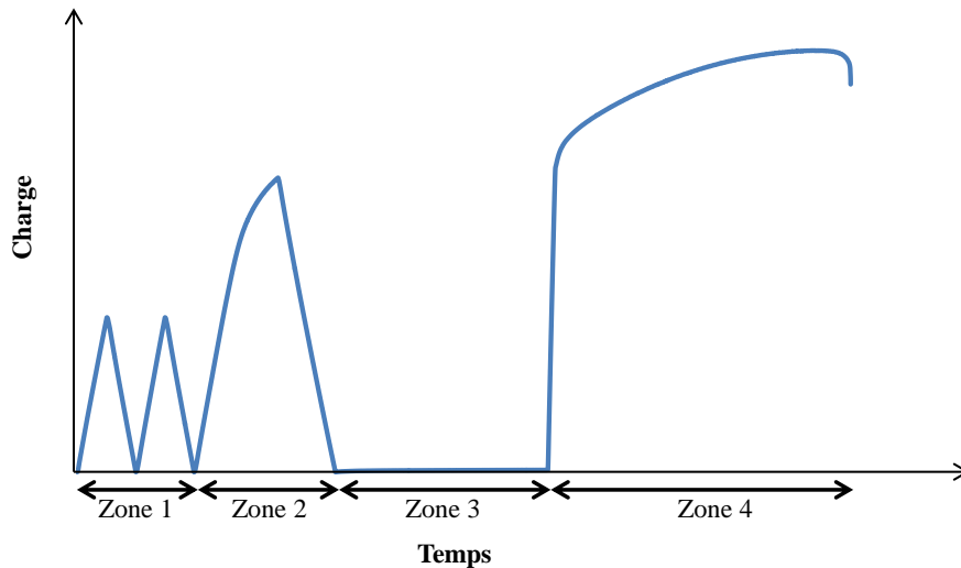
Figure II-12: Courbe de charge typique suivie pour les essais de traction
