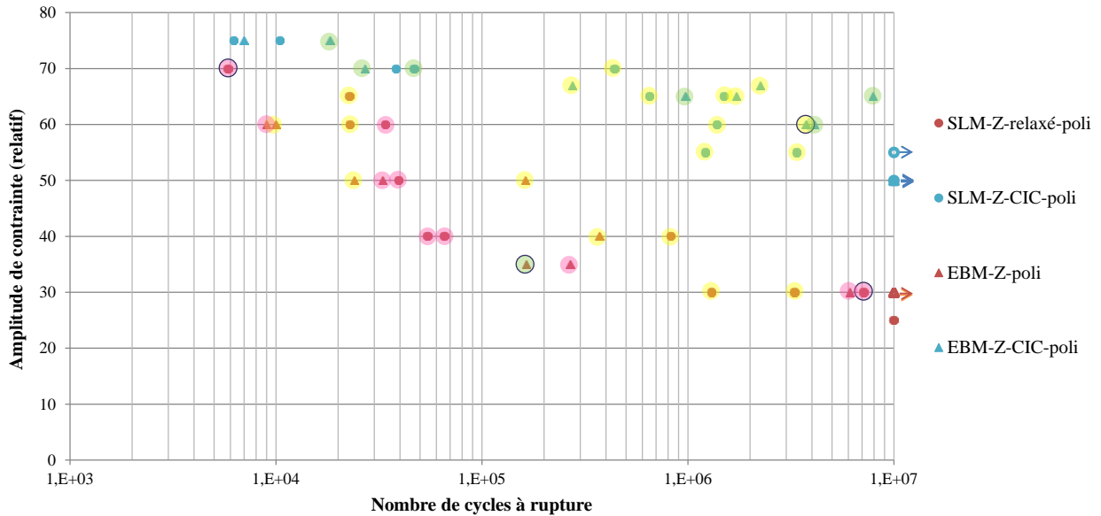
Figure III-30: Résultats des fractographies intégrées aux résultats de fatigue à grand nombre de cycles : effet du traitement CIC
