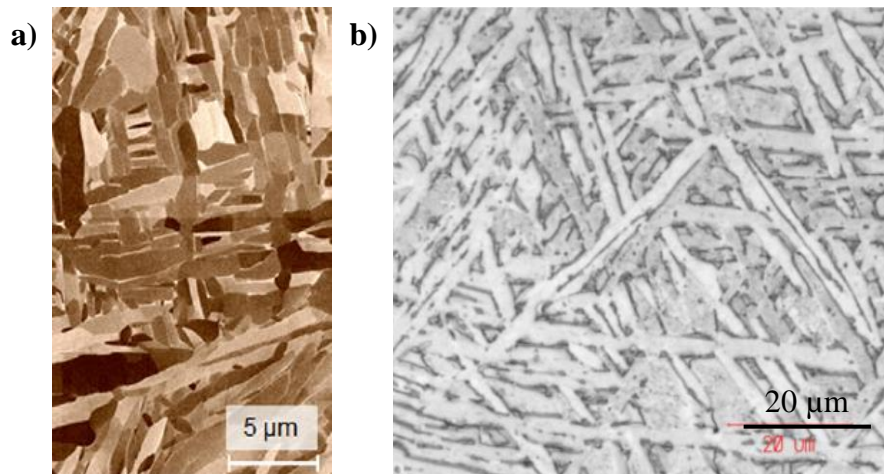
Figure I-23: Images optiques montrant la microstructure du Ti-6Al-4V après traitement CIC pour des échantillons fabriqués par (a) SLM [79] et (b) EBM [74]
