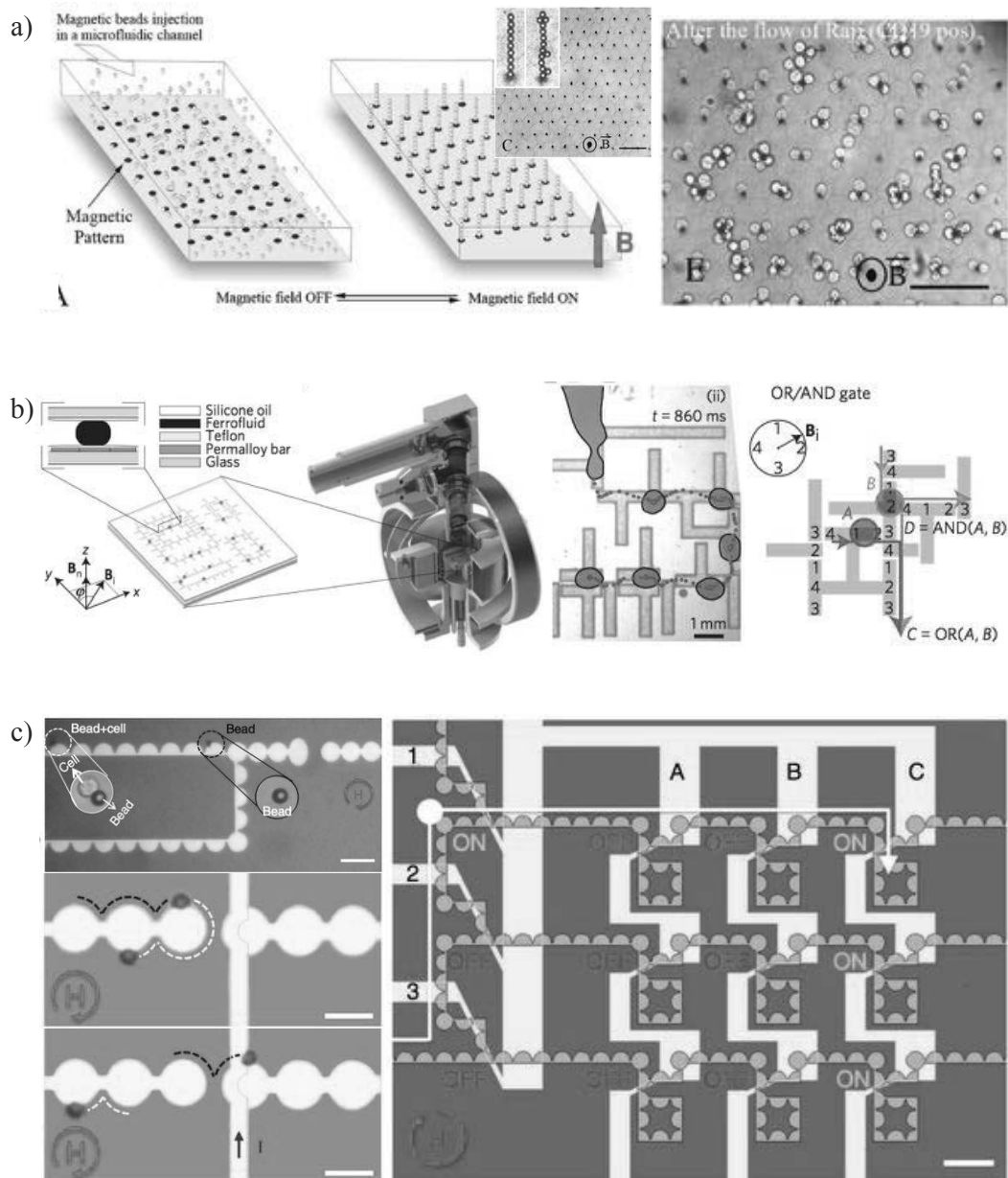
FIGURE 1.23 – Bobines externes, micro-structures (a) et (b) ainsi que micro-bobines (c). a) Système "Ephésia" pour le piégeage de cellules par un réseau de colonnes de micro-billes [41]. b) Calcul booléen avec des gouttes de ferrofluides en utilisant des champs magnétiques tournant planaire et vertical. Exemple de génération de goutte et de porte logique OU/ET [163]. c) Déplacement de billes et cellules marquées le long de structures magnétiques avec un champ tournant, et contrôle du passage de structures (transistor) par injection de courant dans une micro-bobine de type fil. Image de cellules de stockage [164].
