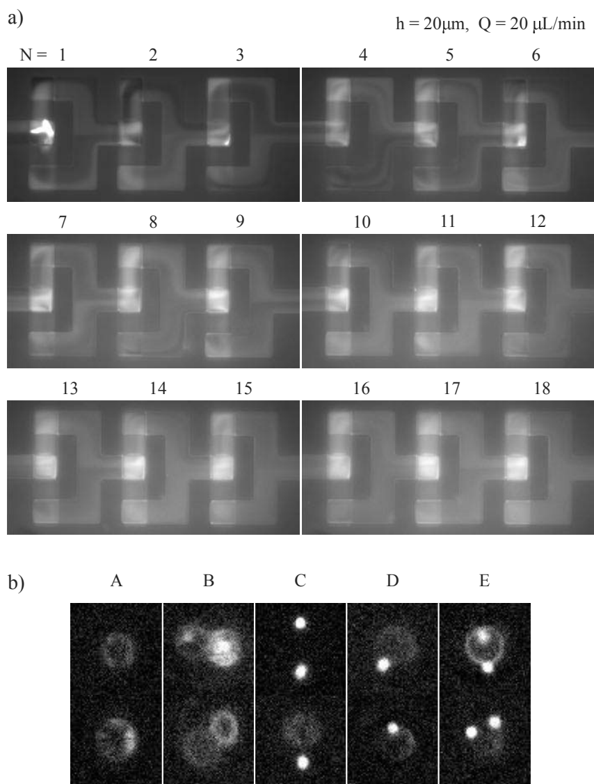
FIGURE 2.9 – Expériences de mélange de particules et de marquage de cellules. a) Images de fluorescence de différents étages d'un mélangeur (solutions : eau et particules de diamètre 500\text{ nm} ) à un débit de 20\mu\text{L}\cdot\text{min}^{-1} et d'une hauteur de canaux de 20\mu\text{m} . b) Images de microscopie en champ clair de monocytes, billes (diamètre 5\mu\text{m} ), et cellules marquées. A : cellules seules, B : cellules attachées ou en division, C : billes isolées et cellule proche d'une bille mais non marquée, D : cellules marquées (1 bille), E : cellules marquées (2 billes).
