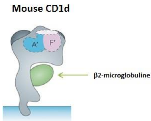
Figure 4: Représentation en 2 dimensions de la molécule CD1d murine
