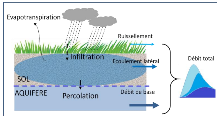
Figure 20: Représentation schématique des mouvements de l'eau lors de la percolation
