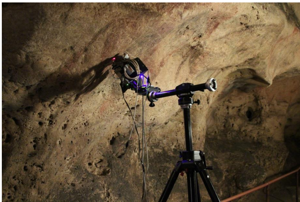
Figure IV. 35 : Spectromètre de FX portable face au bison 43 (© Gay M./LAMS).
