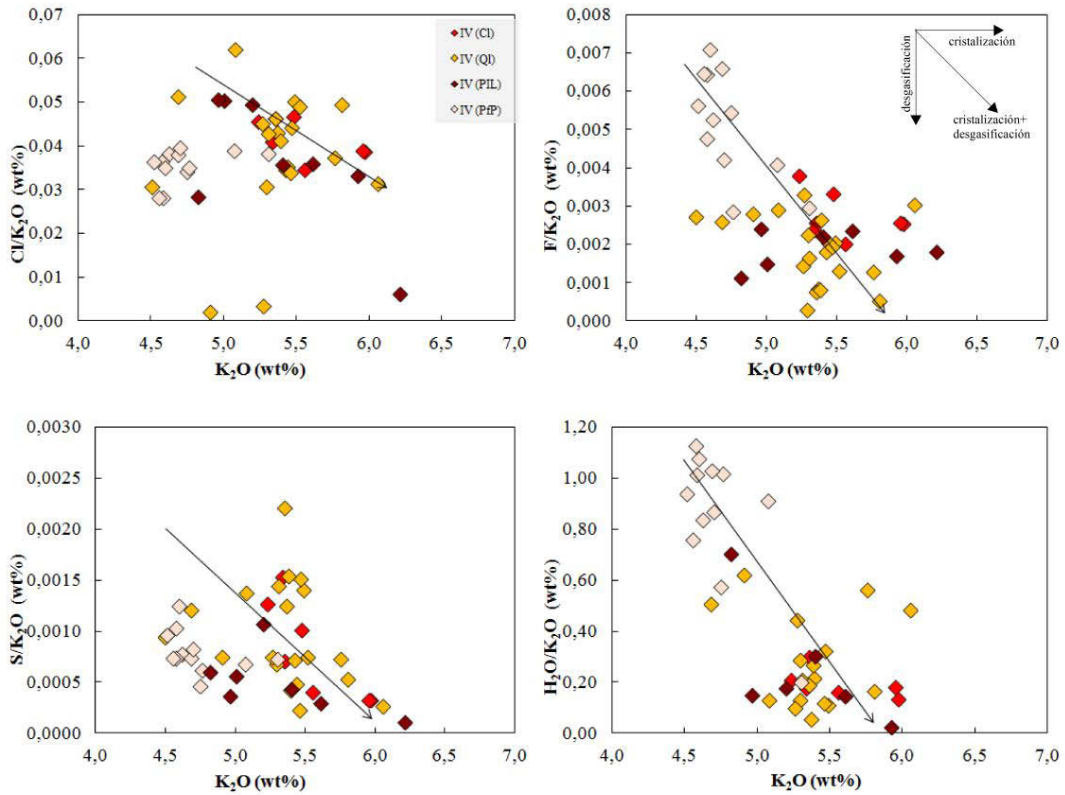
Figura 4.15. Razón volátiles/ K_2O versus el K_2O en inclusiones vítreas del volcán Iruputuncu. El grafico indica si las inclusiones fueron atrapadas en etapas de cristalización, desgasificación o ambas. En general, se observa que las razones de F, Cl, S y H_2O/K_2O disminuye con el aumento del K_2O , indicando desgasificación de estos volátiles durante la cristalización fraccionada.
