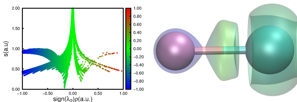
Figure 4: Analyses NCI pour la molécule de FBr. (Gauche) Diagramme de RDG versus \text{sign}(\lambda_2)\rho coloré avec les valeurs de \text{sign}(\lambda_2)\rho . (Droite) RDG=0.5 isosurface coloré avec les valeurs de \text{sign}(\lambda_2)\rho .
