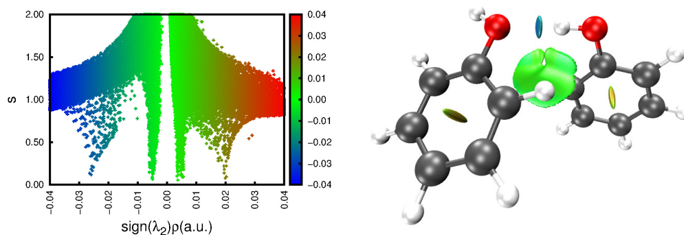
Figure 2: Analyses NCI pour le dimère de phénol. (Gauche) Diagramme de RDG versus \text{sign}(\lambda_2)\rho coloré avec les valeurs de \text{sign}(\lambda_2)\rho . (Droite) RDG=0.5 isosurface coloré avec les valeurs de \text{sign}(\lambda_2)\rho .
