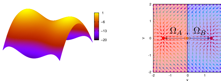
Figure 1: Fonction f(\mathbf{x}, \mathbf{y}) = -x^4 + 4(x^2 - y^2) - 3 (gauche) et la partition induite par son champ de gradient (droite).
