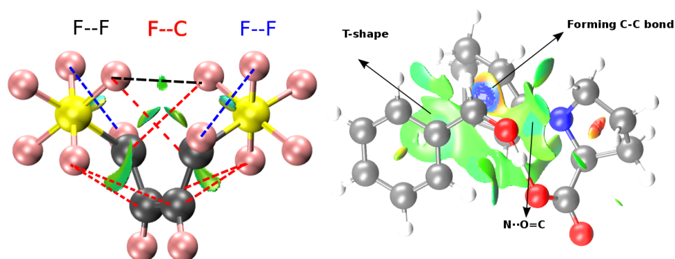
Figure 6: États de transition analyses dans les chapitre 8. (Gauche) État de transition étudié pour analyser l'effet TORQUO avec l'isosurface du RDG à valeur 0.5. (Droite) État de Transition de Houk-List avec l'isosurface du RDG à valeur 0.5.
