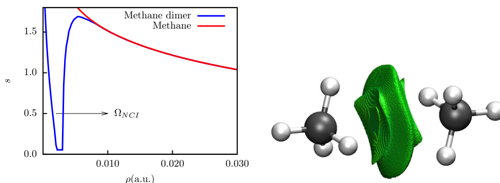
Figure 3: (Left) \Omega_{NCI} pour le dimère de méthane. Dans le diagramme de RDG versus la densité électronique (gauche) et dans la représentation tridimensionnel (droite) \Omega_{NCI} .
