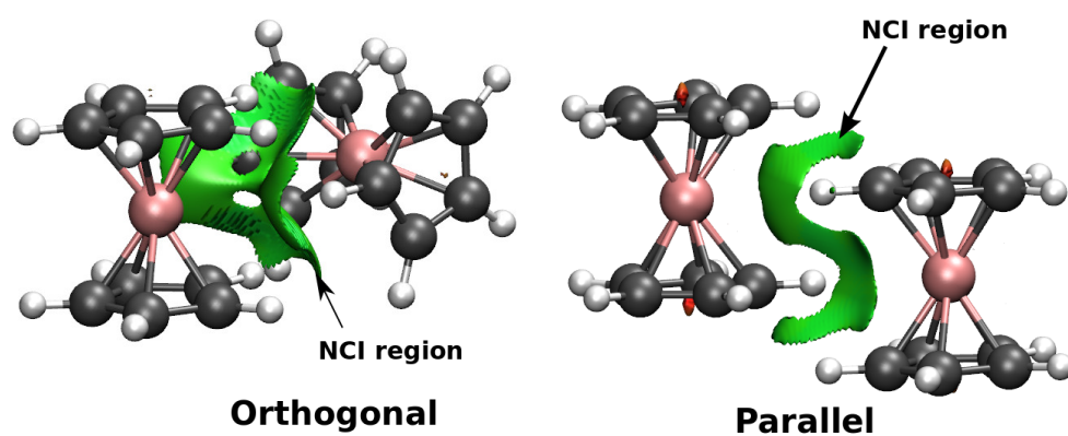
Figure 5: RDG=0.5 isosurfaces pour les dimères de ferrocene en configuration orthogonale (gauche) et parallèle (droite)
