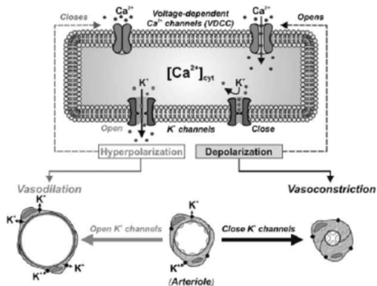
FIGURE 2 [13]: Relaxation de la CML par hyperpolarisation avec ouverture des canaux potassiques calcium-sensible (KCa) et fermeture des canaux calciques voltage dépendants (VOC)
