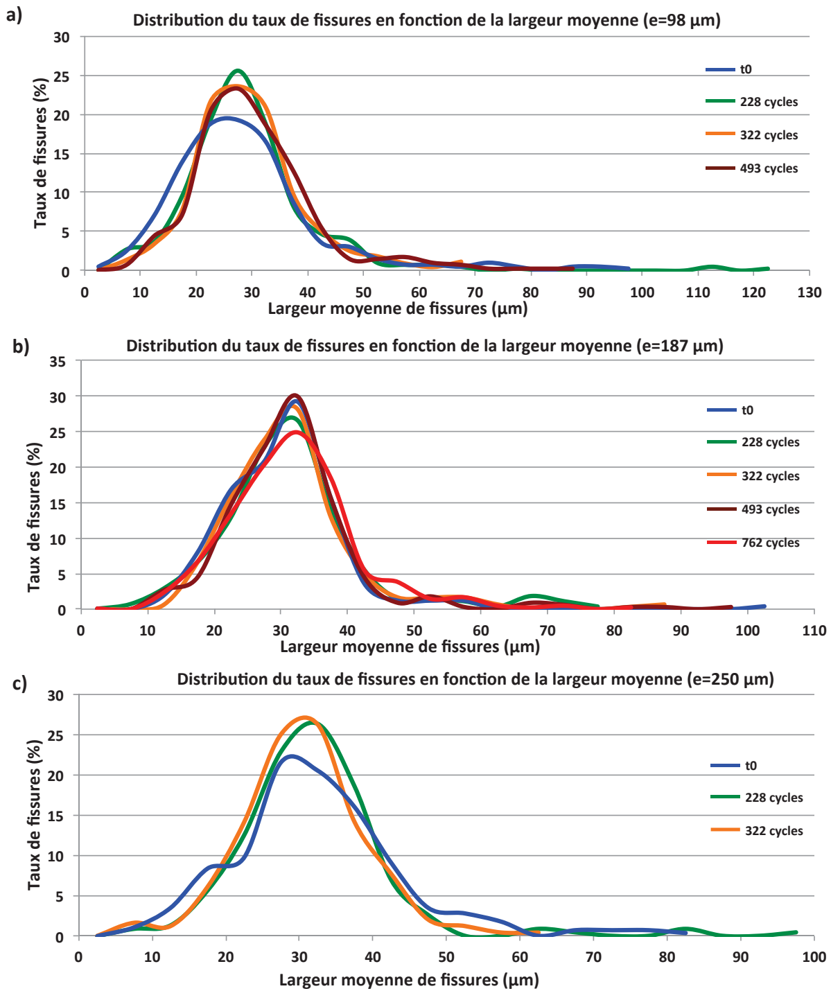
Figure 87 : Evolution du taux de cellules en fonction de la largeur de fissures moyenne pour chaque échantillon en fonction du vieillissement
