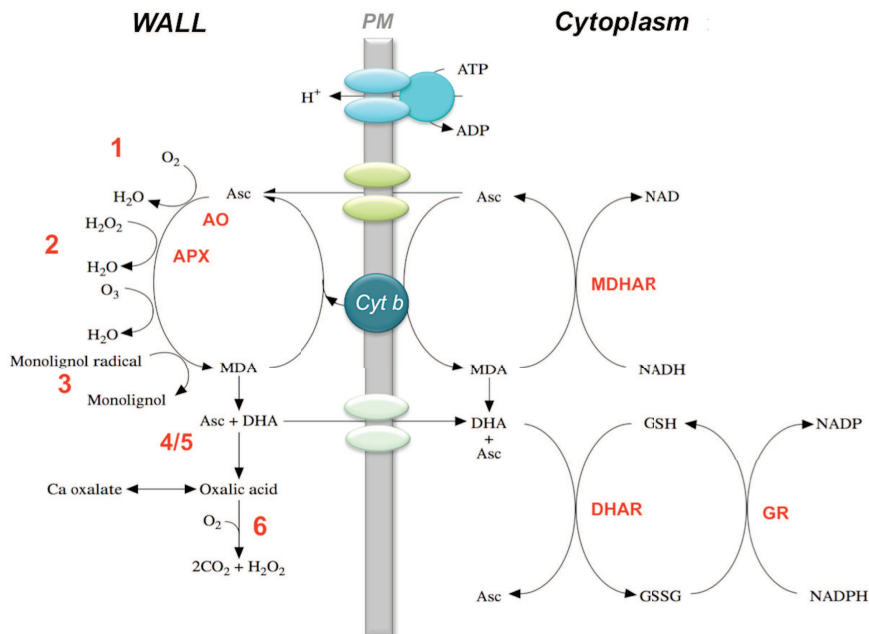
Figure 22: Rôle de l'ascorbate (Asc) dans le cytoplasme et la paroi durant l'expansion cellulaire. (1) L'ascorbate oxydase (AO) catalyse l'oxydation de l'ascorbate en monodéhydroascorbate (MDHA). Le MDHA accepte les électrons provenant du cytochrome b ( Cyt b ) ce qui induit une dépolarisation de la membrane. Cette dépolarisation active une H + -ATPase qui permet le relâchement de la paroi. (2) L'ascorbate peroxydase (APX) en neutralisant le peroxyde d'hydrogène, maintient la plasticité membranaire. (3) L'ascorbate inhibe la réticulation par oxydation des polysaccharides pariétaux mais également la polymérisation de la lignine par piégeage de peroxyde d'hydrogène et des radicaux de monolignol. (4) Le déhydroascorbate (DHA) peut réagir avec les chaînes latérales d'acides aminées des polypeptides pariétaux et ainsi prévenir la réticulation de la matrice de polysaccharide. (5) L'ascorbate et le DHA permettent la formation d'oxalate, lequel est à l'origine du relâchement de la paroi via la fixation de calcium. (6) La dégradation de l'oxalate par l'oxalate oxydase entraîne la production de peroxyde d'hydrogène et de calcium, favorisant ainsi le resserrement de la paroi. (Smirnoff 1996) Abréviations: glutathion réductase (GR); DHA réductase (DHAR); MDA réductase (MDAR)
