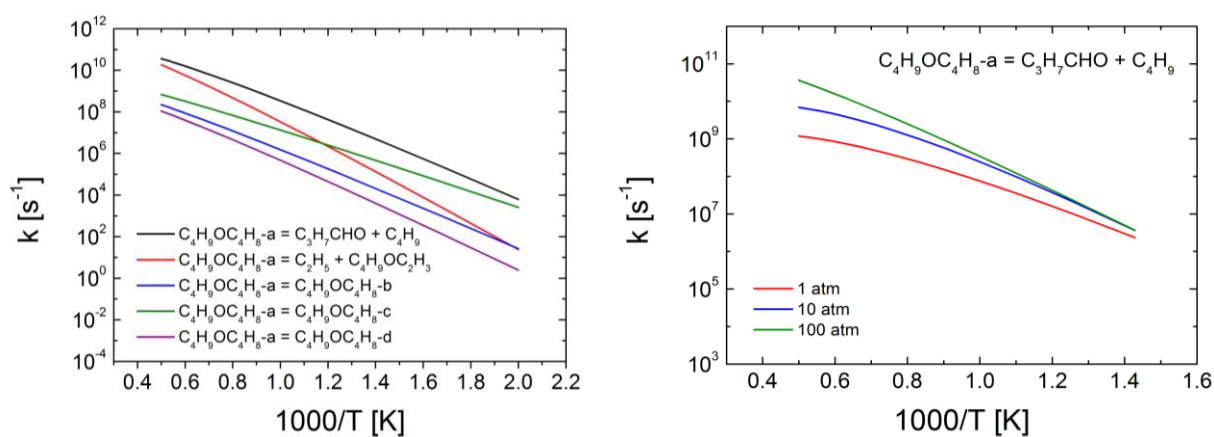
Figure 7.5 : Comparaison des constantes de vitesse haute pression pour les cinq voies de décomposition du radical majoritaire du DBE (gauche). Dépendance en pression de la réaction de consommation majoritaire du radical « a » pour le DBE (droite).
