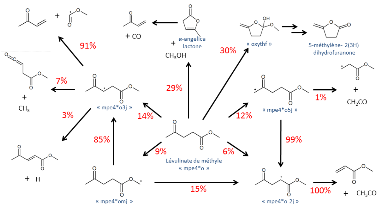
Figure 8.12 : Analyse de voies réactionnelles dans le cas de l'oxydation du lévulinate de méthyle à 1 atm, 1000 K et \phi = 1 .
