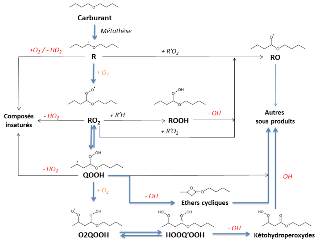
Figure 2.1 : Mécanisme d'oxydation des hydrocarbures en régime de basse température, exemple lié au dibutyl-ether.
