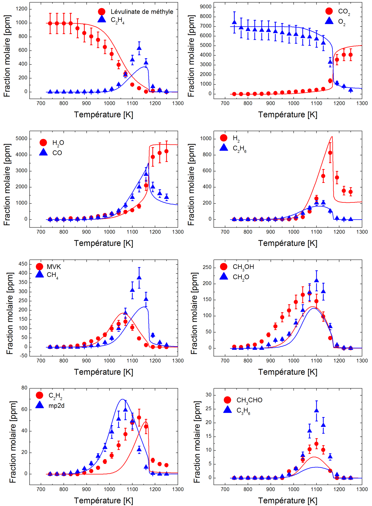
Figure 8.8 : Résultats obtenus à la stoechiométrie ( \phi = 1 ) en réacteur parfaitement agité à 1 atm, \tau = 0,07s et pour 1000 ppm de lévulinate de méthyle. Ligne : ce modèle.
