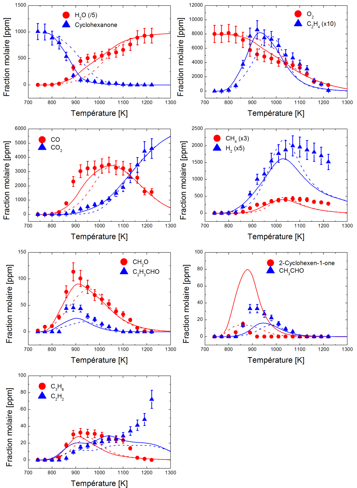
Figure 6.27 : Résultats obtenus à la stœchiométrie en réacteur parfaitement agité à 10 atm, \tau = 0,7s et pour 1000 ppm de cyclohexanone. Traits plein : ce travail. Tirets : Serinyel et al. [93]
