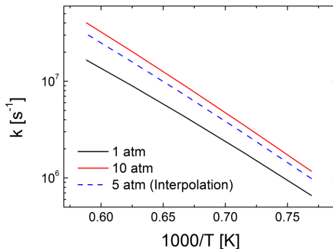
Figure 5.3 : Illustration de l'interpolation réalisée par Chemkin lors de l'utilisation du mot clef « PLOG ». Cas de la réaction \text{CH}_3\text{CHCOCH}_3 = \text{CH}_3 + \text{CH}_3\text{CHCO} .
