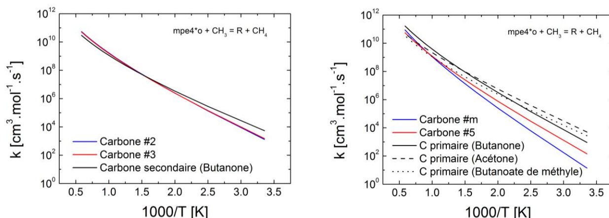
Figure 8.6 : Constantes de vitesse pour les réactions d'arrachement d'hydrogène par le radical méthyle sur le lévulinate de méthyle. Comparaison avec la butanone pour les carbones secondaires (gauche) et avec la butanone, l'acétone [38] et le butanoate de méthyle [213] pour le cas des carbones primaires (droite).
