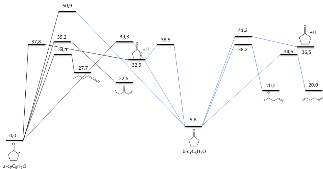
Figure 6.11 : Surface d'énergie potentielle des radicaux de la cyclopentanone (G3//MP2/aug-cc-pVDZ) ( E_0 en \text{kcal.mol}^{-1} )
