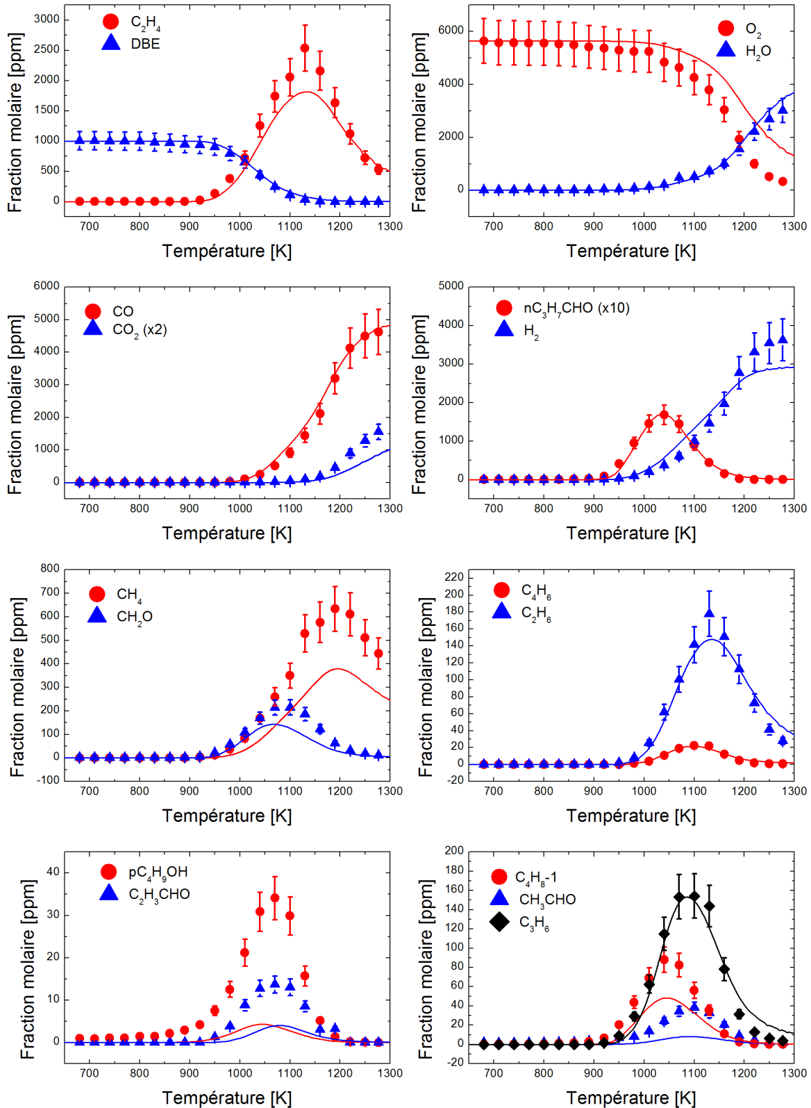
Résultats obtenus en mélange riche ( \phi = 2 ) en réacteur parfaitement agité à 1 atm, \tau = 0,07s et pour 1000 ppm de DBE.
