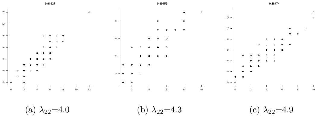
FIGURE 2.1 – 100 observations d’une loi de Poisson bivariée ( p = 1 ) de lois marginales corrélées par \rho_{12} = 0.9
