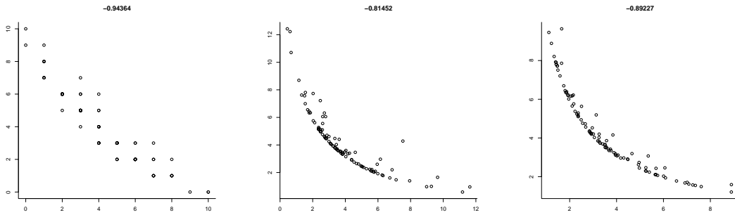
(a) Poisson bivariée ( p = 1 ) (b) Gamma bivariée ( p = 2 ) (c) 1/3-stable bivariée ( p = 5/2 )
