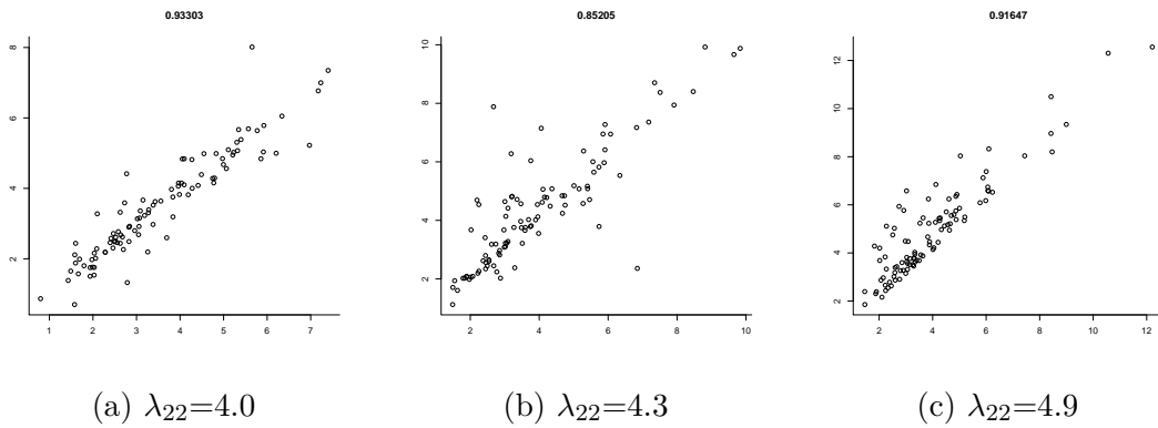
FIGURE 2.3 – 100 observations d’une loi inverse gaussienne bivariée ( p = 3 ) de lois marginales corrélées par \rho_{12} = 0.9
