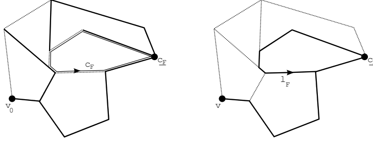
FIGURE 10. Un élément d'une base de lassos
