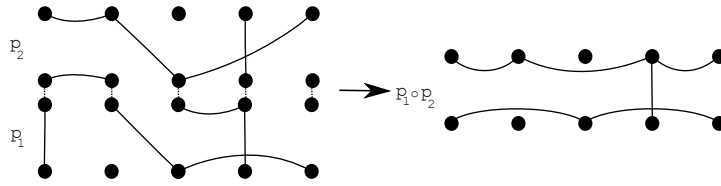
FIGURE 16. Concaténation de deux partitions : p_1 \circ p_2
