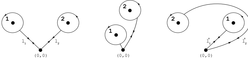
FIGURE 9. Permutation d'un système de particules anyoniques
