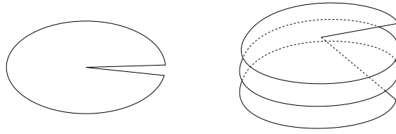
FIGURE 2. Hélice “bouclée” d’ordre trois
