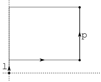
FIGURE 4. Chemin et boucle associée
