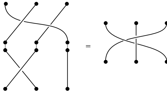
FIGURE 7. Multiplication de deux tresses
