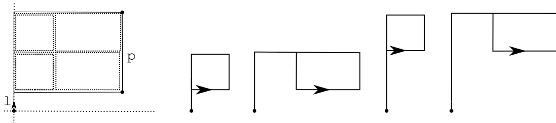
FIGURE 5. Décomposition en L -lassos réguliers
