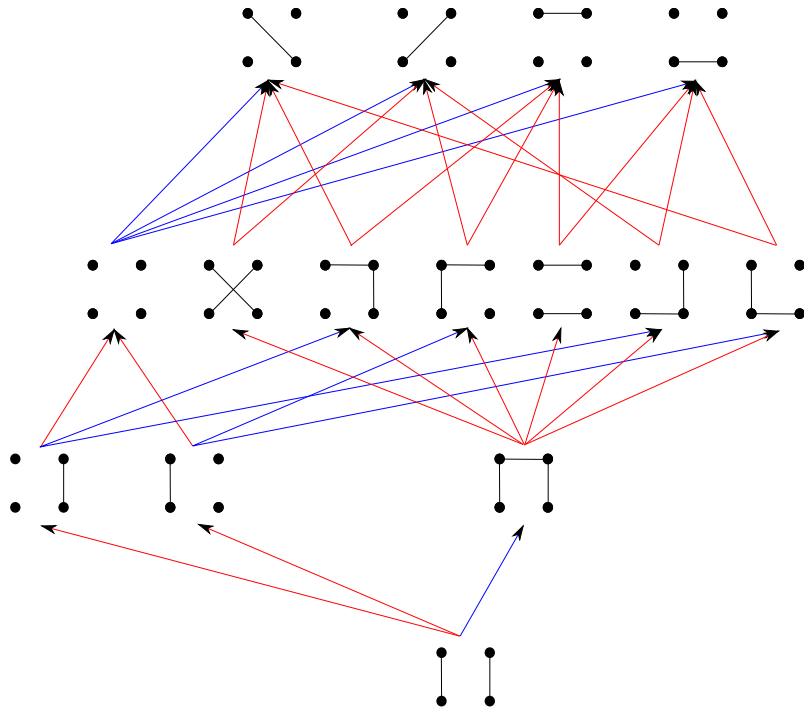
FIGURE 13. Diagramme de Hasse de l'ordre géodésique
