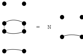
FIGURE 17. Produit faisant intervenir \kappa(p_1, p_2)
