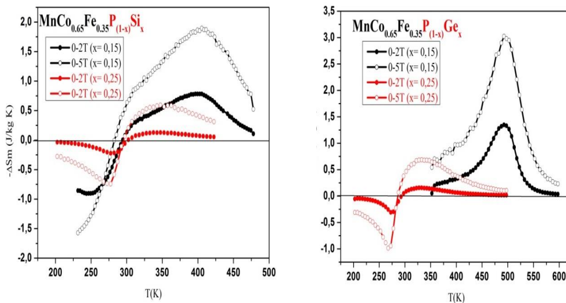
Figure III.54: Dépendance de la variation d'entropie magnétique pour les composés \text{MnFe}_{0.35}\text{Co}_{0.65}\text{P}_{(1-x)}\text{Si}_x et \text{MnFe}_{0.35}\text{Co}_{0.65}\text{P}_{(1-x)}\text{Ge}_x pour des variations de champ 0-2 T et 0-5 T.
