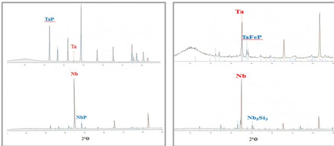
Figure IV.6: DRX de Ta (haut) et Nb (bas) après traitement à 1100°C, du précurseur Fe-P (gauche) et du composé Fe 2 P (droite).
