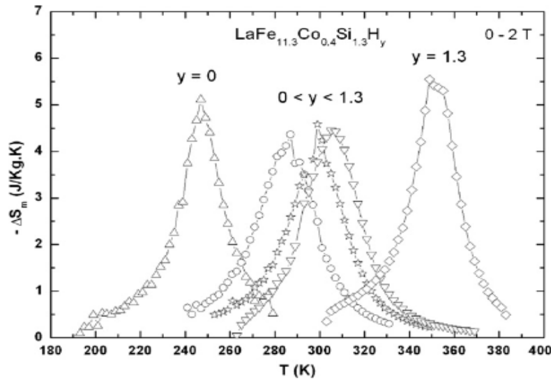
Figure I.11: Variation d'entropie magnétique de composés LaFe_{11.3}Co_{0.4}Si_{1.3}H_y pour une variation de champ 0-2 T [ROS, 10a].
