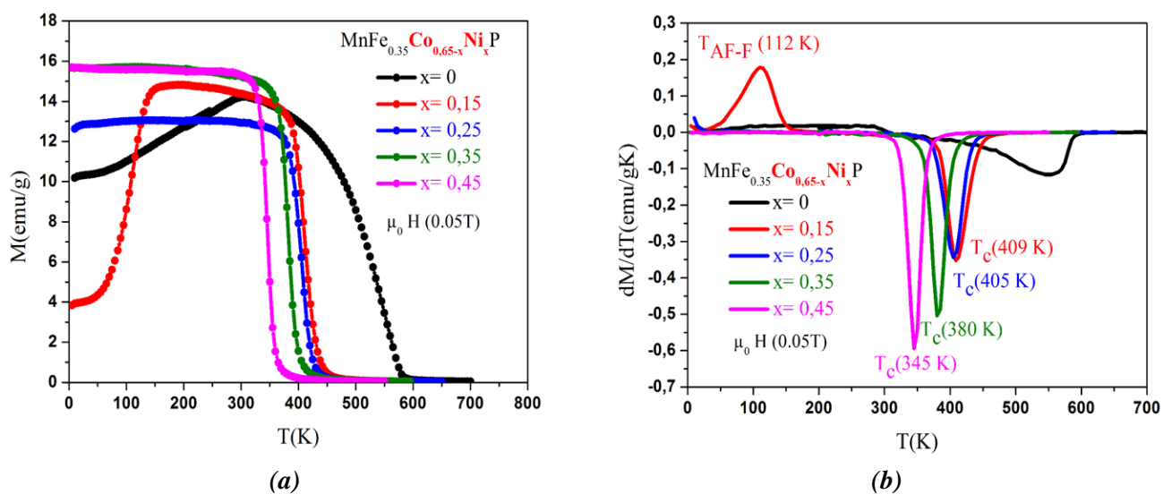
Figure III.26: Dépendance en température de l'aimantation des composés \text{MnFe}_{0.35}\text{Co}_{0.65-x}\text{Ni}_x\text{P} sous un champ constant de 0.05\text{T} (a) et dérivée de l'aimantation par rapport à la température (b).
