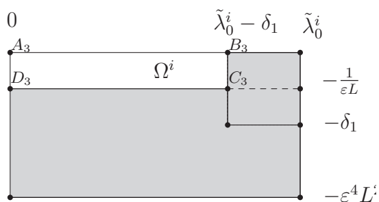
Figure 1.4: Zone ne contenant pas de résonances dans \mathcal{R}^i := [0, \tilde{\lambda}_0^i] - i[0, L^2\varepsilon]
