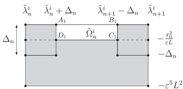
Figure 1.3: Zone ne contenant pas de résonances quand \Delta_n \geq \frac{x_0^2}{\varepsilon L}
