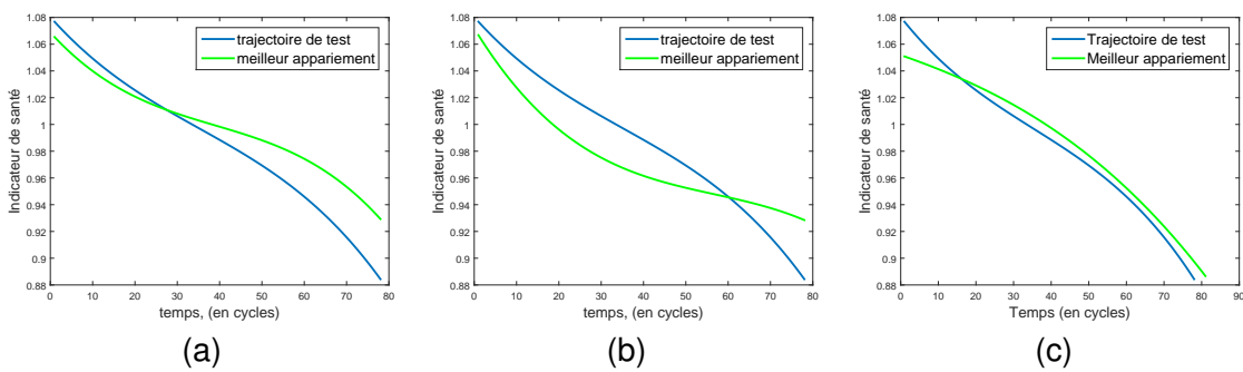
FIGURE 3.20 – Les paires similaires obtenues (a) avec la distance euclidienne, (b) la similarité pondérée et (c) la similarité pondérée avec projection temporelle.
