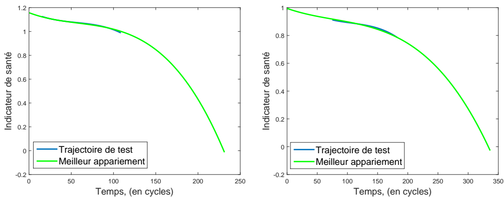
FIGURE 3.21 – Localisation de la trajectoire test sur la trajectoire d'apprentissage la plus similaire.
