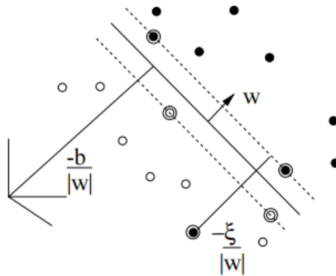
FIGURE 5.5 – Des hyperplans linéaires séparateurs pour le cas non séparable [Burges, 1998].
