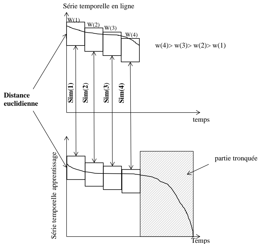
FIGURE 3.13 – Illustration de la similarité pondérée.
