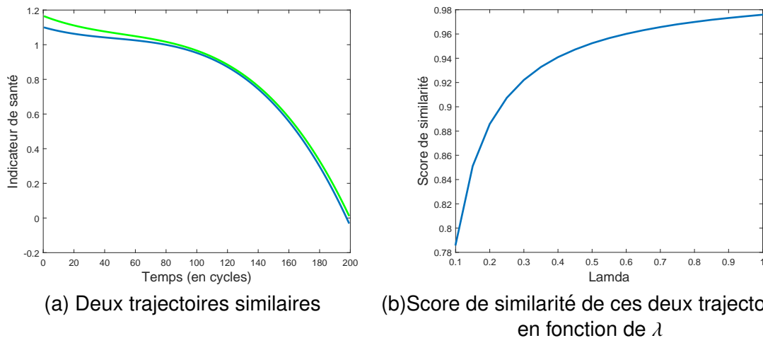
FIGURE 3.15 – Influence de \lambda sur le score de la similarité.
