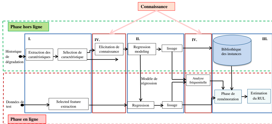
FIGURE 2.12 – Le schéma général de l'approche globale proposée.
