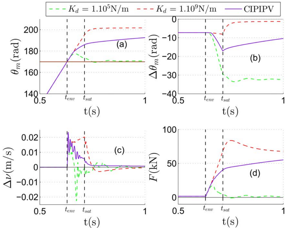
FIGURE 6.14 – Résultats obtenus pour le test avec un CIIPV sur un intervalle temporel restreint avec (a) le suivi de trajectoire de \theta_m , en (b) l’erreur de position \Delta\theta = \theta_d - \theta_m , en (c) \Delta\nu et en (d) l’énergie mécanique perdue dans la transmission.
