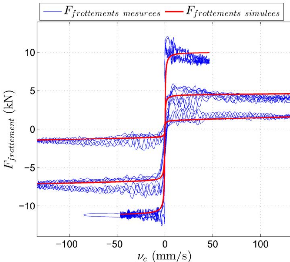
FIGURE 2.13 – Comparaison entre les forces de frottement réelles et simulées grâce au modèle présenté précédemment pour F_a = 0 \text{ kN} , F_a = 20 \text{ kN} et F_a = 35 \text{ kN} .
