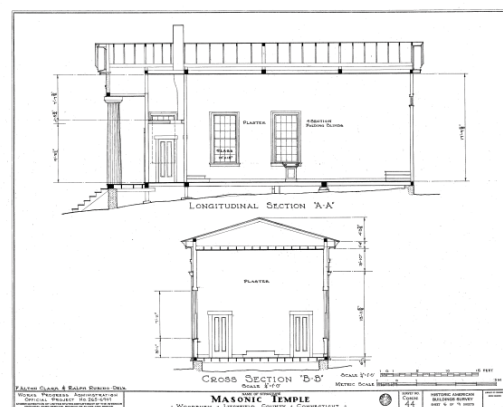
Fig. 59 et 60 : Temple maçonnique de Woodbury, Connecticut. Architecte inconnu, 1838. Plans et coupes.
