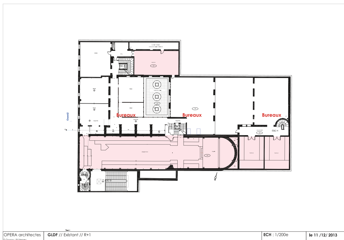
Fig. 75 & fig. 76 : Siège de la Grande Loge de France à Paris – Plan du rez-de-chaussée et du 1 er étage, avant les travaux de 2014. En rose, emplacement des temples. Le bâtiment en comporte 20 en tout, dont le « Grand Temple » au 1 er étage ; ci-dessus. Source : OPERA Architectes
