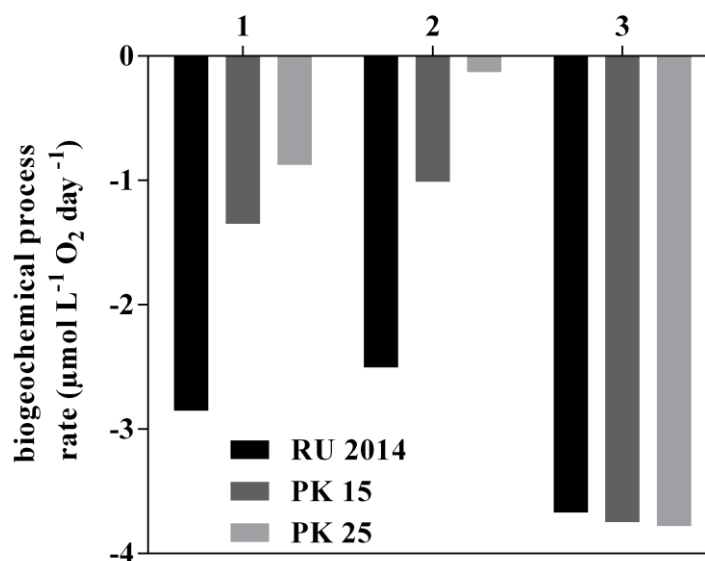
Figure IV.27 : Moyennes estivales des flux biogéochimiques consommateurs d'oxygène dans la zone de Bordeaux pour les scénarii d'augmentation de la température : 1-nitrification, 2-minéralisation du CO provenant des rejets urbains, 3-minéralisation du CO provenant du bassin versant (COP litière + COD fluvial).
