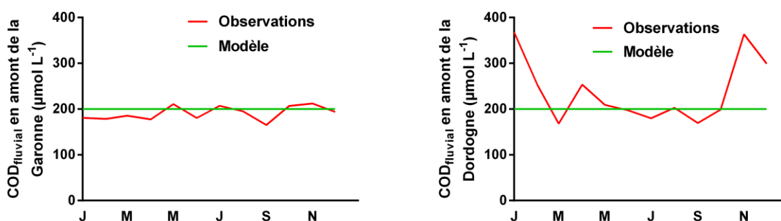
Figure II.8 : Moyenne mensuelle du \text{COD}_{\text{fluvial}} en amont de la Garonne (gauche) et de la Dordogne (droite). Les observations sont en rouge (Veyssy, 1998a) et les valeurs insérées dans le modèle sont en vert.
