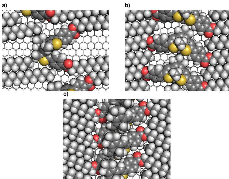
FIGURE 5 – Modèles de couches auto-assemblées générées par les formes a) ouvertes, b) fermées, et c) sous-produit du diaryléthène photoswitcher.
