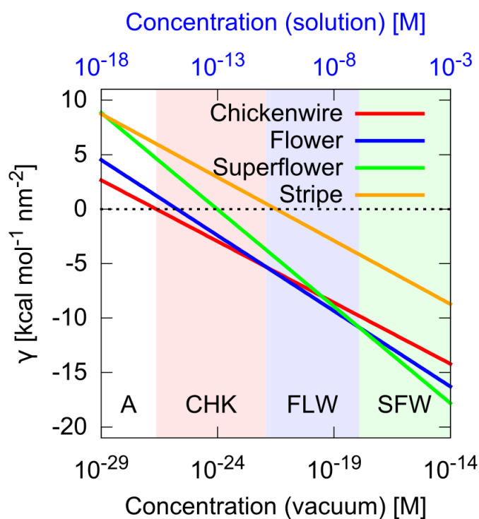
FIGURE 2 – Énergie libre de surface en fonction de la concentration de monomères pour l'auto-assemblage de l'acide trimésique (TMA) dans les trois architectures observées expérimentalement - chickenwire (CHK), fleur (FLW), et superfleur (SFW) - et l'architecture hypothétique stripe (STR). La dépendance à la concentration est évidente, montrant comment, à faible concentration, l'état monomère A est favorisé, alors que à concentration plus élevée les trois auto-assemblages CHK, FLW, et SFW sont visibles dans cet ordre. La valeur de \gamma pour l'architecture STR est, à toutes les concentrations, plus élevée que celle des autres. Cela signifie que cet architecture n'est jamais visible à l'équilibre thermodynamique.
