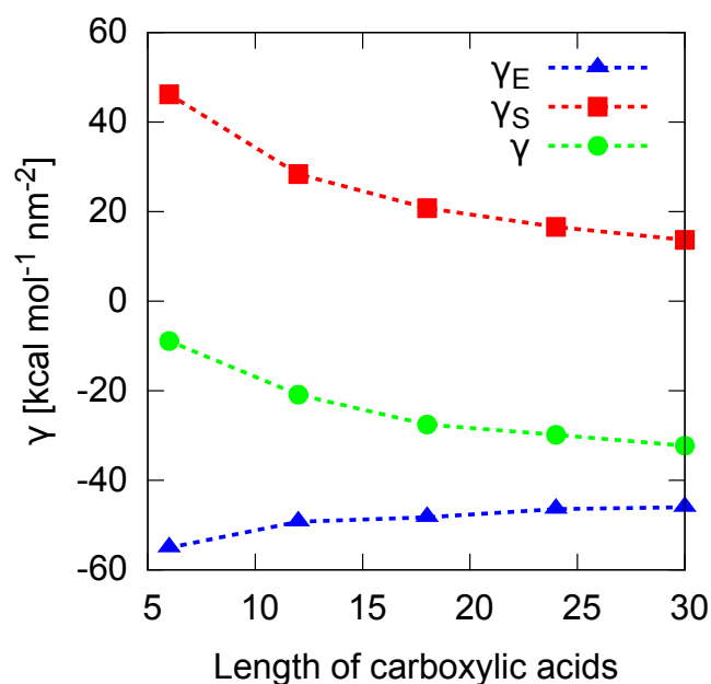
FIGURE 4 – Différences d'énergie (bleu), entropie (rouge) et d'énergie libre (vert) normalisées par la surface pour l'auto-assemblage des molécules étudiées en fonction de la longueur de la chaîne.
