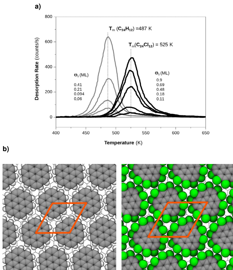
FIGURE 6 – a) Données obtenues par désorption à température programmée (TPD) pour le coronène et le coronène perchloriné. L'augmentation de la température de désorption après perchloration est clairement visible. b) monocouches auto-assemblées modélisées pour le coronène et le perchlorocoronène. Les deux s'assemblent en un réseau hexagonal, la seconde avec une maille élémentaire 30% plus grande que la première.
