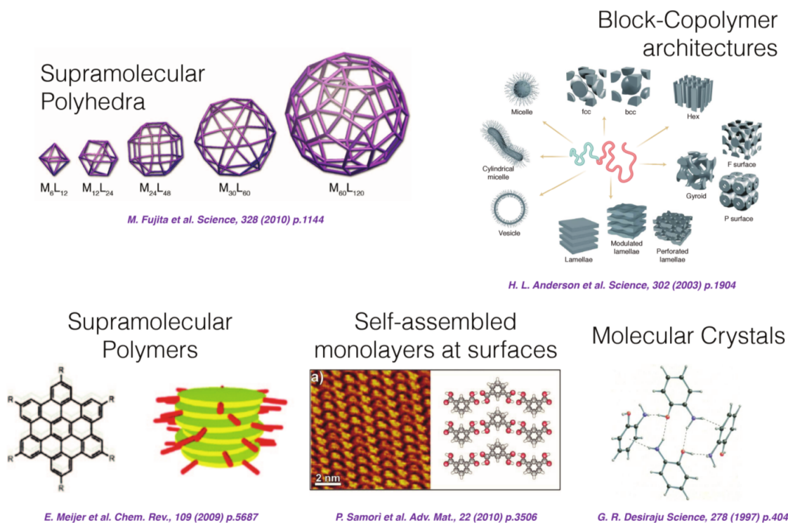
FIGURE 1 – Exemples d’auto-assemblage moléculaire de taille fini et infini.
