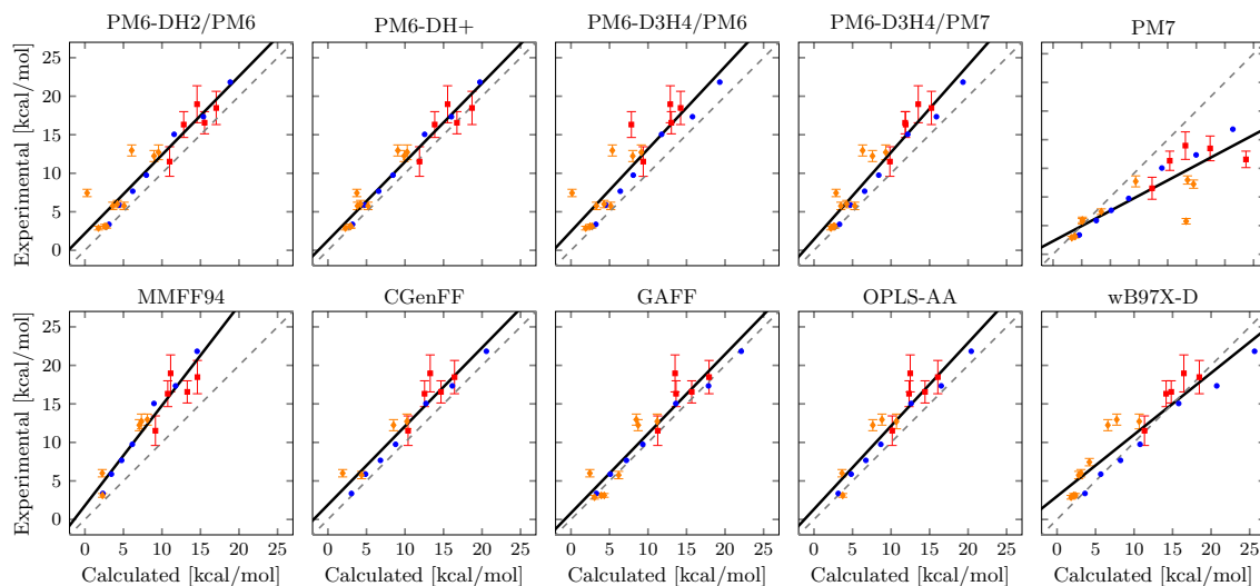
FIGURE 3 – Graphes de corrélation entre les énergies de désorption expérimentales et calculées pour cinq méthodes semi-empiriques (PM6-DH2/PM6, PM6-DH+, PM6-D3H4/PM6, PM6-D3H4/PM7 et PM7), quatre champs de force classiques (MMFF94, CGenFF, GAFF et OPLS-AA) et une méthode DFT ( \omega B97XD/6-31G(d)). L’ajustement idéal est représenté par la ligne en pointillé gris, ce qui correspond à une égalité parfaite entre les énergies de désorption calculées et expérimentales. L’ajustement obtenu est la ligne noire solide. Les barres d’erreur correspondent à l’incertitude dans la détermination expérimentale de l’énergie de désorption.
