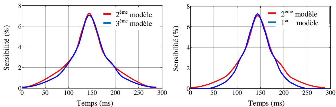
Figure VI.23: Signature d'un véhicule traversant une boucle circulaire
