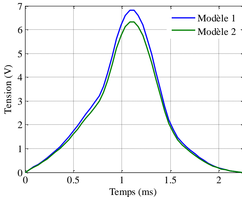
Figure VII.16: Exemple d'un signal de tension généré par un câble piézo-électrique, soumis à une force ( m = 560 \text{ kg} )
