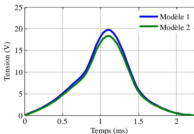
Figure VIII.3: Choc piézoélectrique produit par un PL (vitesse 80 km/h)
