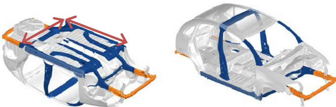
Figure VI.1: Partie du châssis considérée dans l'étude
