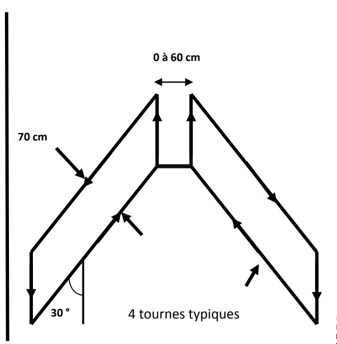
Figure V.12: Boucle électromagnétique en forme chevron
