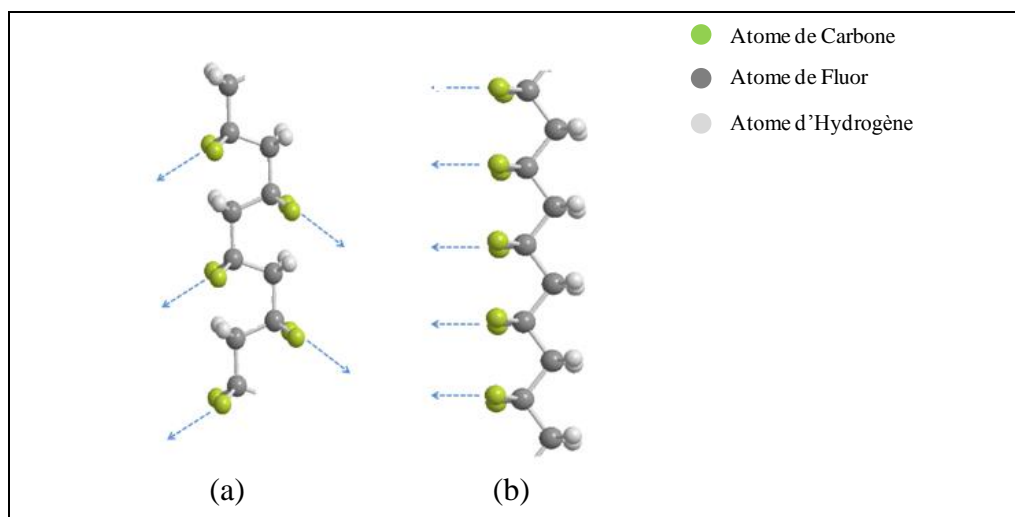
Figure VII.4: Structure d'un polymère (a) conformation non polarisée, (b) conformation polarisée [57]
