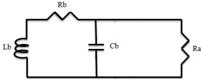
Figure 0.4: Circuit équivalent de l'oscillateur quasi-sinusoidal
