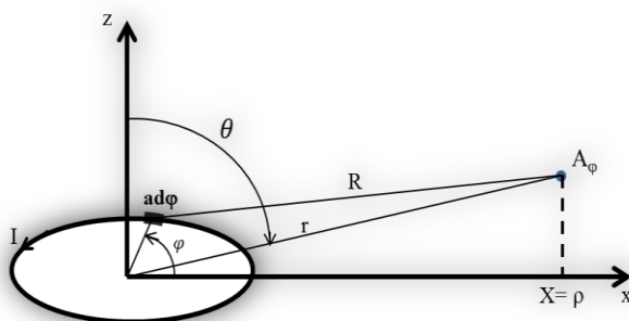
Figure VI.17: Boucle électromagnétique circulaire
