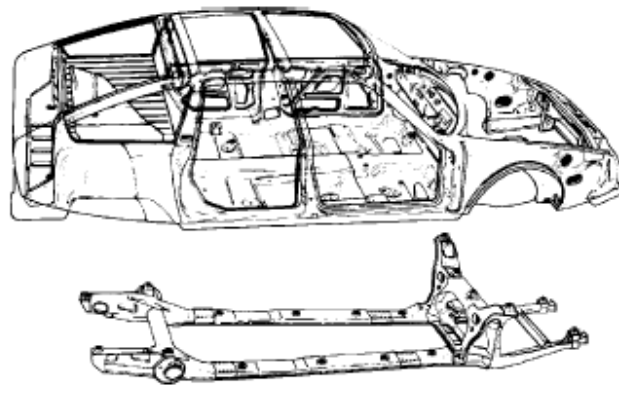
Figure V.7: Châssis caisson [28]
