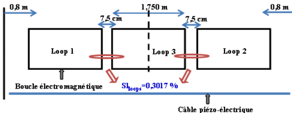
Figure VIII.7: Configuration optimisée du capteur hybride
