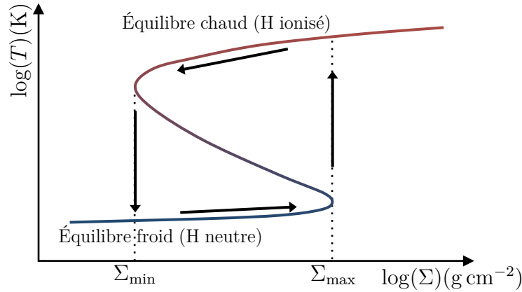
Figure 2.3 – Relation entre la température T et la densité surfacique \Sigma pour un anneau de disque d'accrétion. Deux branches d'équilibre stable « froide » et « chaude » existent. Le passage de l'une à l'autre se fait de façon hystérétique du fait de l'instabilité thermo-visqueuse. La branche instable (au milieu) se situe aux alentours de la température d'ionisation de l'hydrogène ( \sim 5000 K). Figure inspirée de Latter & Papaloizou (2012) .
