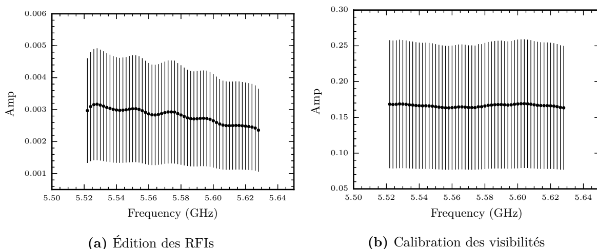
Figure 7.8 – Figures similaires à celle présentée en fig. 7.6b, illustrant l’amplitude des visibilitées en fonction de la fréquence pour la fenêtre spectrale SW 6 du VLA lors de l’observation de GRS 1739–278. Le signal de radar périodique a été éliminé en fig. 7.8a (comparativement à la fig. 7.6b). Les données ont été ensuite calibrées en fig. 7.8b. Entre autres (§7.3.2), la réponse du récepteur a été prise en compte et le signal a visiblement été lissé.
