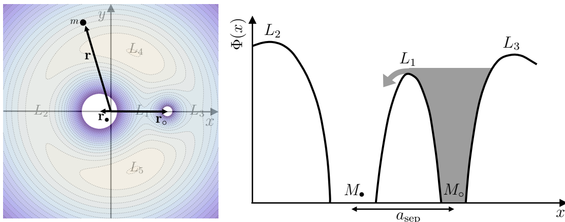
Figure 1.4 – Gauche : potentiel de Roche exercé par un système binaire composé d'un trou noir de masse M_{\bullet} et d'une étoile de masse M_{\circ} tel que M_{\bullet} = 5M_{\circ} . L'origine du repère correspond au centre de masse du système. Les points de Lagrange L_n y sont représentés. Crédits : Ileyk El Mellah 4 . Droite : potentiel de Roche selon une coupe dans l'axe des points L_1 , L_2 et L_3 . Le transfert de masse de l'étoile vers l'objet compact est illustré.
