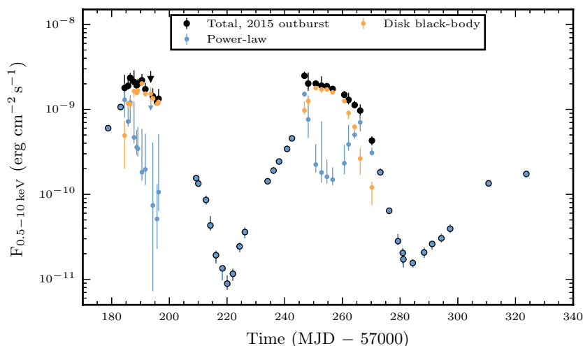
Figure 12.7 – Évolution du flux 0.5–10 keV en 2015, associé aux composantes loi de puissance (points bleus) et corps noir multi-températures du disque d'accrétion (points orange). La somme de ces deux composantes est représentée par les points noirs.
