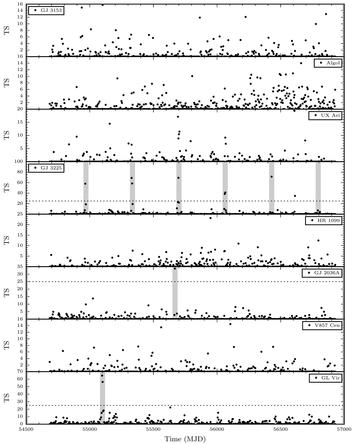
Figure 9.11 – Évolution de la significativité \gamma moyennée sur 4 jours à partir d'un modèle d'émission de la région fixe pour différents systèmes de type RS CVn/Algol sélectionnés. Le graphe de GJ 3225 contient un point non représenté ici : pour MJD 56424, le TS atteint \sim 2432 à cause d'une éruption solaire proche.
