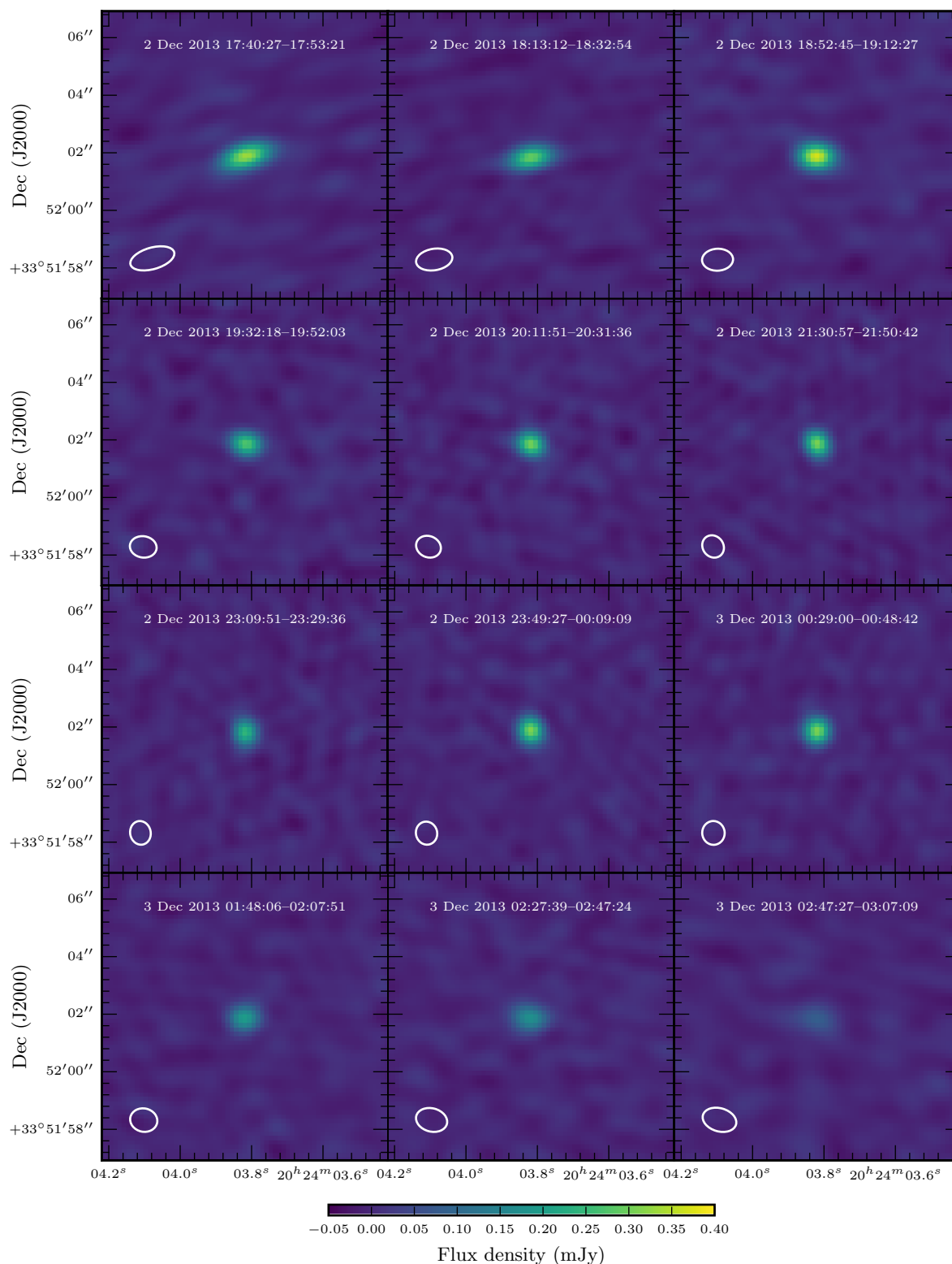
Figure 11.1 – Échantillon d’images de V404 Cyg avec le VLA au cours de l’observation. Chaque image est moyennée sur deux scans consécutifs dans la bande 6.94–7.96 GHz. L’évolution de la forme de la PSF synthétisée traduit la variation de l’élévation au cours du programme. Une variabilité significative est visible à l’œil nu.
