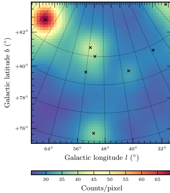
Figure 9.3 – Carte de l'émission \gamma intégrée sur les sept années de données du LAT analysées. La région, proche du pôle Nord Galactique ne présente qu'une faible densité de sources Fermi (repérées par les croix noires) et une émission diffuse très modérée.
