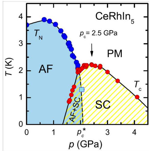
Figure 1 Diagramme de phase typique d'un fermion lourd, représenté par \text{CeRhIn}_5 [108]. AF, PM et SC sont les états antiferromagnétique, paramagnétique et supraconducteur respectivement. T_N et T_c sont les températures de Néel et supraconductrice respectivement. p_c and p_c^* sont les pressions critiques, correspondant au maximum de T_c et à la pression à laquelle T_N \rightarrow 0\text{K} respectivement.
