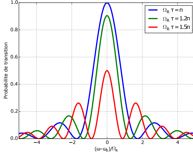
FIGURE I.2 – Probabilité de transition - Méthode de Rabi
