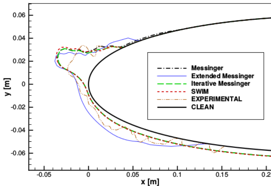
Figure 3.13 Comparaison des formes de givre obtenues entre les modèles de Messenger, Messenger Itératif, SWIM et Extended Messenger à T = 269.10K , LWC = 1.3g/m^3 , d = 20\mu m , A0A = 4^\circ , U_\infty = 58m/s , t = 480s [Lavoie et al., 2016]
