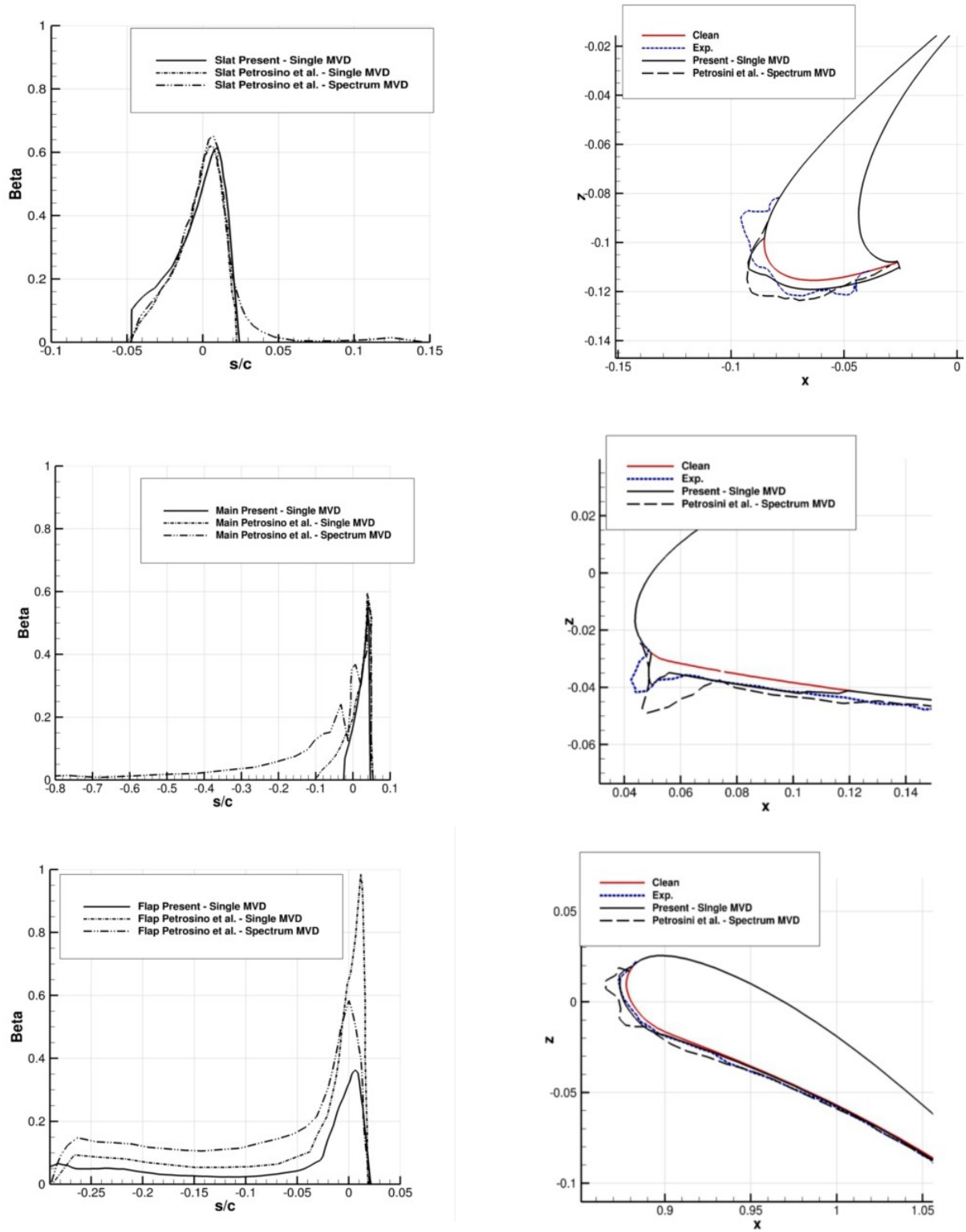
Figure 7.35 Comparisons de l'efficacité de collection et du givrage avec [Petrosino et al., 2011] et les résultats expérimentaux du NASA Glenn Research Center [Kind et al., 2001].
