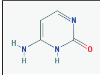
Cytosine
