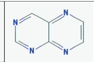
Ptéridine
