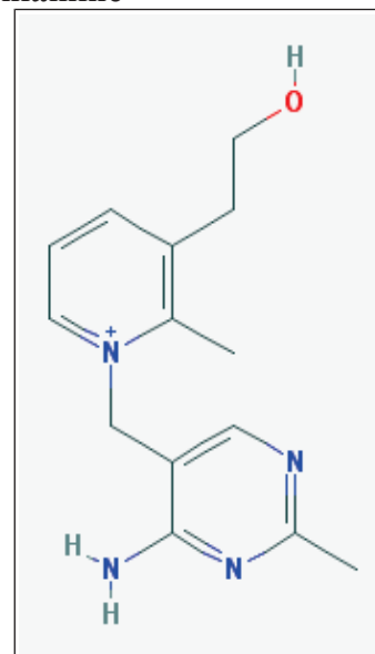
Pyriothiamine
