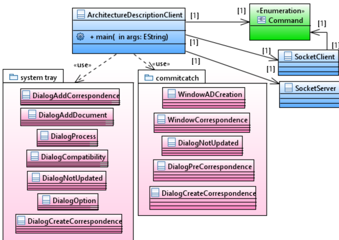
FIGURE 5-4 DIAGRAMME DE CLASSE SIMPLIFIÉ DE LA PARTIE CLIENT D'APPE
