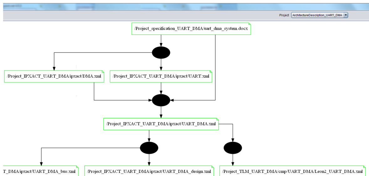
FIGURE 6-8 APPE : GÉNÉRATION DU PROCESSUS (EXTRAIT)
