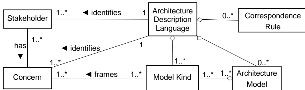
FIGURE 3-7 LANGAGE DE DESCRIPTION D'ARCHITECTURE DANS LE STANDARD 42010
