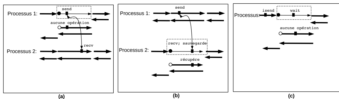
FIGURE 2: Trois exemples dans lesquels nous appliquons du receive-logging. Pour plus de clarté, nous avons séparé les processus: processus 1 en haut et processus 2 en bas. (a) Un programme adjoint après le checkpointing d’un morceau de code ne contenant que la partie send d’une communication point à point. (b) Un programme adjoint après le checkpointing d’un morceau de code ne contenant que la partie recv d’une communication point à point. (c) Un programme adjoint après le checkpointing d’un morceau de code contenant seulement la partie wait d’une communication non bloquante.
