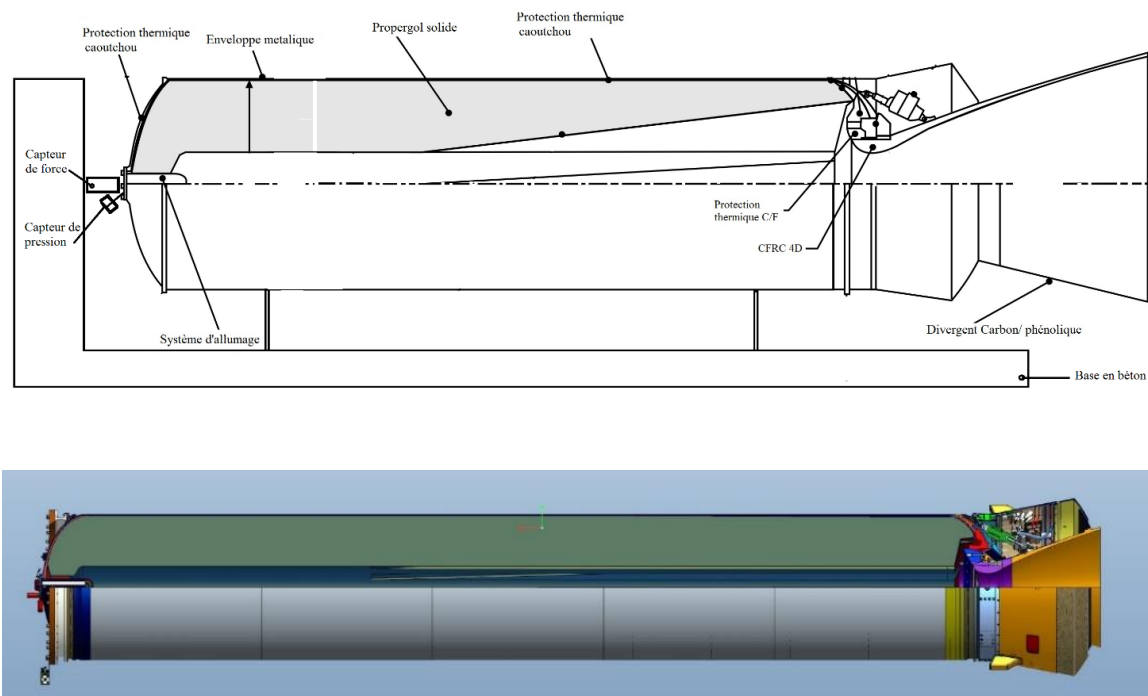
Figure 2.15 – Dimensionnement et illustration du moteur S43.
