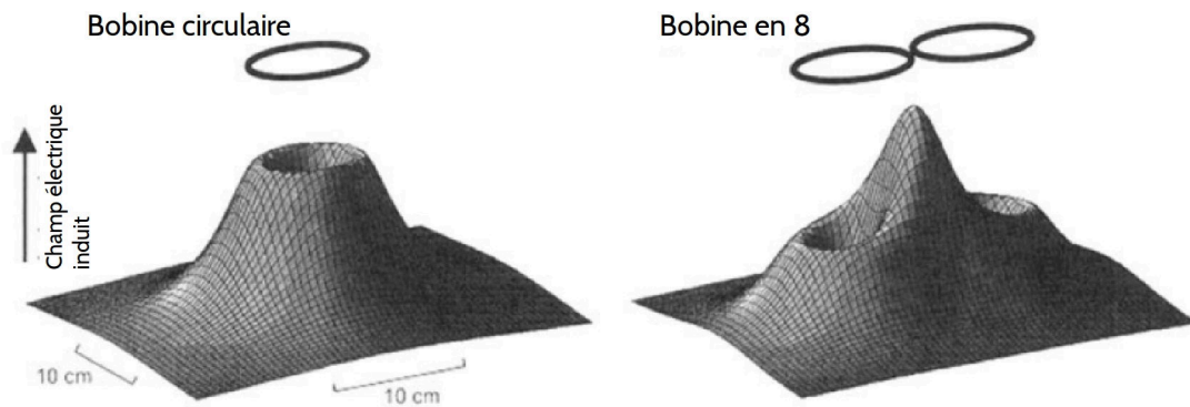
FIGURE 3.4 – Distribution spatiale du champ électrique induit pour une bobine circulaire et en huit, sur une surface plane homogène, d’après Ilmoniemi et al. (1999).
