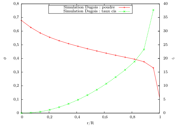
Figure 3.9 – Superposition des profils de répartition de poudre et de taux de cisaillement en sortie de canal. Résultats obtenus pour une suspension initialement homogène en poudre à \phi_0^s = 0,45 dans la configuration a/R = 0,0256 .
