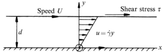
Figure 1.7 – Cisaillement simple. Écoulement d'un fluide newtonien entre une plaque immobile (bas) et une plaque mobile (haut) à vitesse U séparées d'une distance d . \dot{\gamma} = U/d . [Tanner, 1985].
