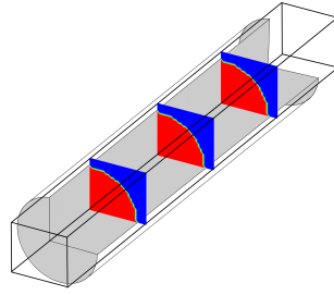
Figure 3.3 – Domaine de simulation représentatif du montage expérimental des travaux de Hampton. La boîte noire représente le domaine d'étude numérique. En bleu, la zone imperméable et pénalisée (extérieur de la conduite). En rouge, la partie fluide (intérieur de la conduite).
