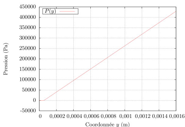
Figure 3.15 – Champs de pression selon y dans un milieu poreux de référence de perméabilité K_b en écoulement établi. La perte de charge observée numériquement est de \Delta p_b = 4,2916 \cdot 10^5 Pa.
