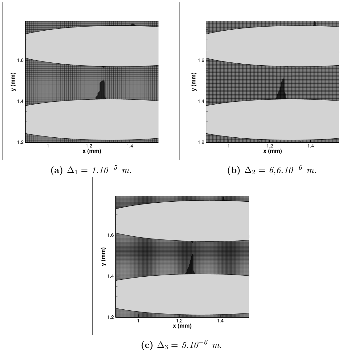
Figure 4.22 – Exemple d'une inhomogénéité résolue par le modèle développé dans ces travaux. Comparaison des résultats obtenus sur trois maillages de plus en plus fins.
