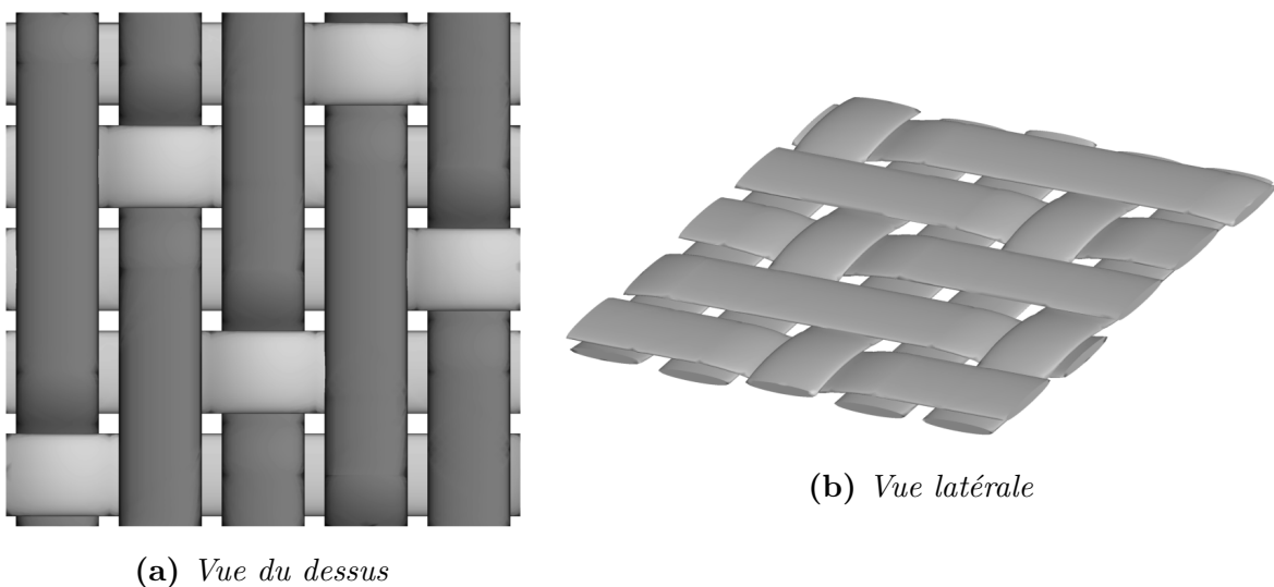
Figure 4.24 – Conception assistée par ordinateur d'une armure de satin de module 5 et de décochement 3.
