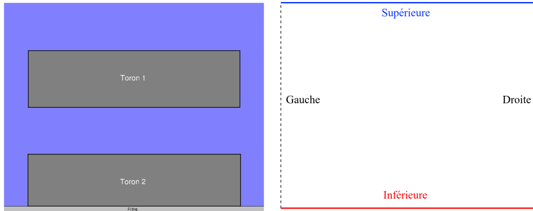
Figure 4.4 – Représentation du domaine de calcul pour l'étude paramétrique ( gauche ) et noms des limites du domaine ( droite ).
