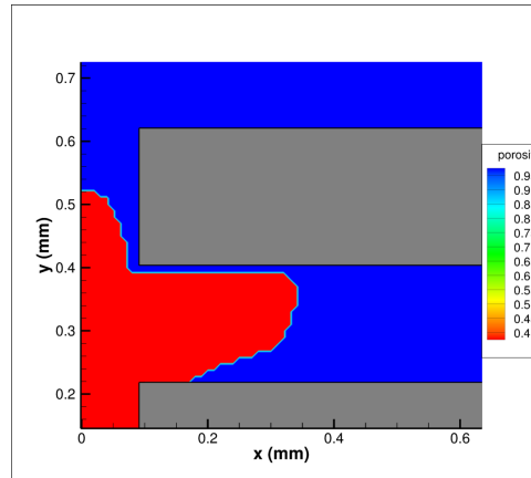
Figure 4.7 – Veine de 3 mailles d'épaisseur entre le gâteau particulaire et le toron supérieur à t = 3,96 \text{ s}
