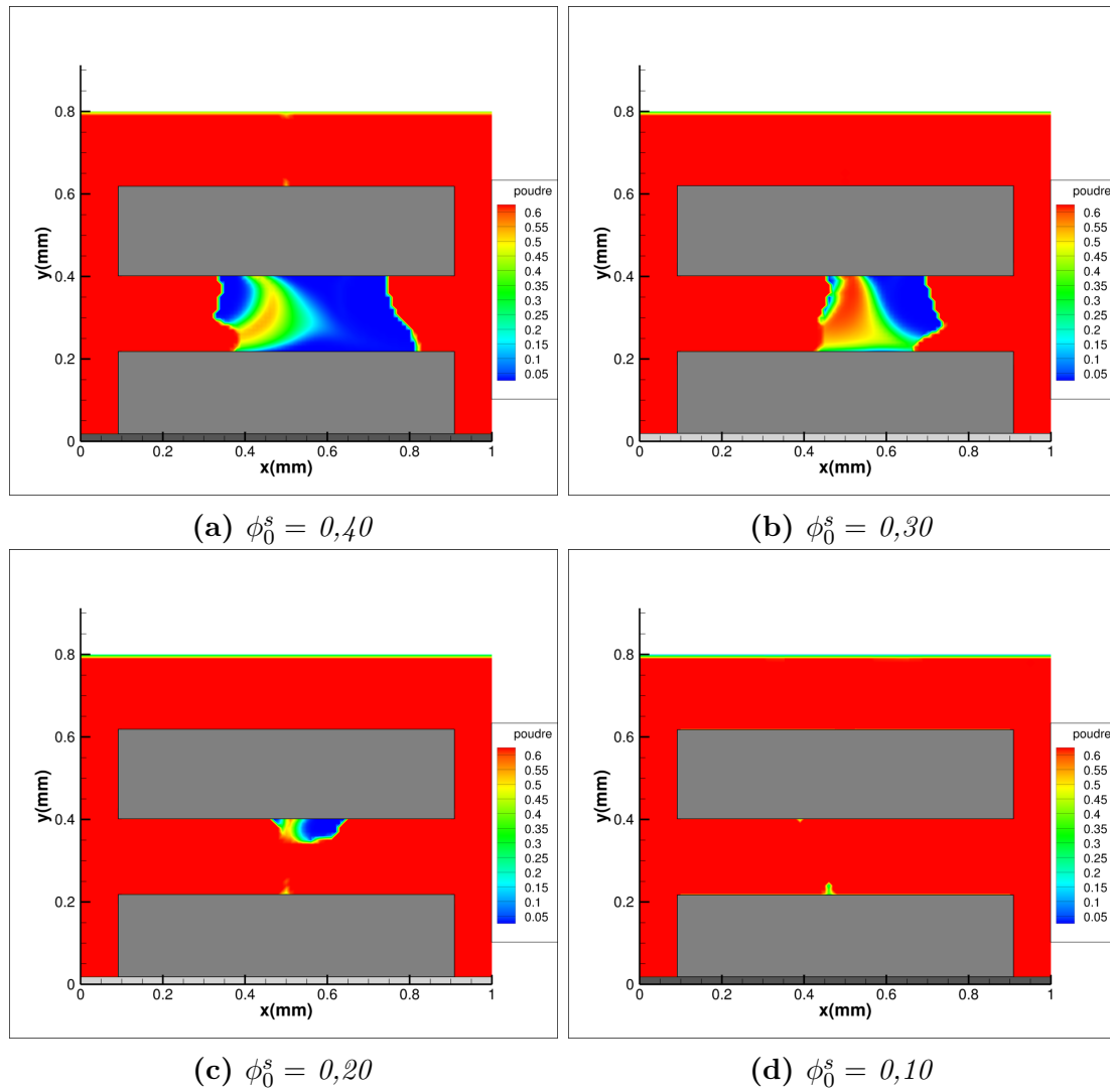
Figure 4.11 – Champs finaux de fraction volumique de poudre et taille de la macroporosité obtenue pour quatre suspensions différemment chargées en particules.
