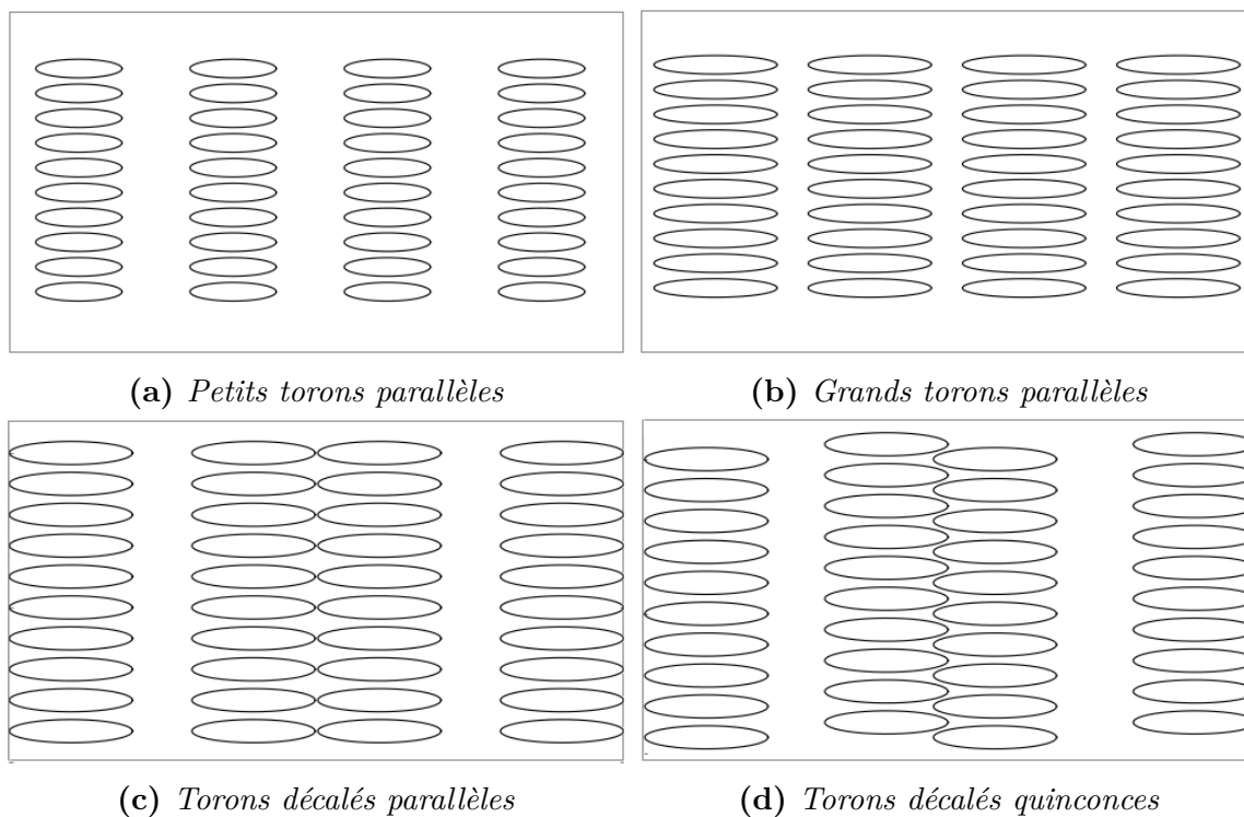
Figure 4.2 – Exemples de configurations géométriques de torons, rencontrées dans la pré-forme fibreuse utilisée dans ces travaux. Vue selon une coupe 2D.
