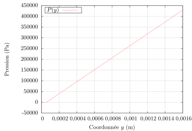
Figure 3.15 – Champs de pression selon y dans un milieu poreux de référence de perméabilité K_b en écoulement établi. La perte de charge observée numériquement est de \Delta p_b = 4,2916 \cdot 10^5 \text{ Pa} .
