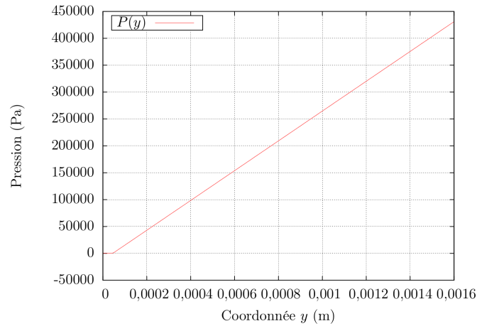
Figure 3.17 – Champs de pression selon y dans le gâteau particulaire en écoulement établi. La perte de charge observée est de \Delta p = 4,2916 \cdot 10^5 Pa.
