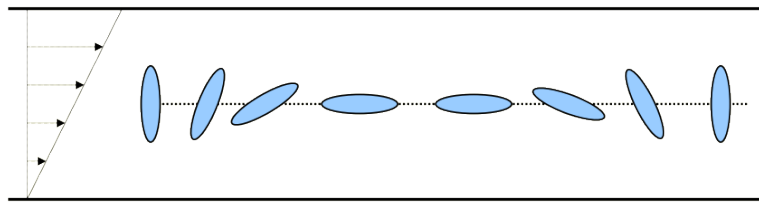
Figure 1.12 – Modification de l'orientation d'une particule aplatie ( F > 1 ) dans un écoulement à cisaillement simple.
