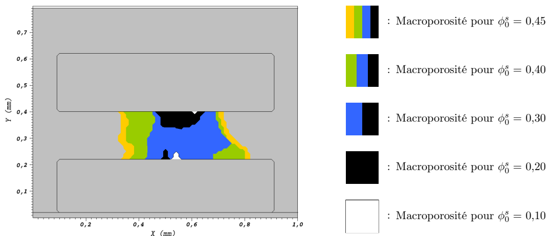
Figure 4.12 – Superposition de la taille moyenne de la macroporosité obtenue pour les cinq suspensions initiales (0,10; 0,20; 0,30; 0,40 & 0,45). Plus la concentration initiale en particules est faible, plus la macroporosité est petite.
