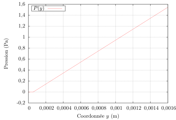
Figure 3.14 – Champs de pression selon y dans un milieu poreux de référence de perméabilité K_a en écoulement établi. La perte de charge observée numériquement est de \Delta p_a = 1,545 \text{ Pa} .
