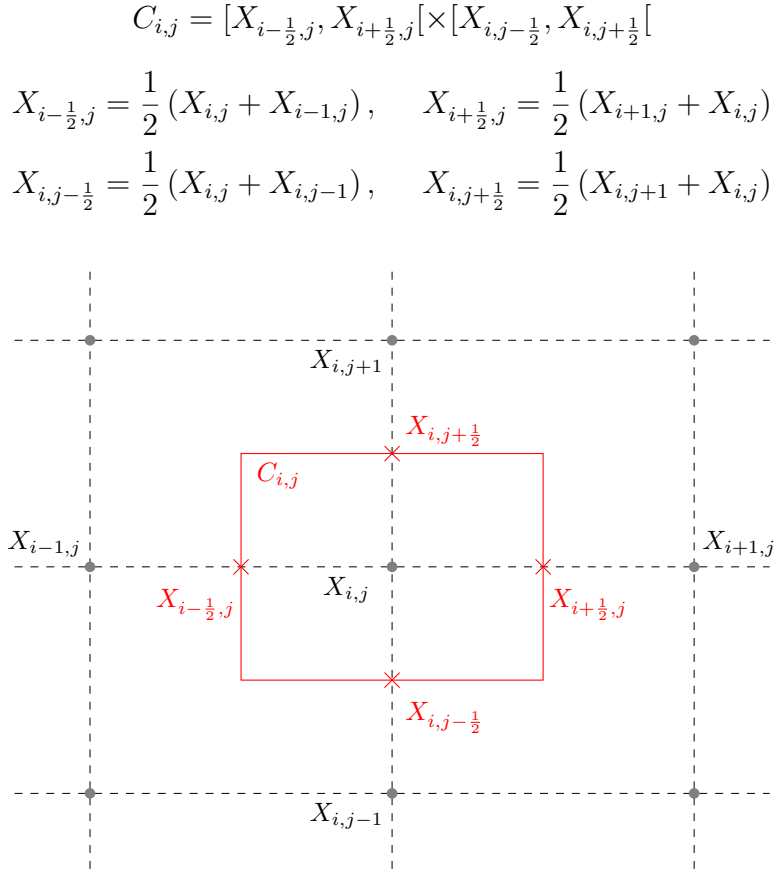
Figure 2.6 – Discretisation de l'espace en un nombre fini de points et visualisation du volume de contrôle élémentaire C_{i,j} dans une approche 2D de la méthode des volumes finis.
