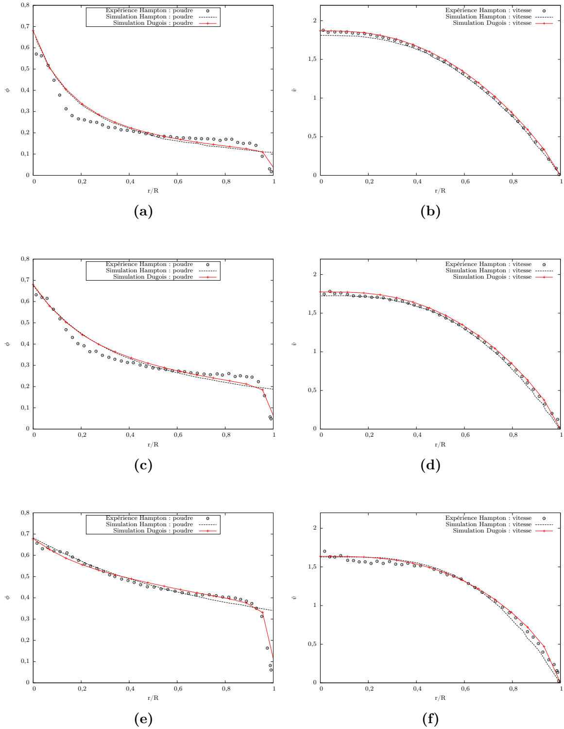
Figure 3.7 – Profils radiaux expérimentaux de fraction \phi^s (gauche) et vitesses \hat{u} (droite) en régime établi ( \circ ). Comparaison aux résultats obtenus avec le modèle de Phillips originel (---) et le modèle modifié dans cette thèse (—) dans la configuration a/R = 0,0256 , pour des suspensions initialement homogènes à (a)(b) \phi_0^s = 0,20 , (c)(d) \phi_0^s = 0,30 et (e)(f) \phi_0^s = 0,45 .
