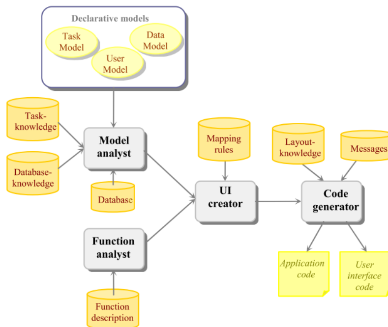
Figure 46 Les composants principaux de leur architecture de génération d'interface et de codes
