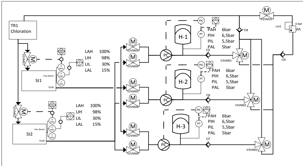
Figure 22 Schéma P&ID d'un système de transfert de fluide
