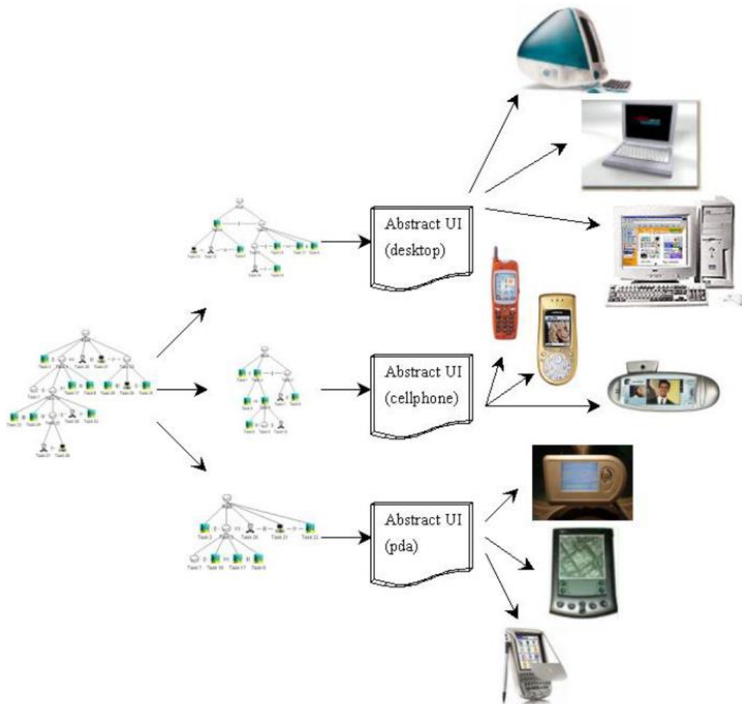
Figure 41 Les transformations supportées par TERESA (Berti et al. 2003)
