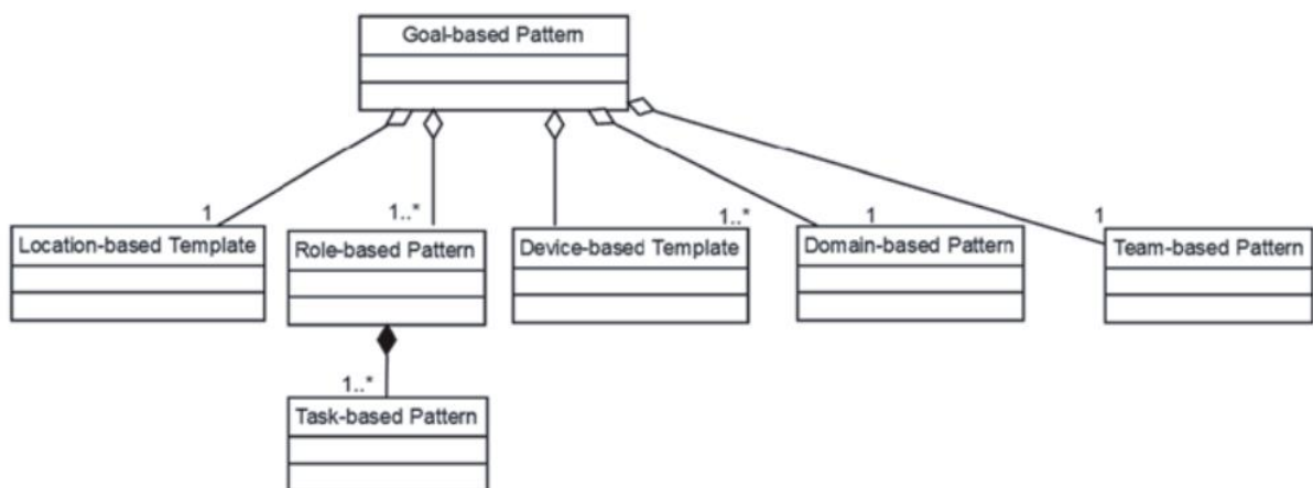
Figure 31 Les catégories de patterns pour un smart meeting room
