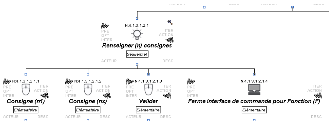
Figure 66 Extrait du pattern de tâches pour décrire la fonction de transfert entre deux soutes
