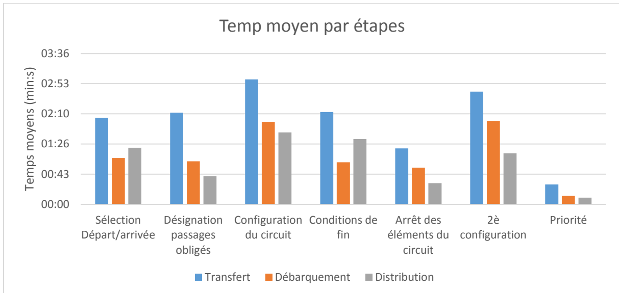
Figure 148 Temps moyens de réalisation des étapes selon la fonction
