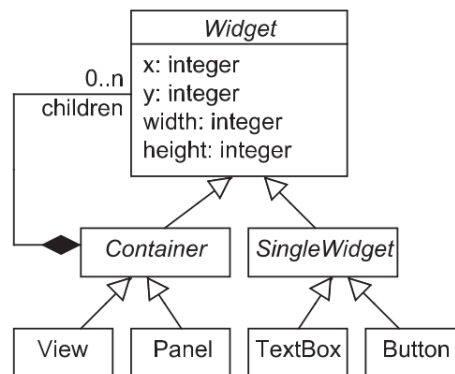
Figure 59 Modèle basique de GUI (Ramón et al. 2016)
