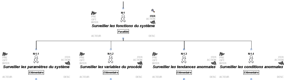
Figure 34 Représentation graphique de la sous-tâche « Surveiller les fonctions du système avec K-MADe
