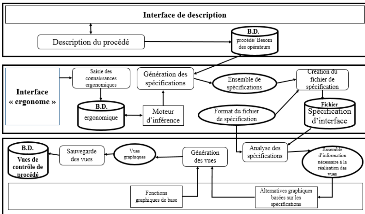
Figure 15 Architecture du système ERGO-CONCEPTOR
