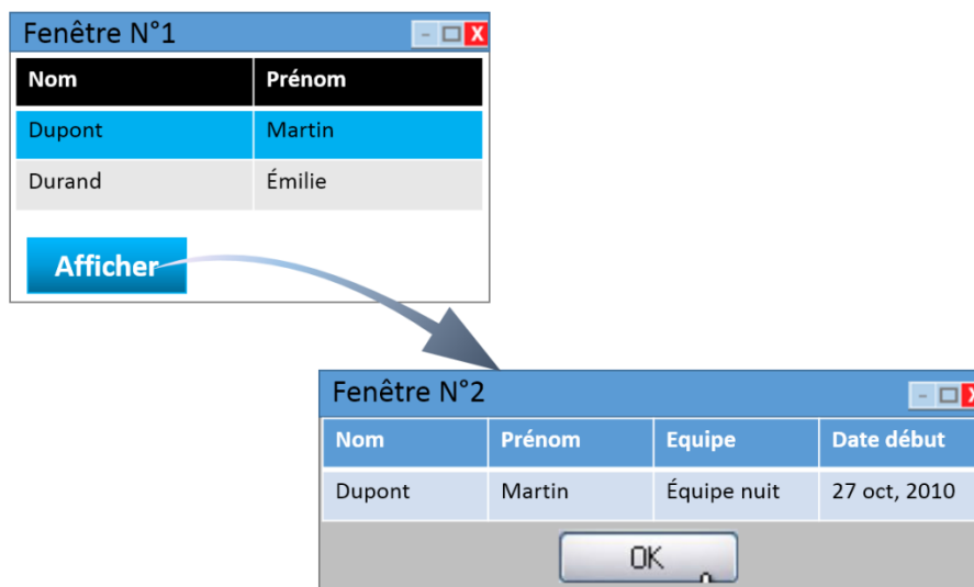
Figure 39 Exemple de dialogue inter-fenêtre
