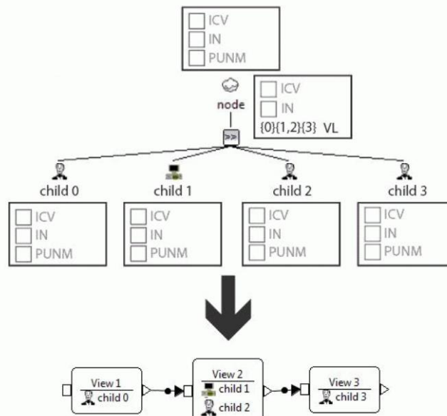
Figure 45 Transformation d'un modèle de tâches annoté
