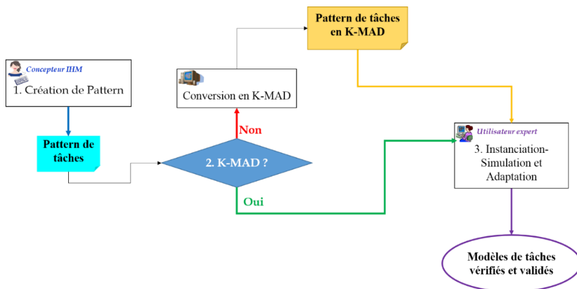
Figure 38 Démarche globale d'obtention des patterns à partir des modèles de tâches
