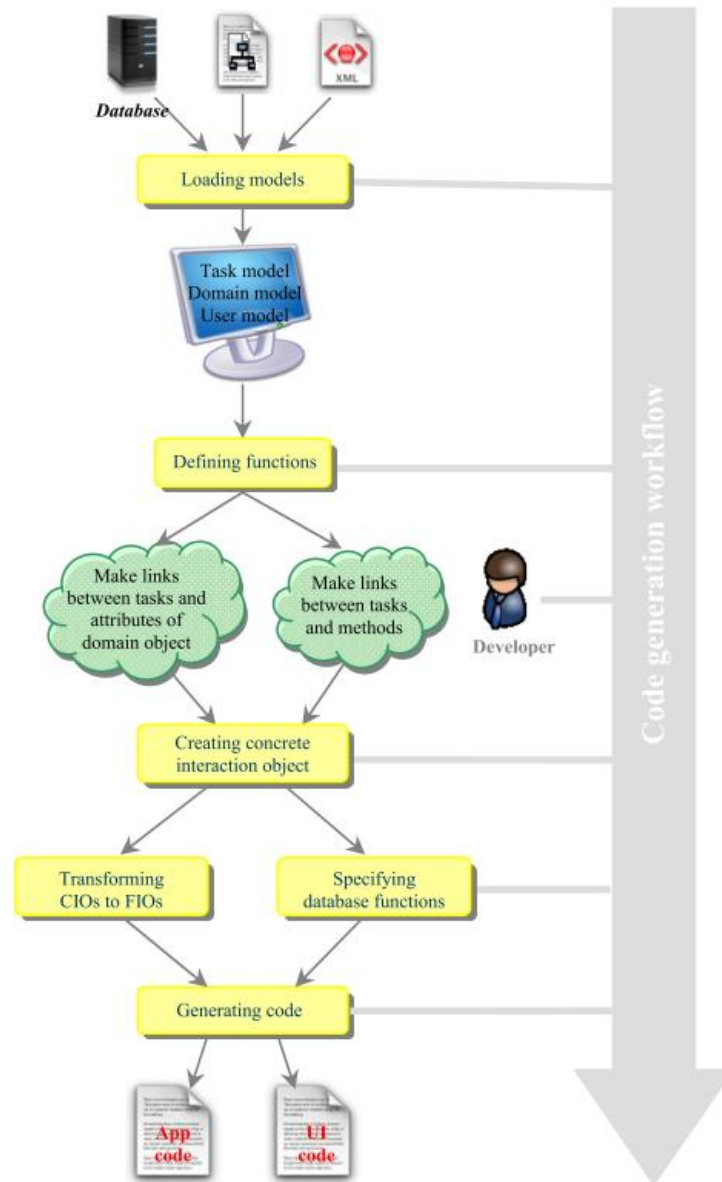
Figure 47 Flot de génération de code : interface utilisateur générée à partir du modèle de tâches, du modèle de domaine et du modèle de l'utilisateur.
