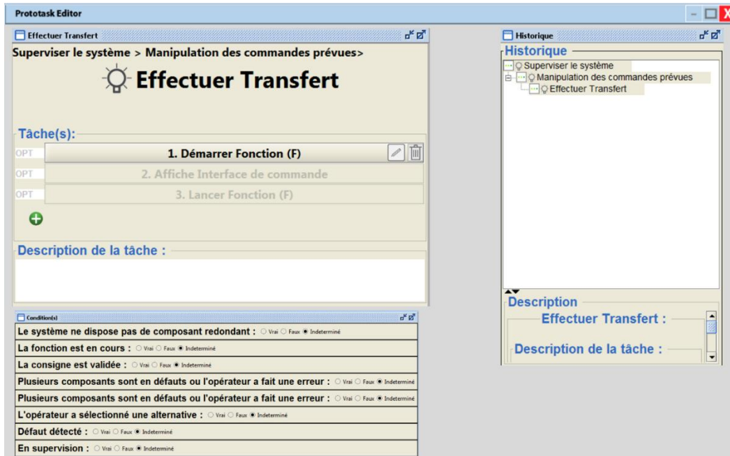
Figure 112 Prototask Editor – Changement de nom d'une tâche
