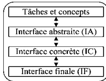
Figure 13 Modèles fondamentaux de CAMELEON
