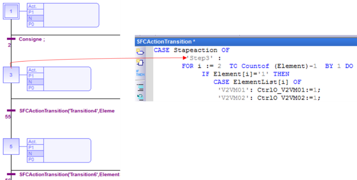
Figure 101 Extrait du résultat de l'opération de génération de codes de commande
