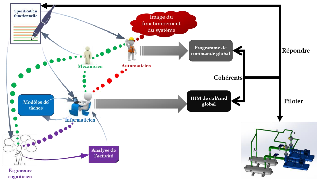
Figure 18 Conception d'IHM et de programme de commande globaux
