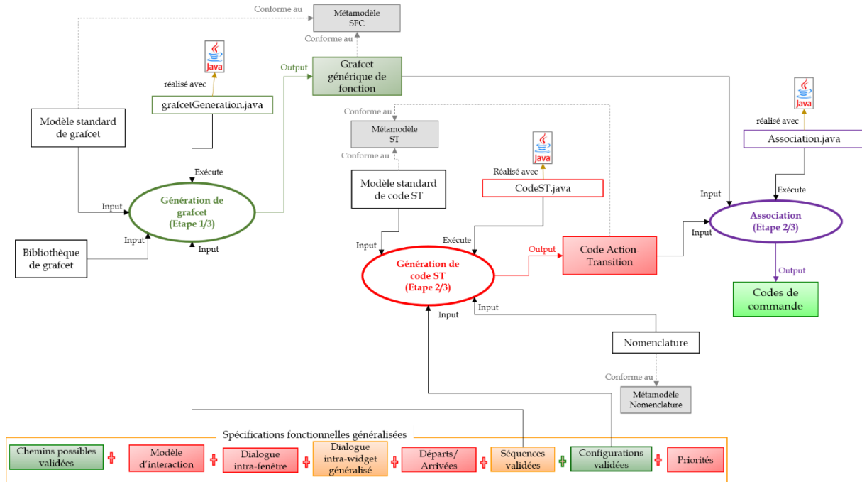
Figure 100 Détail de la génération de codes de commande
