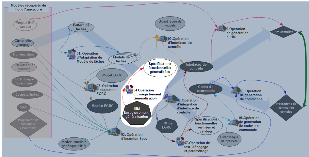
Figure 87 Opération d'enregistrement-généralisation
