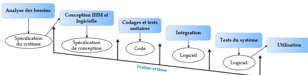
Figure 9 Modèle de Long
