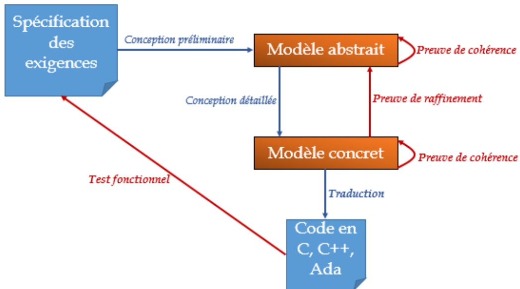
Figure 21 Processus de spécification avec B
