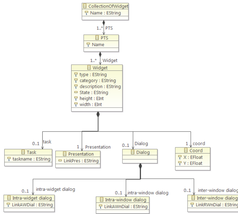
Figure 92 Méta-modèle Collection de Widgets
