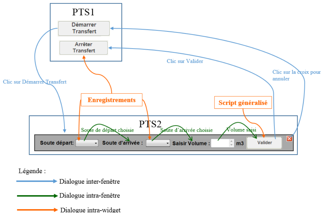
Figure 131. Synthèse de la génération du dialogue à tous les niveaux
