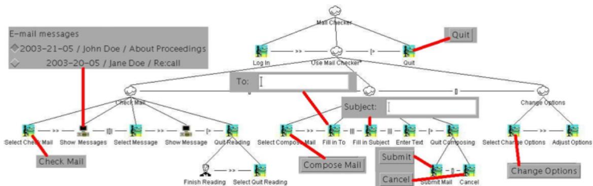
Figure 42 Exemple d'un diagramme CTT annoté avec les widgets associés aux tâches (Caffiau 2009)
