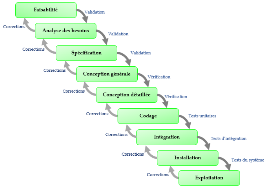
Figure 5 Modèle en cascade
