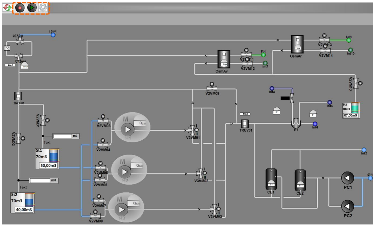
Figure 118 Résultat de l'opération d'insertion Spec - IHM d'EGRC
