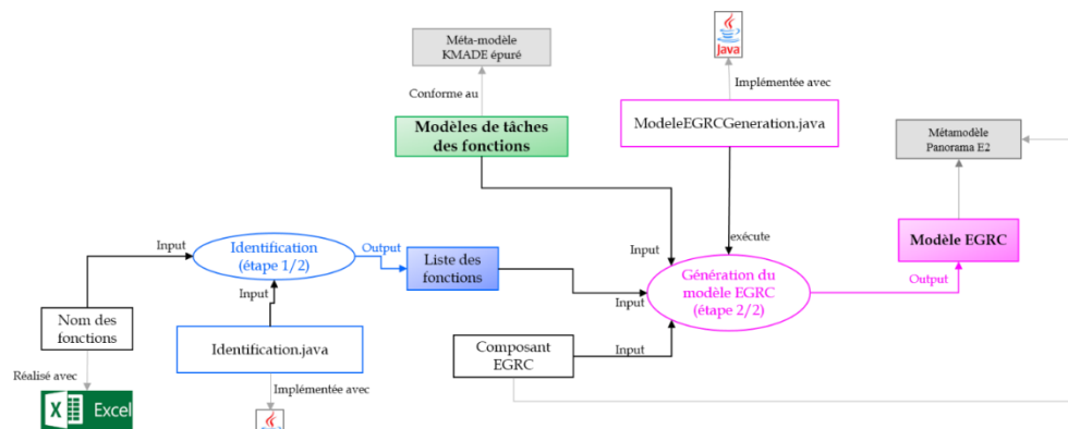
Figure 70 Détail de l'opération d'adaptation du modèle EGRC
