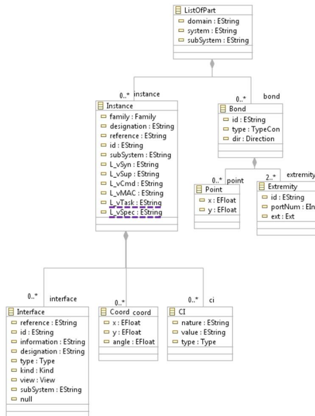
Figure 77 Extension du méta-modèle de la nomenclature
