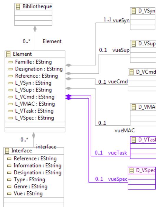
Figure 74 Méta-modèle de la bibliothèque d'Anaxagore
