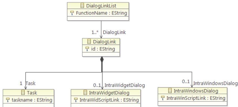
Figure 55 Méta-modèle de liaison tâches-dialogue
