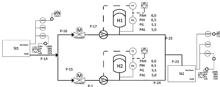
Figure 64 Exemple de P&ID
