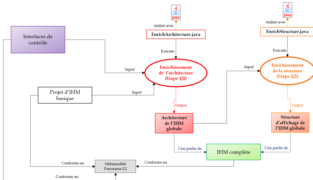
Figure 105 Détail de l'opération de génération d'IHM
