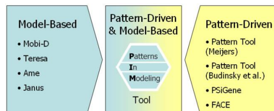
Figure 29 Objectif de l'outil PIM
