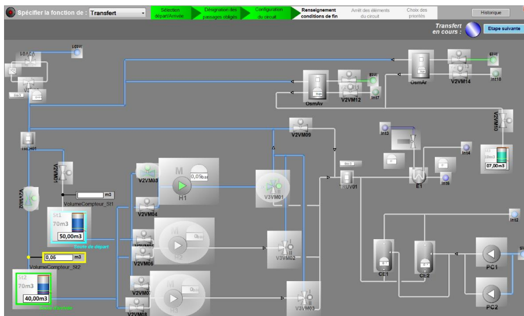
Figure 156 Animation « transfert en cours » en haut à droite
