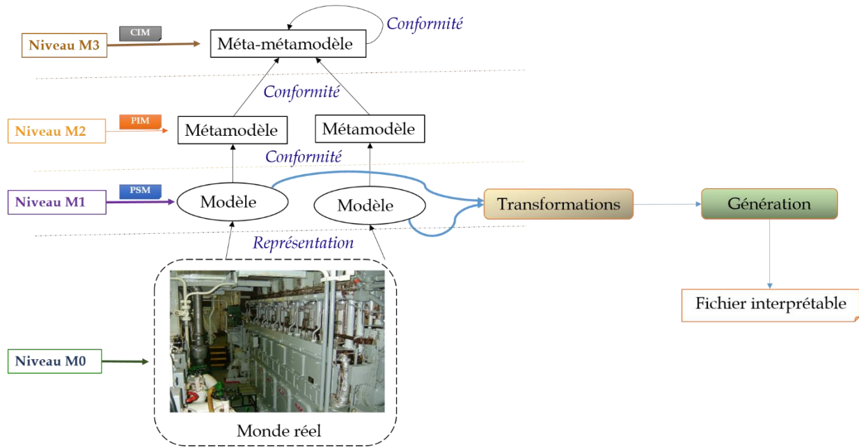
Figure 12 L'approche de l'IDM
