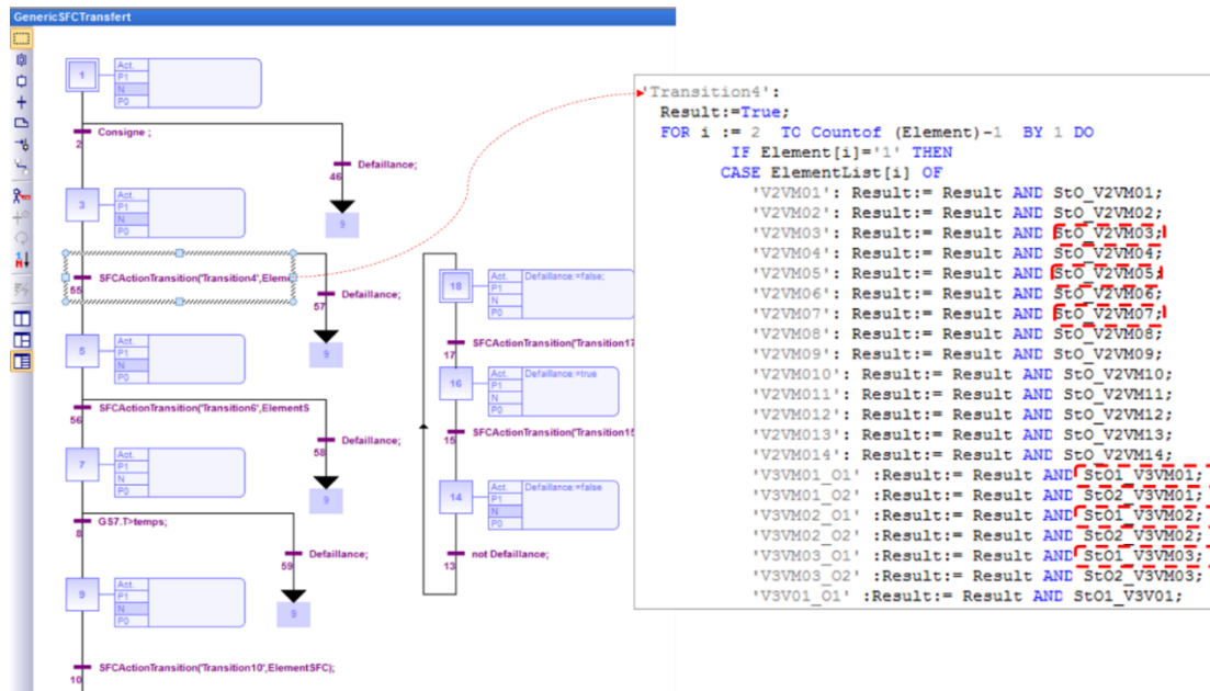
Figure 137 Extrait du résultat de la génération du code global de commande de la fonction de transfert
