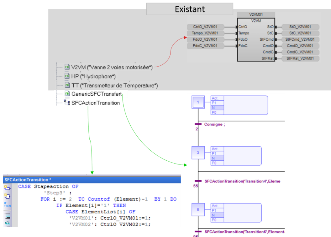
Figure 108 Extrait du résultat de l'opération de génération de commande
