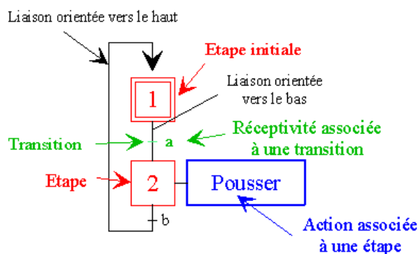
Figure 61 Exemple de représentation du grafcet
