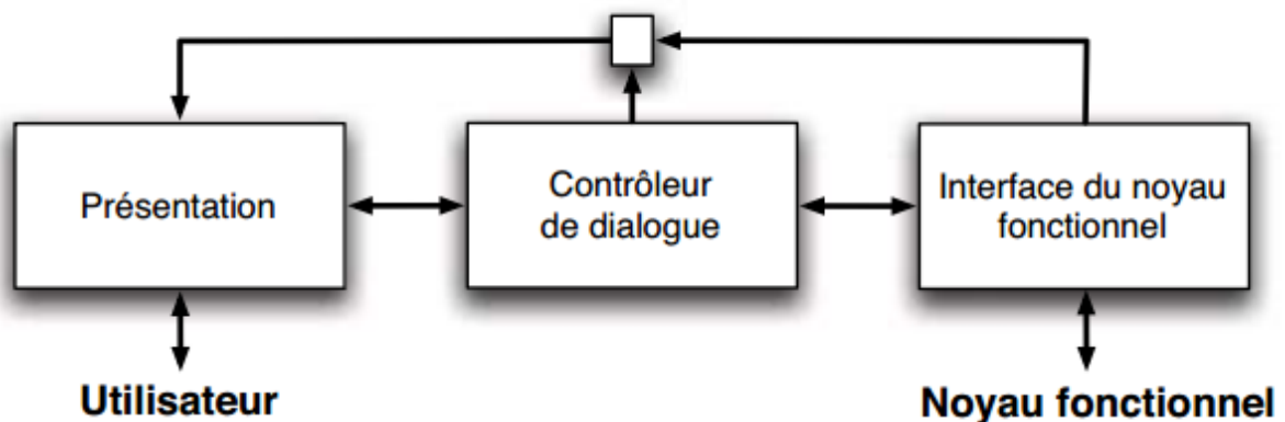
Figure 54 Le modèle de Seeheim (Pfaff, 1985) (Samaan 2006)
