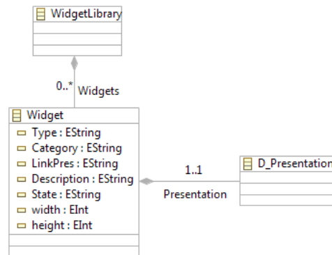
Figure 57 Métamodèle de la bibliothèque de widgets décrit avec EMF
