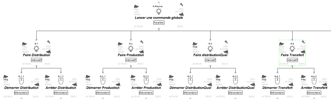
Figure 128. Extrait du modèle de tâches de lancement de contrôle-commandes globaux
