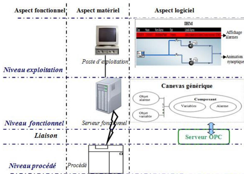
Figure 63 Schéma d'architecture de Panorama E2 (Goubali et al. 2014)
