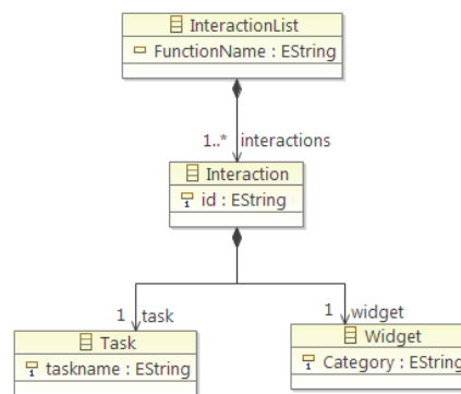
Figure 56 Un métamodèle pour le modèle d'interaction décrit avec EMF
