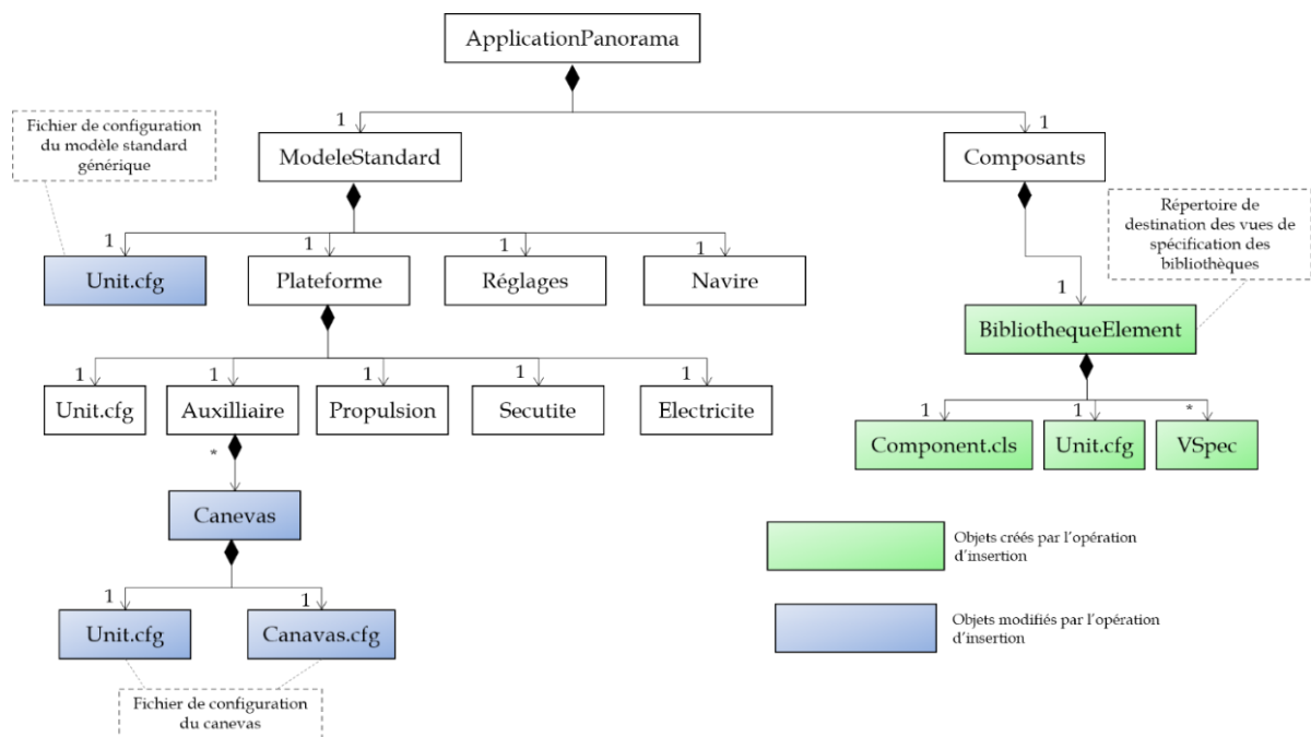
Figure 81 Structure du modèle standard générique sous Panorama E2 (Bignon 2012)
