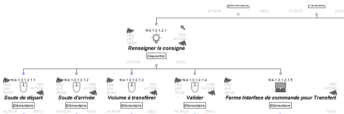
Figure 67 Extrait de modèle de tâches adapté à la fonction Transfert
