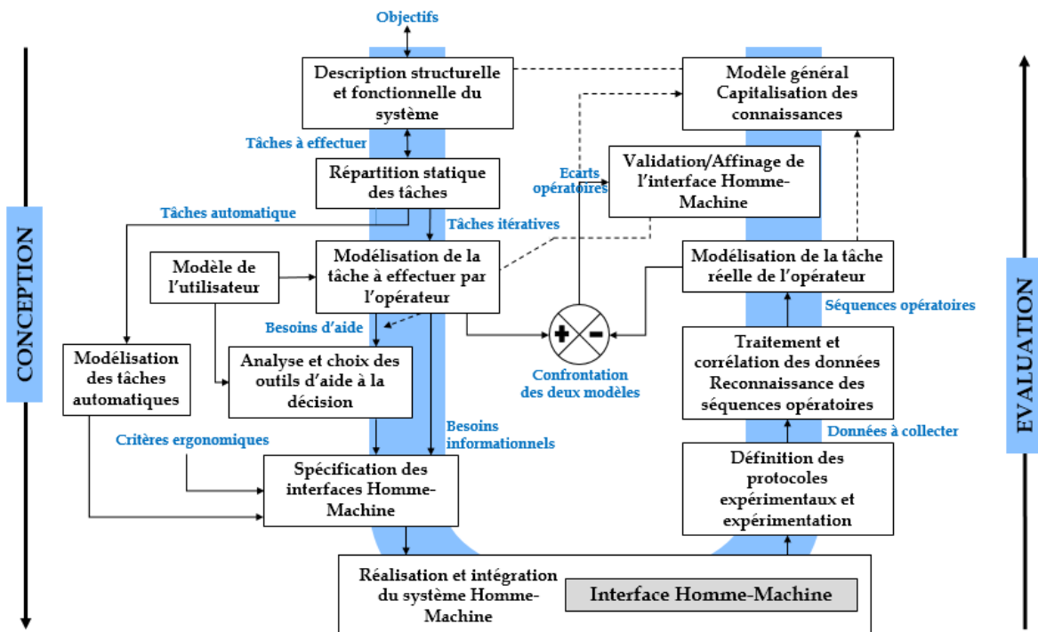
Figure 10 Modèle en U
