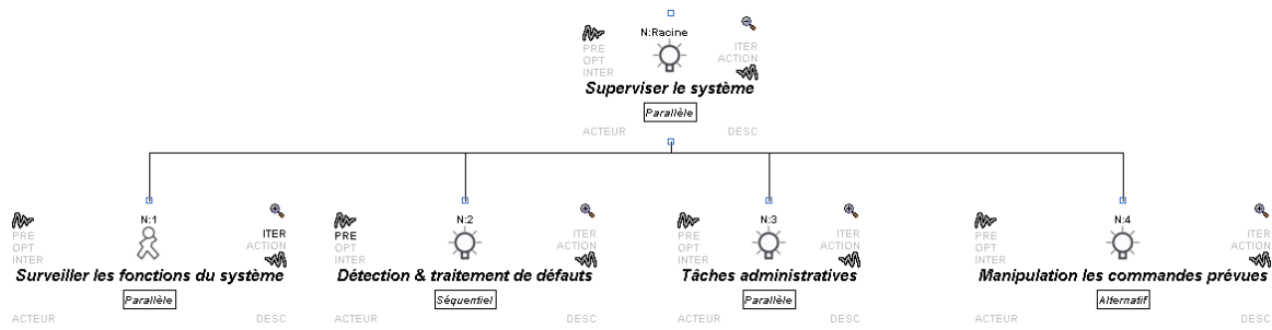
Figure 33 Description de la tâche « Superviser le système avec K-MADe
