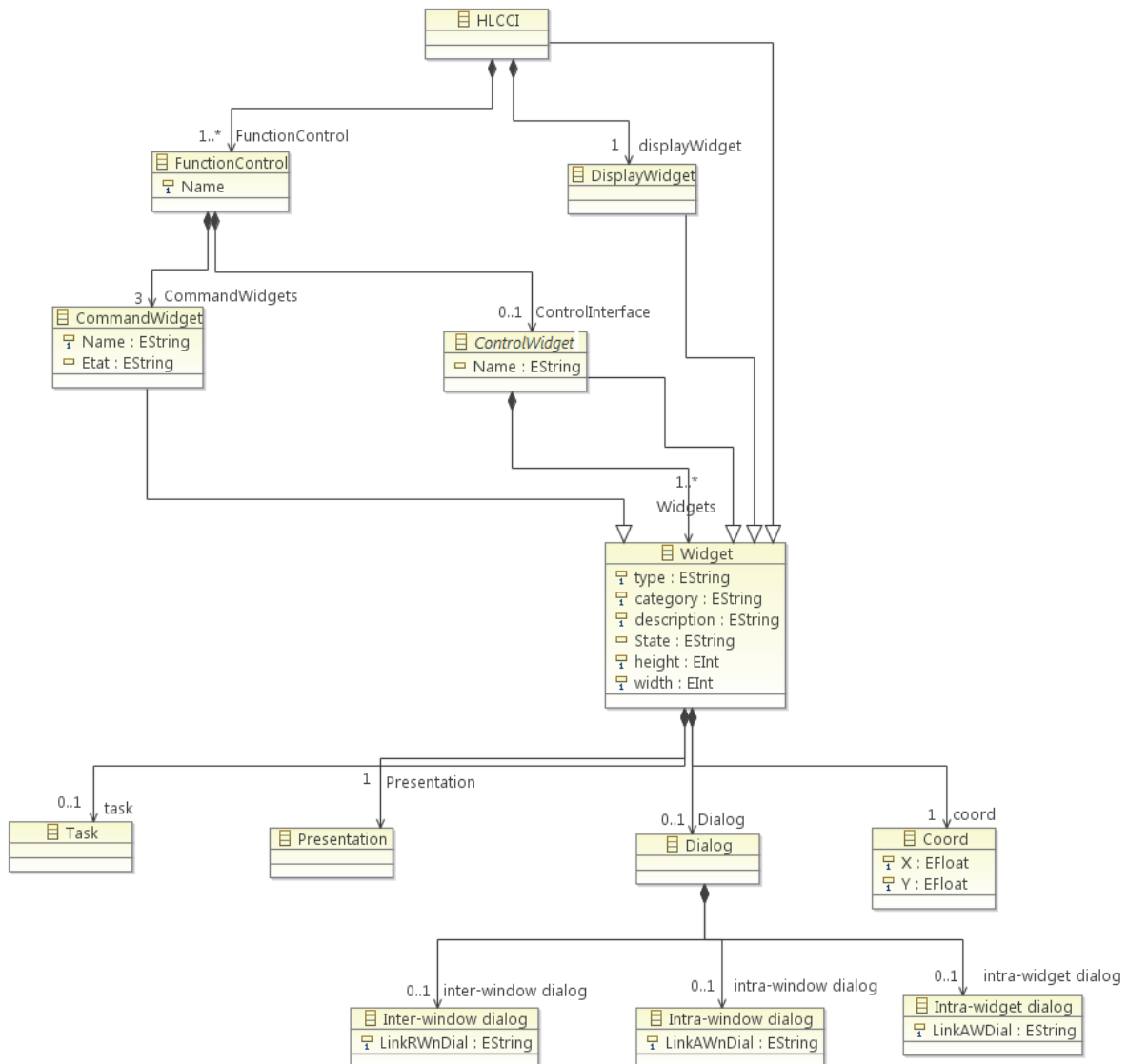
Figure 60 Un métamodèle pour le modèle d'interface décrit avec EMF
