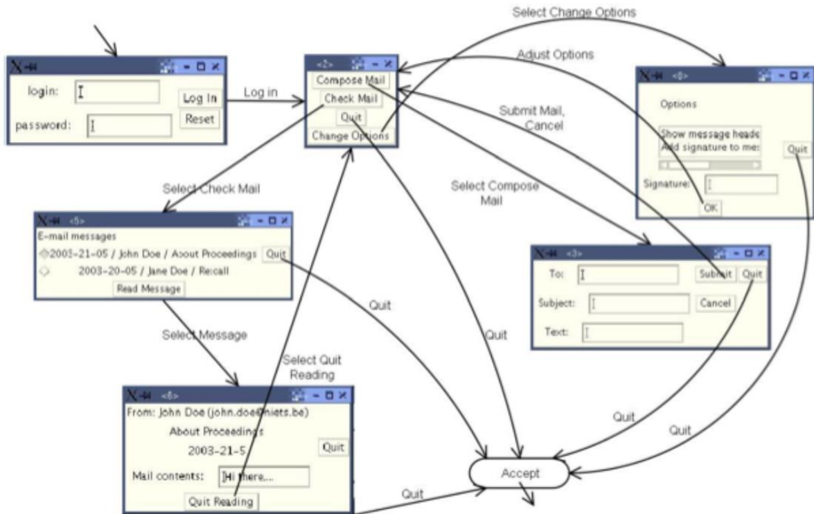
Figure 44 Le dialogue de l'application exemple (Caffiau 2010) ].
