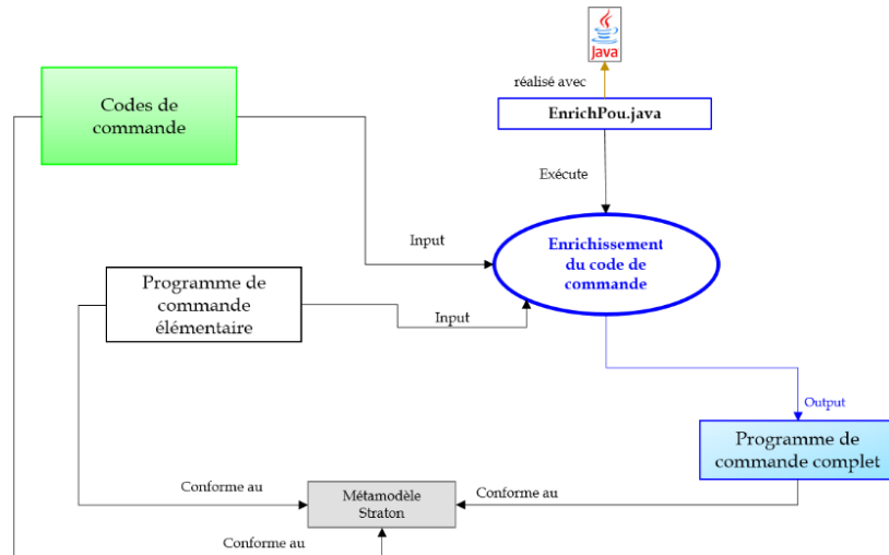
Figure 107 Détail de l'opération de génération de code de commande
