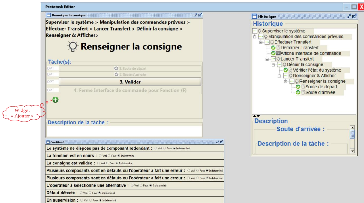
Figure 113 Prototask Editor – illustration du widget « ajouter »
