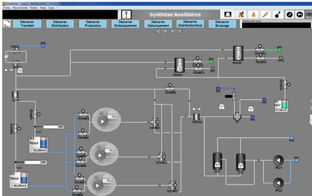
Figure 139 IHM complète - Résultat de l'opération de génération d'IHM
