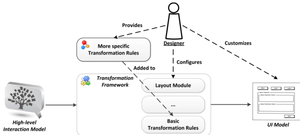
Figure 49 intégration du Layout Hints dans UCP:UI
