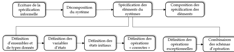
Figure 20 Processus de développement d'une spécification avec Z
