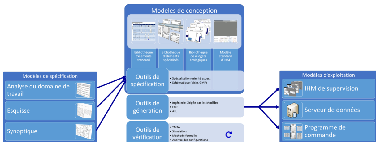
Figure 17 Ecosystème d'Anaxagore
