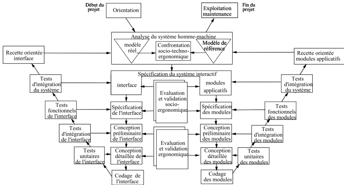
Figure 11 Modèle Nabla
