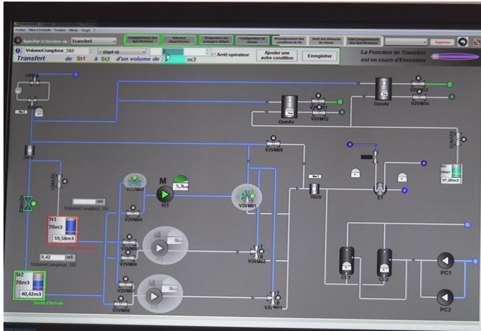
Figure 143 Glisser/Déposer
