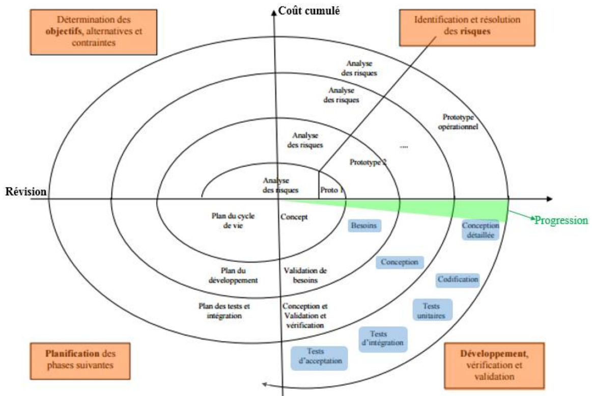
Figure 7 Modèle en spirale
