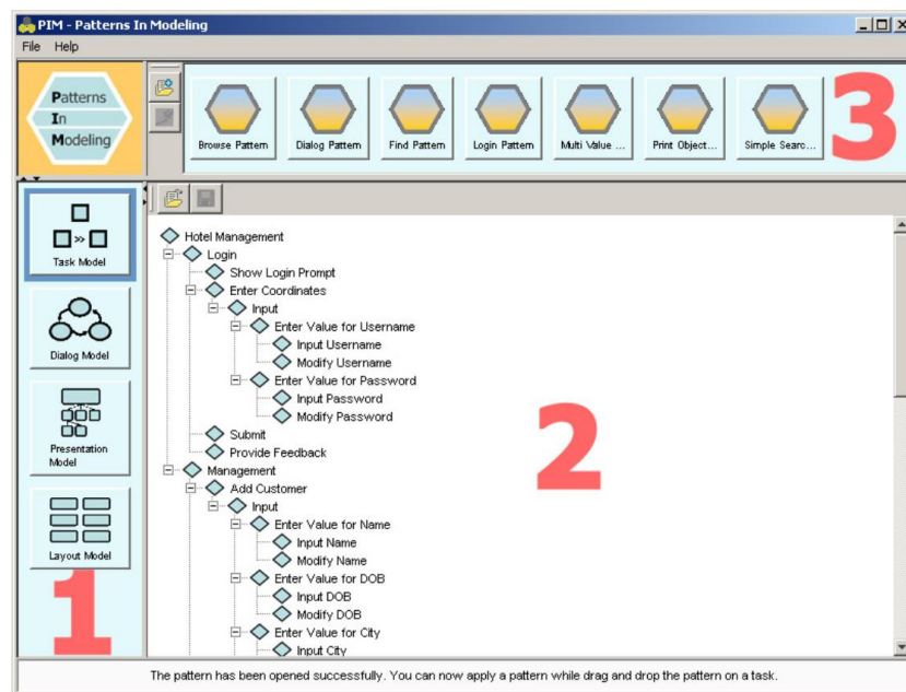
Figure 26 L'interface utilisateur de l'outil PIM
