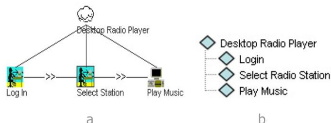
Figure 27 Modèle de tâches pour écouter de la musique à travers une station radio. (a) décrit avec CTTE. (b) une fois chargée sur PIM.
