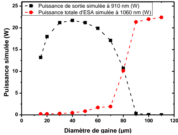
Figure 1.26 : Evolution des puissances de sortie à 910 nm (noir) et totale à 1060 nm (rouge) en fonction du diamètre de gaine pour un diamètre de cœur de 15µm et un miroir M_1 non réfléchissant à 1060 nm
