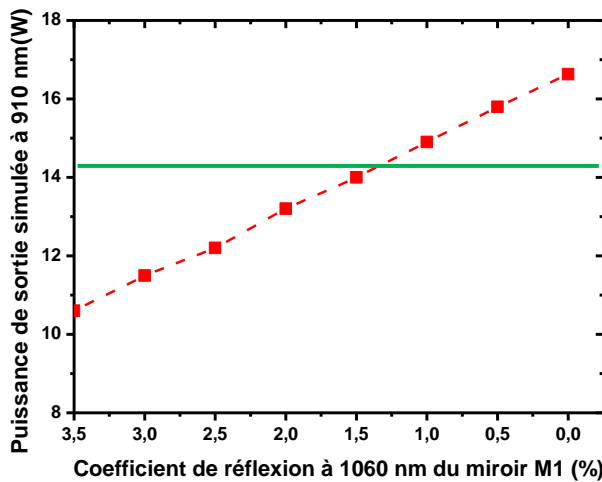
Figure 1.27 : Evolution de la puissance de sortie à 910 nm calculée pour une fibre 15/60 en fonction du coefficient de réflexion à 1060 nm pour R_1^{910} = 3,5\% et des pertes de couplage C fixées à 15%
