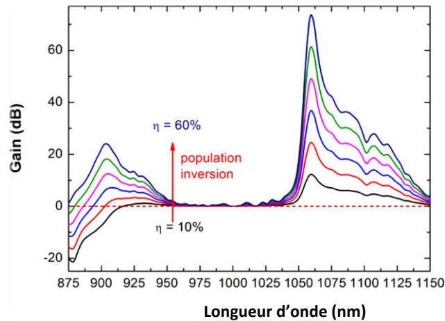
Figure 1.11 : Gain non-saturé calculé dans une fibre dopée Nd 3+ pour différentes inversions de population ( L = 4 m et concentration de 4.10^{18} at.cm -3 )
