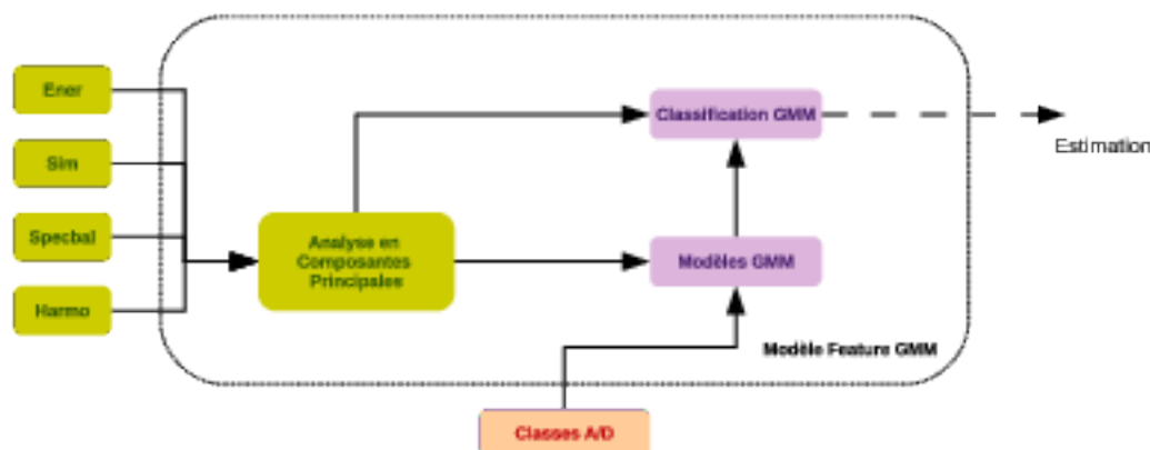
FIGURE 4.4 – Schéma du modèle B (Feature-GMM).
