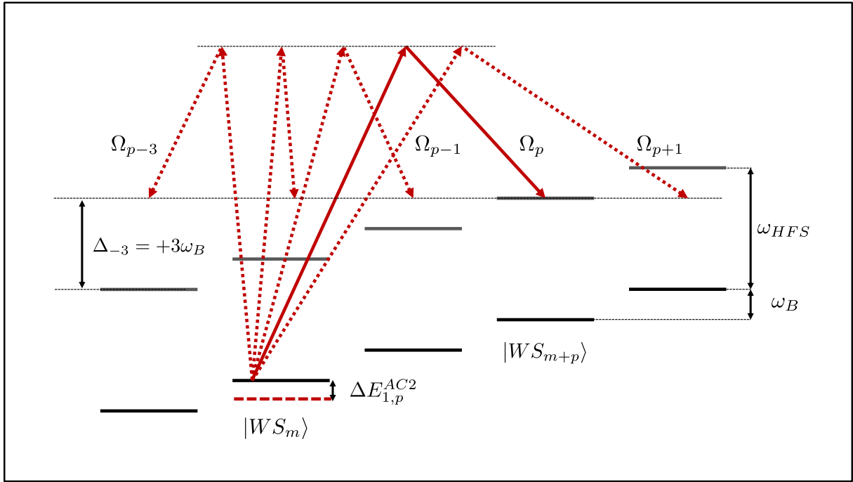
FIGURE III.10 – Déplacement lumineux différentiel à deux photons pour une échelle de Wannier-Stark. Lors d'une transition \Delta m = p , la paire de faisceaux Raman induit plusieurs couplages non-résonnants avec l'ensemble des états de Wannier-Stark |WS_i\rangle désaccordés de \Delta = (i - p) \times \omega_B . La transition résonnante est alors décalée d'une quantité \Delta E_{1,p}^{AC2} . Par soucis de simplicité, seul le déplacement de l'état |WS_m, F = 1\rangle a été représenté, l'état |WS_{m+p}, F = 2\rangle étant déplacé d'une même quantité dans le sens opposé.
