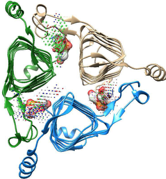
Figure 4.18: dTDP-4-amino-4,6-dideoxyglucose (surface translucide) à l'interface des 3 chaînes (rubans bleus, verts et jaunes) de la galactoside O-acétyltransferase (PDB ID 3vbi). Les points de cavité sont colorés en fonction de leurs propriétés pharmacophoriques (hydrophobe, gris; aromatique, vert; donneur, bleu; positif ionisable, bleu; accepteur; rouge; négatif ionisable, orange)
