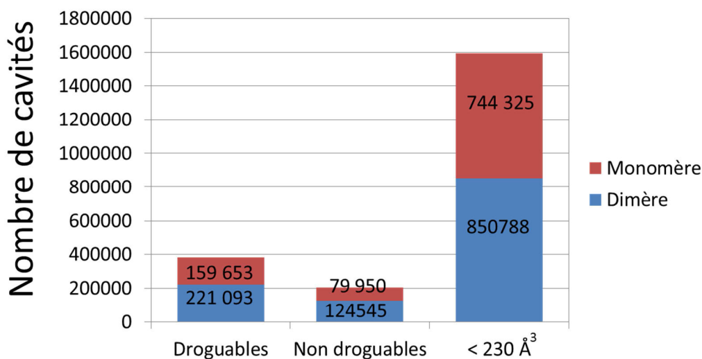
Figure 4.7 : Histogramme empilé des différentes cavités identifiées à la surface des entrées traitées de la PDB possédant une interface biologiquement pertinente. Les cavités de petite taille (< 230 Å 3 ) ne sont pas soumises à une prédiction de droguabilité par VolSite. La quantité de chaque type de cavité est indiquée, soit à la surface d'un dimère soit du dimère dissocié (monomère)
