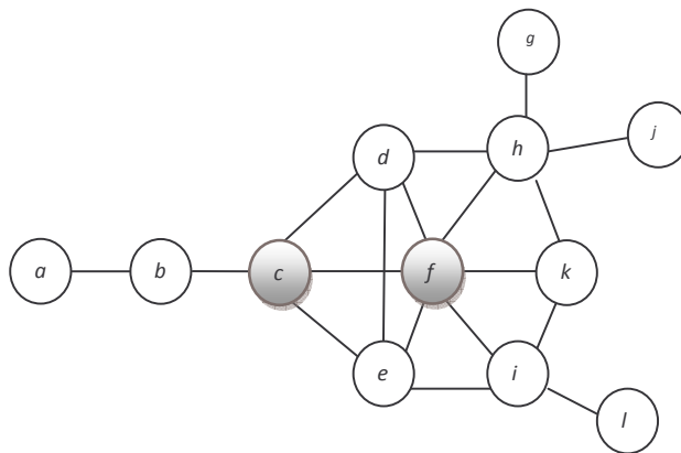
Figure 5..1 Exemple d'un graphe représentant un RCSF. L'ensemble (1,2-saut)-CDS est \{c,f\} .
