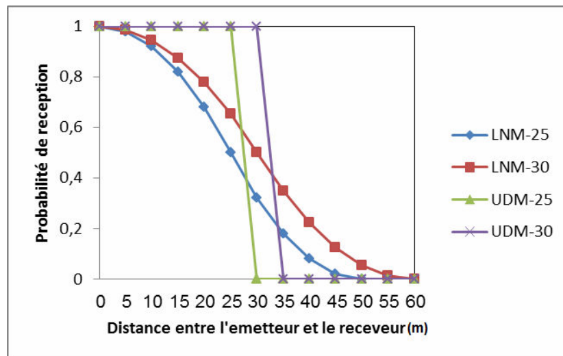
Figure 3.3. Comparaison de probabilité de réception entre LNM et UDM pour différents rayons de transmission
