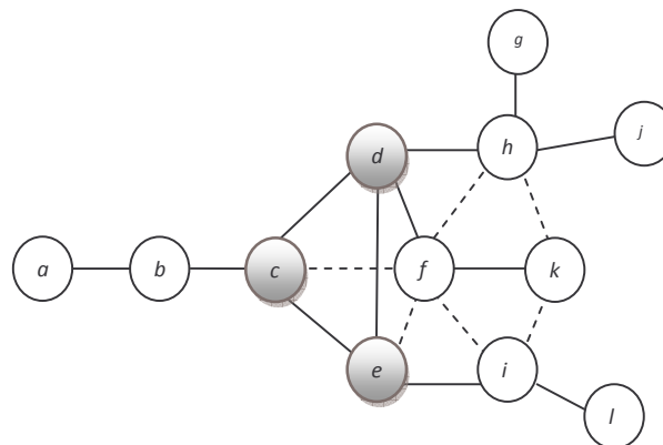
Figure 5..3 Affectation des nœuds dominés à leur dominant approprié : 1ère possibilité
