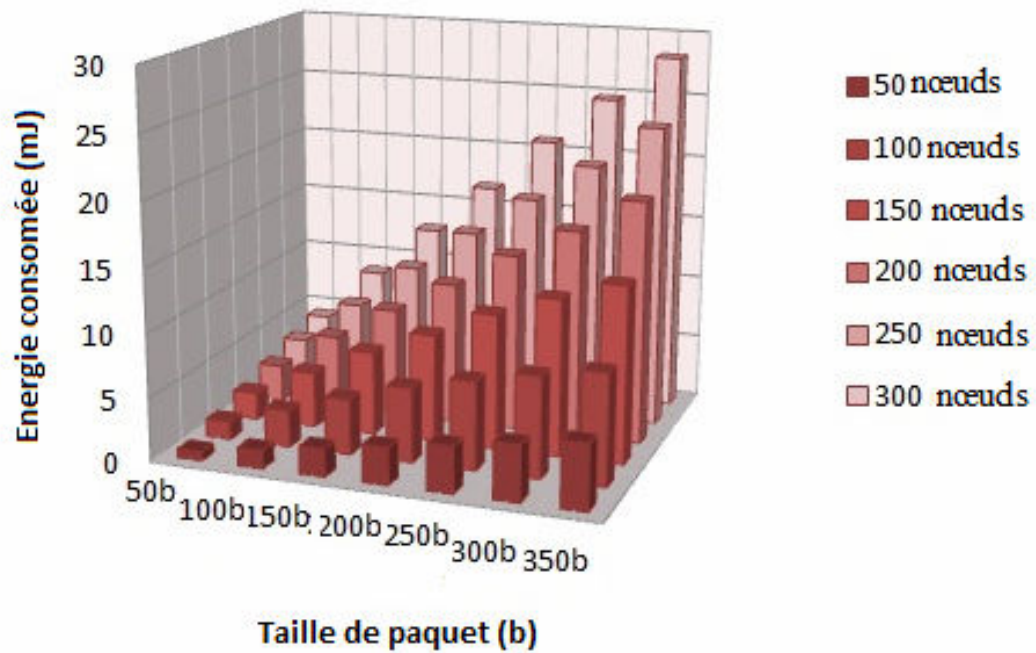
Figure 4.11. Energie totale consommée avec RDS-MRR pour accomplir la diffusion avec des densités différentes et des tailles différentes de paquets
