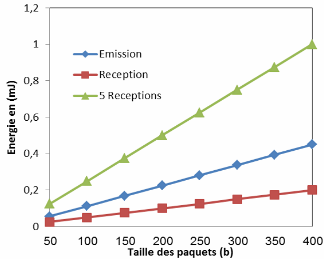
Figure 4.1. Comparaison entre les énergies de réception et d'émission
