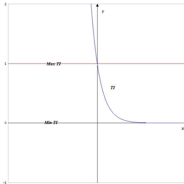
Figure 5..8. Fonction d'indice de confiance entre Max TI=1 et Min TI=0 lorsque v(u) \geq 0
