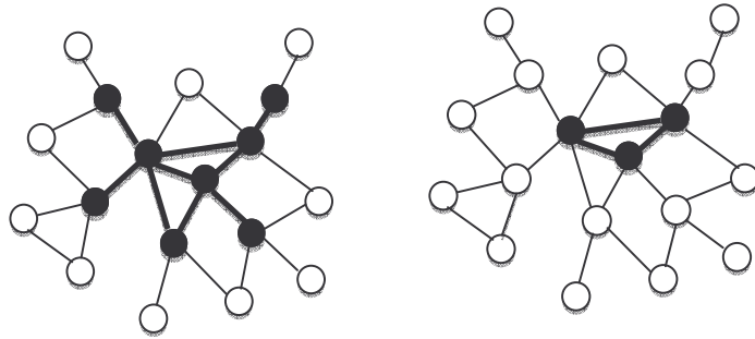
Figure 2.7. Exemple d'un CDS (à gauche) et d'un ensemble 2-saut CDS (à droite) dans un RCSF
