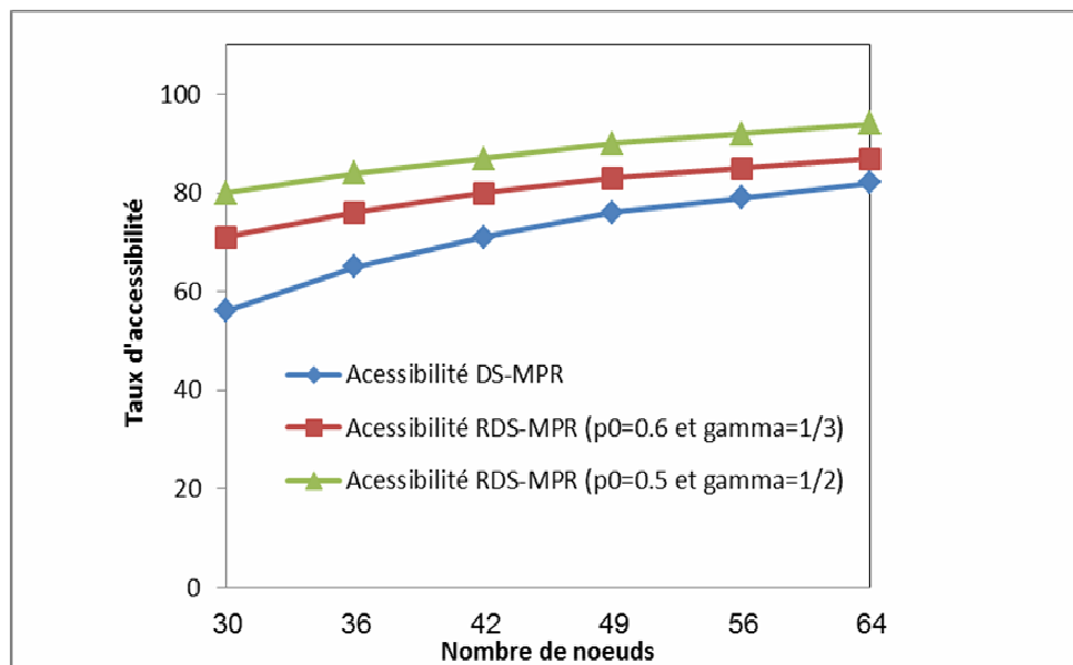
Figure 3.6. Comparaison de l'accessibilité de la méthode DS-MPR et RDS-MPR dans le modèle LNM
