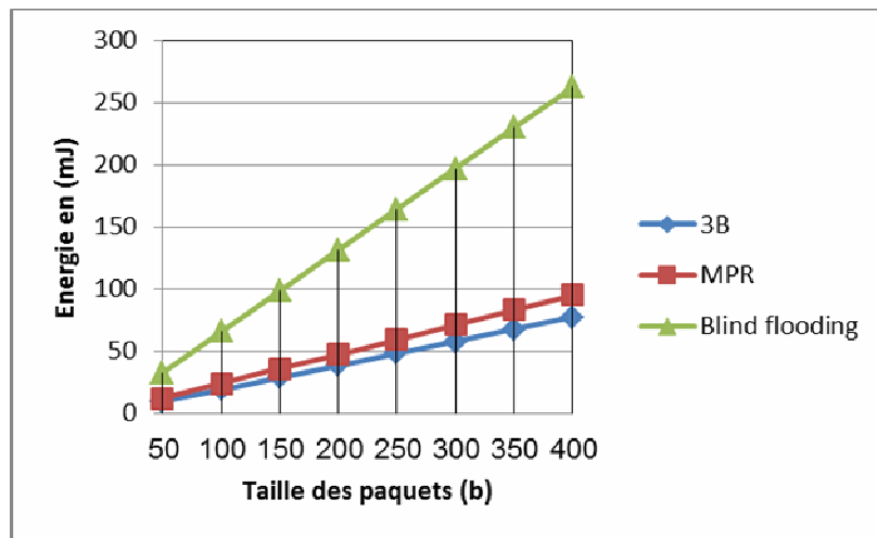
Figure 4.6. Comparaison de l'énergie totale de diffusion pour un réseau de 250 nœuds
