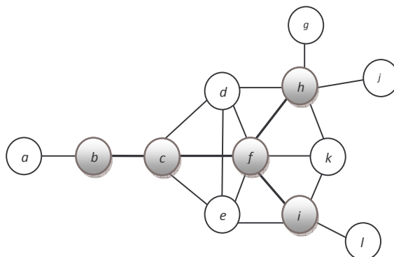
Figure 2.1. L'ensemble \{b,c,f,h,i\} est un CDS du graphe
