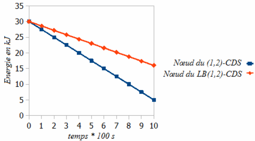
Figure 5.6. Evolution de l'énergie dans le nœud qui a fait plus de communication dans (1,2)-CDS avec une densité égale à 200 et une taille de paquet égale à 200 octets
