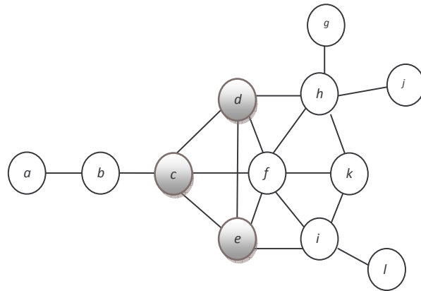
Figure 5..2 Exemple d'un graphe représentant un RCSF. L'ensemble (1,2-saut)-CDS est \{c,d,e\} .
