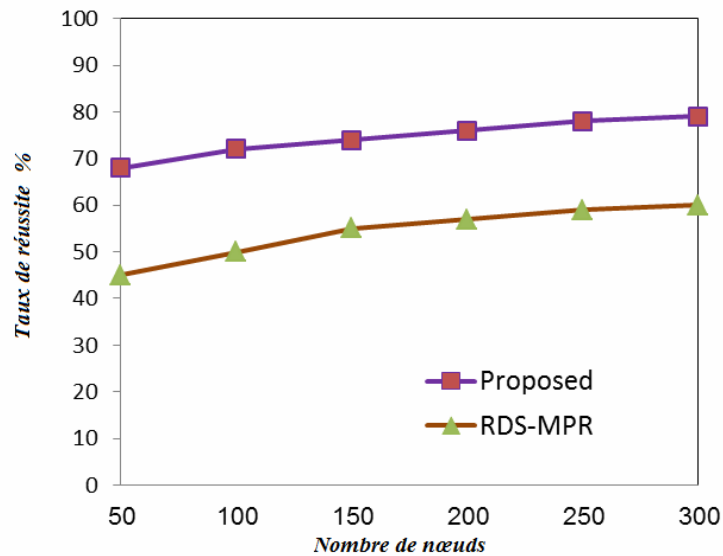
Figure 5.12. Taux de réussite de RRB comparé à RDS-MPR pour un taux de défaillance fixé à 20% et un nombre de nœuds qui varie de 50 à 300
