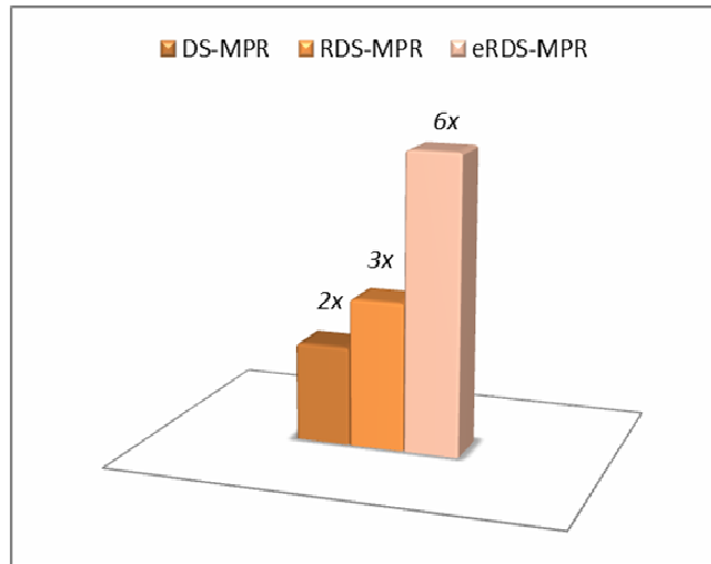
Figure 3.12. Espace mémoire
