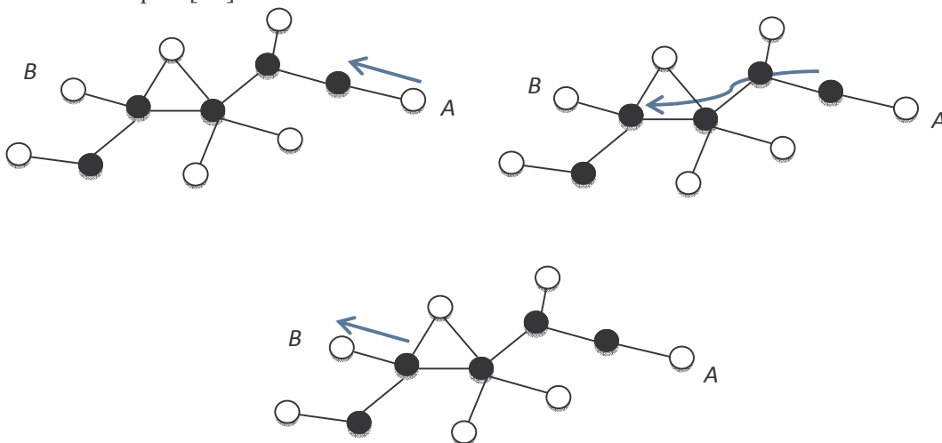
Figure 2.6. Communication à travers un CDS de A vers B
