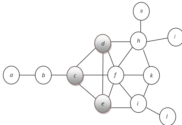
Figure 2.2. L'ensemble \{b,c,e\} est un (2,2-saut)-CDS du graphe
