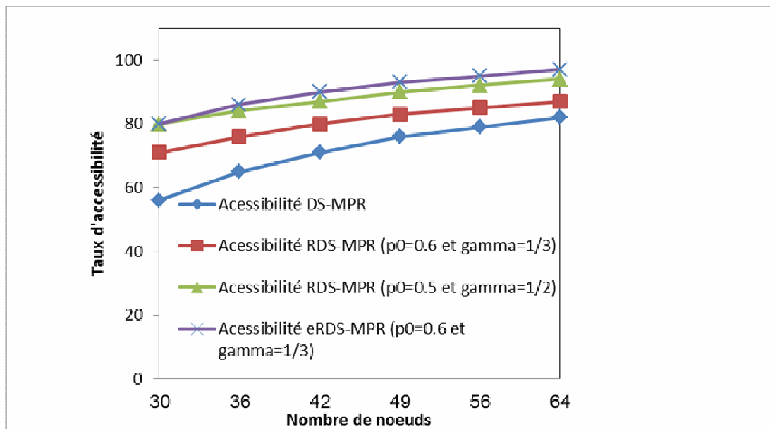
Figure 3.8. Comparaison de l'accessibilité des méthodes DS-MPR, RDS-MPR et eRDS-MPR dans le modèle LNM
