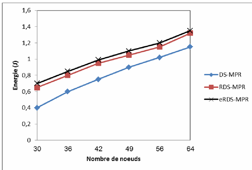
Figure 3.9. Comparaison d'énergie totale consommée pour accomplir la diffusion des méthodes DS-MPR, RDS-MPR et eRDS-MPR.
