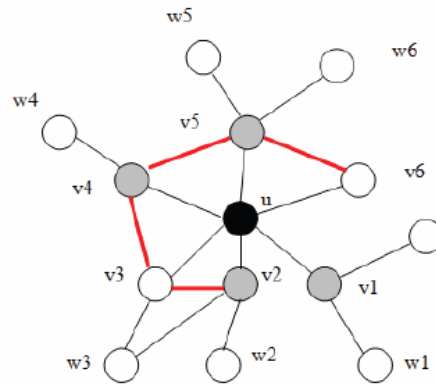
Figure 4.7. Choix des nœuds de relai par RDS-MPR
