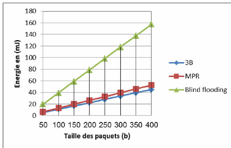
Figure 4.5. Comparaison de l'énergie totale de diffusion pour un réseau de 150 nœuds
