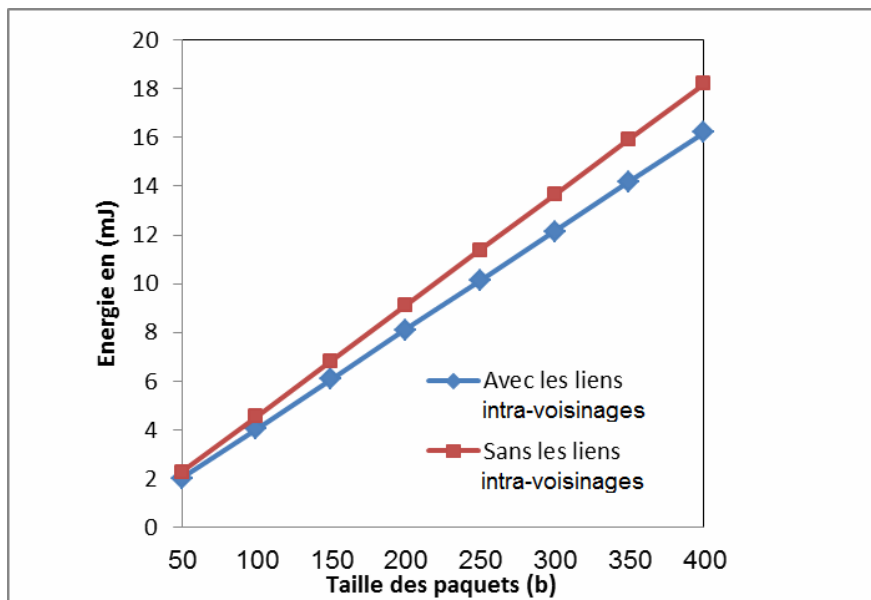
Figure 4.3. Energie de diffusion consommée dans les réseaux de la figure.4.2 avec et sans les liens intra-voisinages
