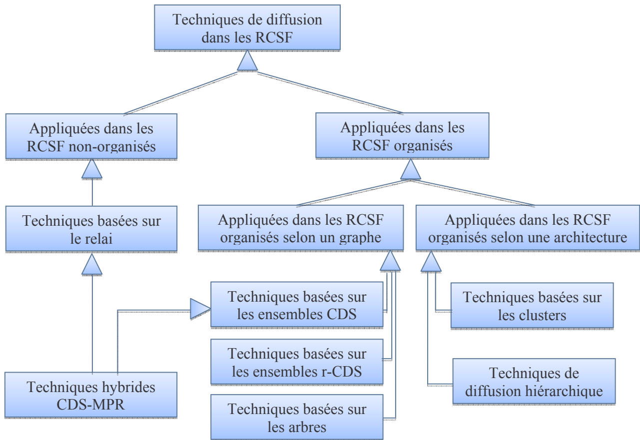
Figure 2.3. Classification des techniques de diffusion dans les RCSF
