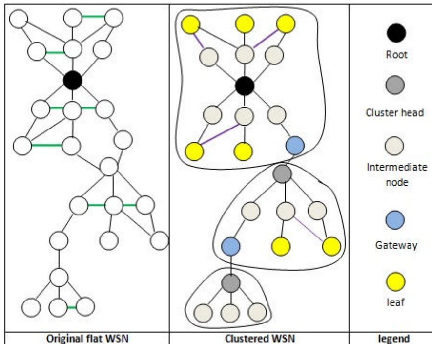
Figure 4.10. Application de SCA à un réseau: les liens intra-niveaux du réseau d'origine sont éliminés mais les liens d'un niveau à l'autre dans le même cluster sont conservés.
