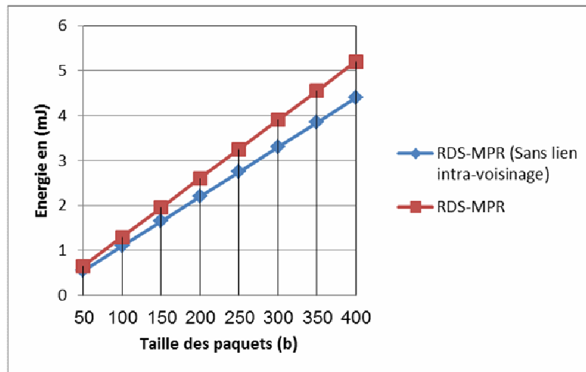
Figure 4.8. Energie totale consommée de diffusion dans le réseau de la figure.4.7 en appliquant RDS-MPR avec et sans liens intra-voisinage
