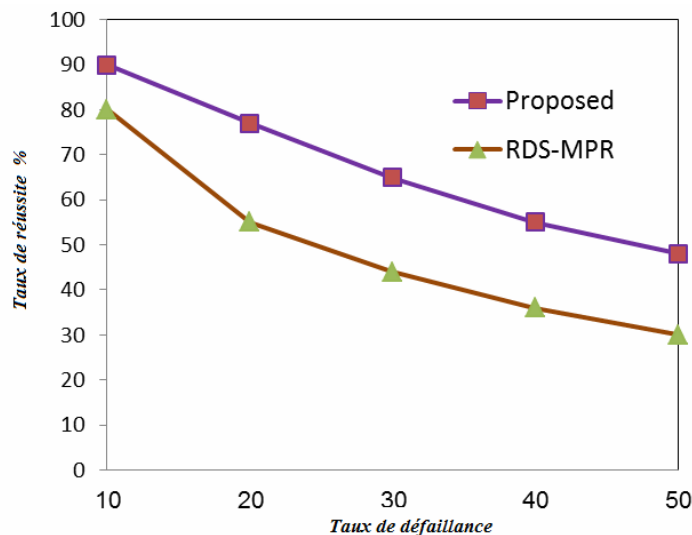
Figure 5.11. Taux de réussite de RRB comparé à RDS-MPR pour un taux de défaillance de nœuds qui varie entre 10 et 50% du nombre total des nœuds-capteurs
