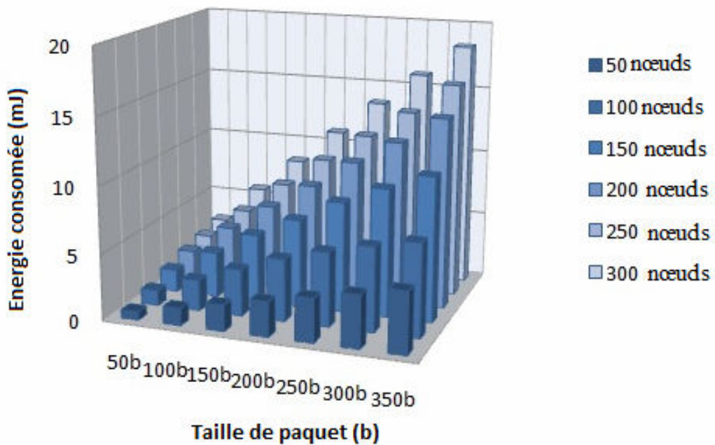
Figure 4.12. Energie totale consommée avec MCR pour accomplir la diffusion avec des densités différentes et des tailles différentes de paquets
