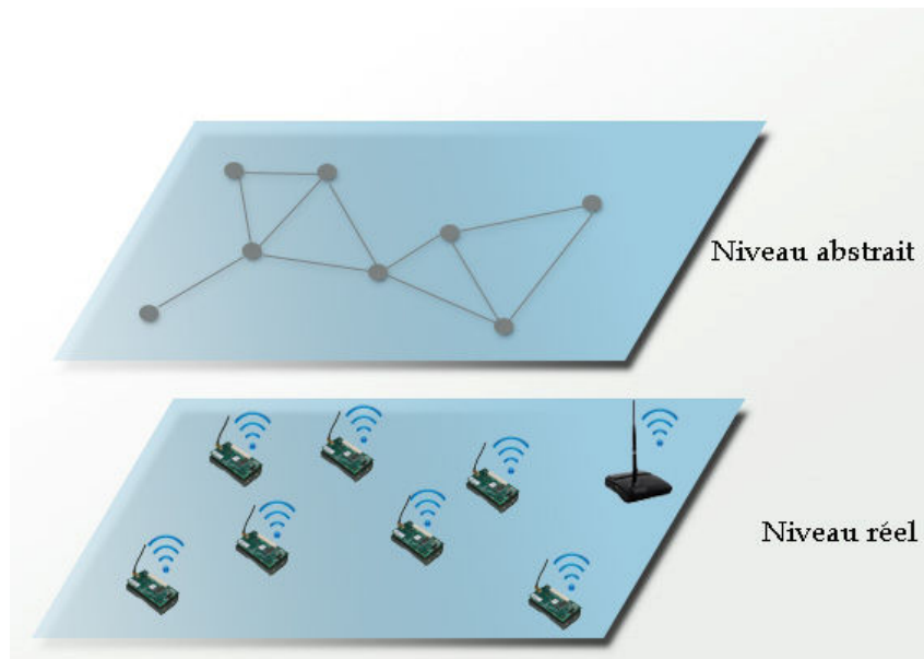
Figure 1.10. Abstraction d'un RCSF
