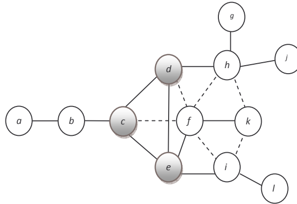
Figure 5.4 Affectation des nœuds dominés à leur dominant approprié: 2ème possibilité
