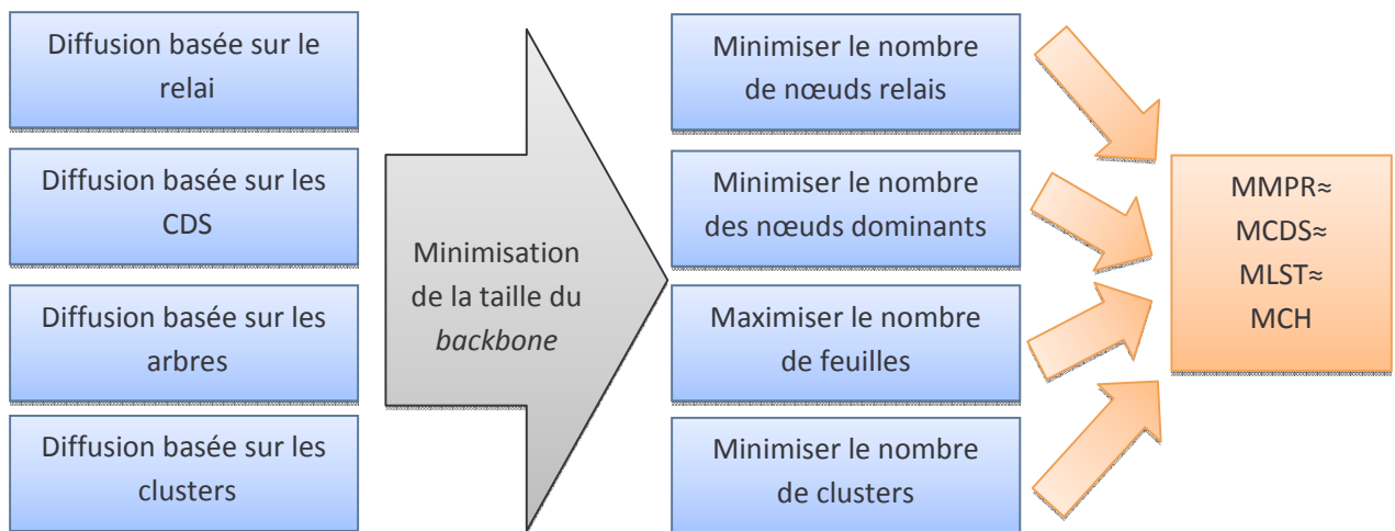
Figure 2.9. Concept de minimisation dans les RCSF
