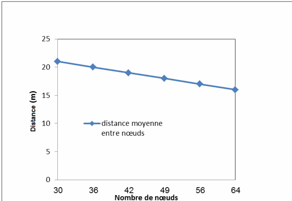
Figure 3.4. La distance moyenne entre les nœuds selon leur rayon de communication
