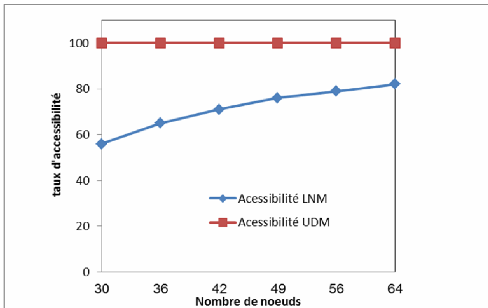
Figure 3.5. Comparaison de l'accessibilité de la méthode DS-MPR dans les deux modèles LNM & UDM
