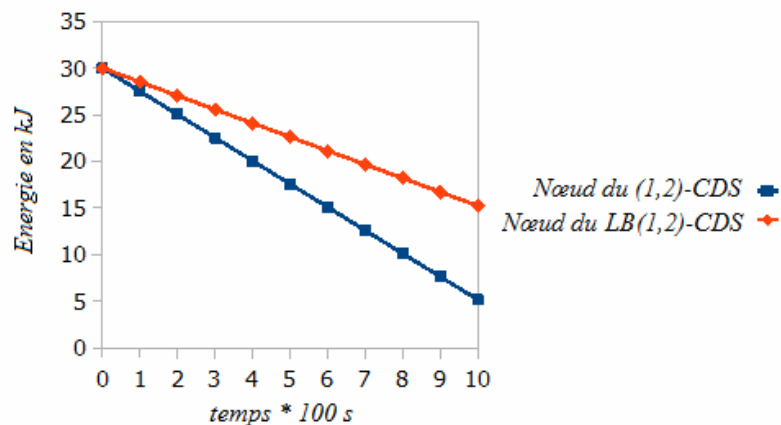
Figure 5.5. Evolution de l'énergie dans le nœud qui a fait plus de communication dans (1,2)-CDS avec une densité égale à 12 et une taille de paquet égale à 200 octets
