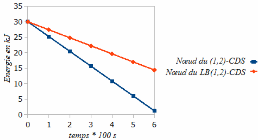
Figure 5.7. Evolution de l'énergie dans le nœud qui a fait plus de communication dans (1,2)-CDS avec une densité égale à 200 et une taille de paquet égale à 400 octets
