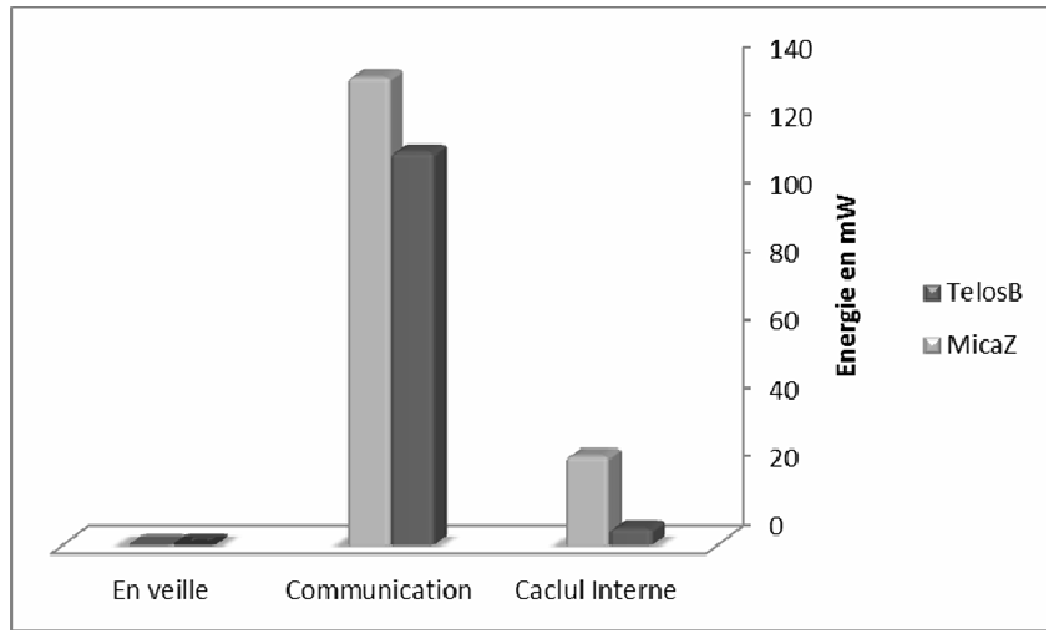
Figure 1.2. Comparaison de la consommation d'énergie du MicaZ et TelosB
