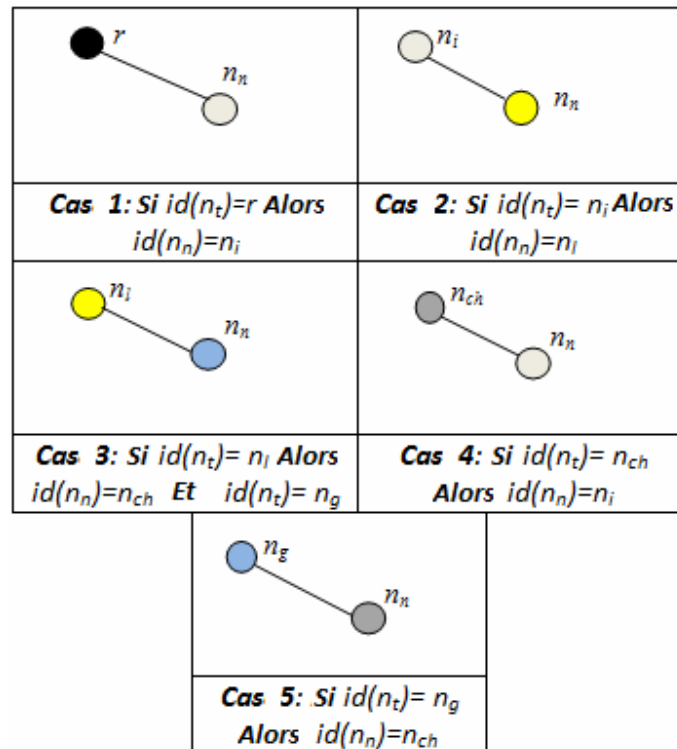
Figure 4.9. Différents cas d'identification d'un nouveau nœud
