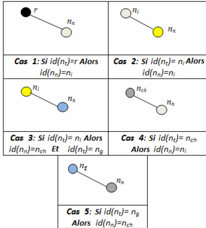
Figure 4.9. Différents cas d'identification d'un nouveau nœud
