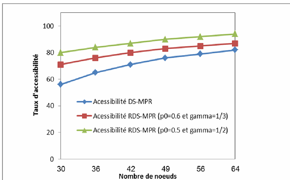
Figure 3.6. Comparaison de l'accessibilité de la méthode DS-MPR et RDS-MPR dans le modèle LNM
