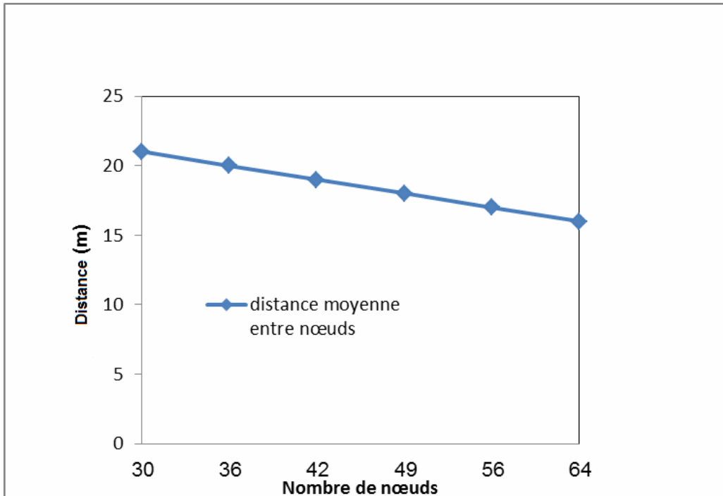
Figure 3.4. La distance moyenne entre les nœuds selon leur rayon de communication
