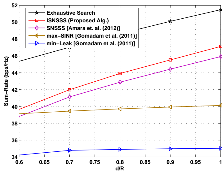
Figure 1.1: Scénario 1.2: Sum-rate moyen par rapport à d/R .
