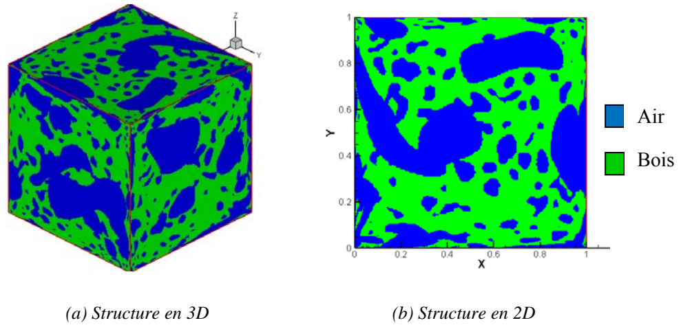
Figure IV. 11: Représentation morphologique du milieu bi phasique (Air-Bois)
