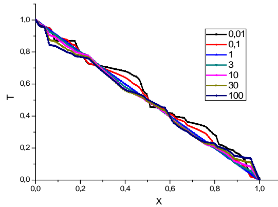
(a) Porosité=50%
