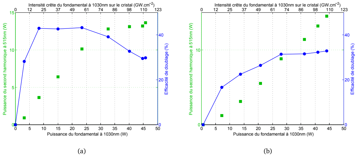
FIGURE 2.77 – Expérience de doublage de fréquence dans un cristal de BBO de 1mm. Le contraste en puissance est de 93% entre les trains à 100kHz et 77MHz, et l'ASE est inexistante. A pleine puissance ( \approx 50W ), le rayon à 1/e^2 dans le cristal de BBO est de 680\mu m , et la durée à mi-hauteur des impulsions dans le cristal est de 561fs déconvoluée par une gaussienne. L'intensité crête est évaluée à partir de ces valeurs quelle soit la puissance. Nous faisons varier la puissance du fondamental : (a) soit en changeant le pompage de l'amplificateur à forte puissance, (b) soit en tournant une lame demi-onde précédant une lame polarisante de type TFP, située après l'amplificateur à fibre barreau pompée à puissance constante pour fournir environ 60W à l'entrée des lames.
