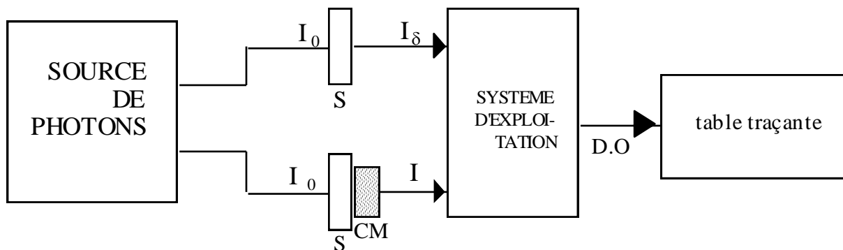
Figure V.10 : Mesure de l'absorption optique (schéma simplifié)
