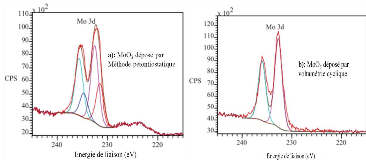
Figure II.7: Spectre XPS Mo3d 5/2 des couches minces de MoO 3 déposées par (a) méthode potentiostatique (b) voltamétrie cyclique [44]
