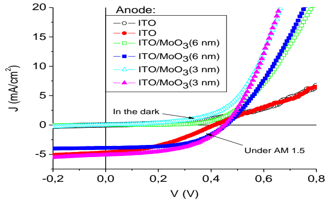
Figure II.6: Effet de l'épaisseur de MoO 3 sur les caractéristiques I-V des cellules sous illumination d'AM1.5 (100 mW/cm 2 )
