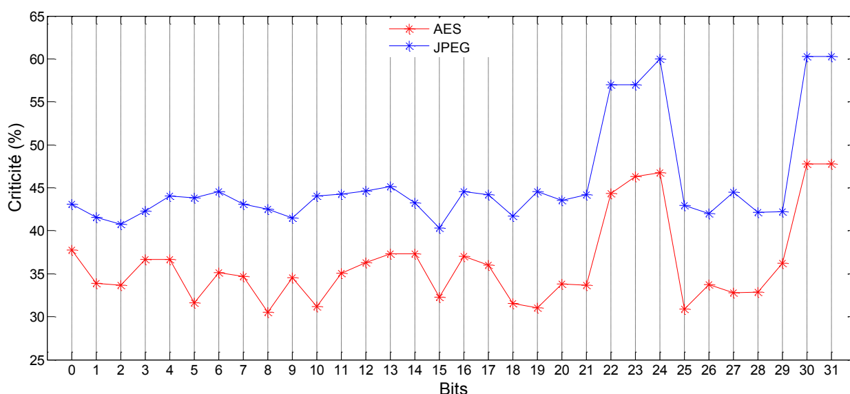
Figure IV-22 : Résultats de criticité des bits du registre d'instruction D_INST, obtenus avec l'analyse de durées de vie.
