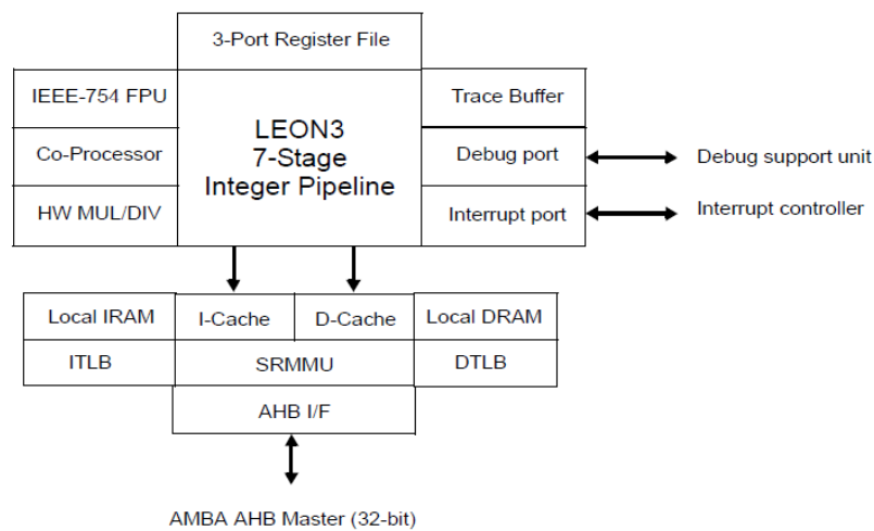
Figure III-3 : Schéma-bloc du processeur LEON3 [Gais. 13].
