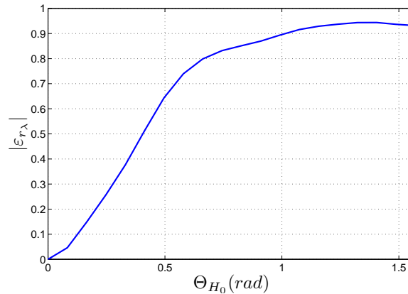
FIGURE 2.2.4 – Erreur relative sur la magnétostriction due à l'hypothèse de susceptibilité isotrope du matériau en fonction de la direction du champ magnétique
