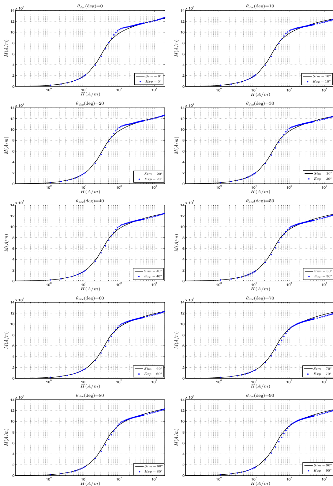
FIGURE 4.3.1 – Comparaison entre expérimentation et simulation de l'aimantation multidirectionnelle
