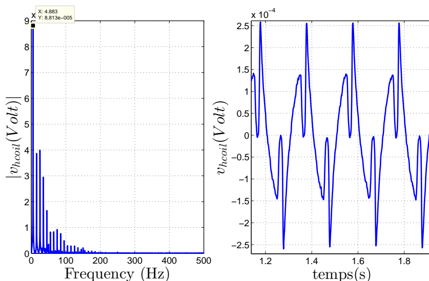
FIGURE 4.1.7 – Signal de sortie du h-coil distordu
