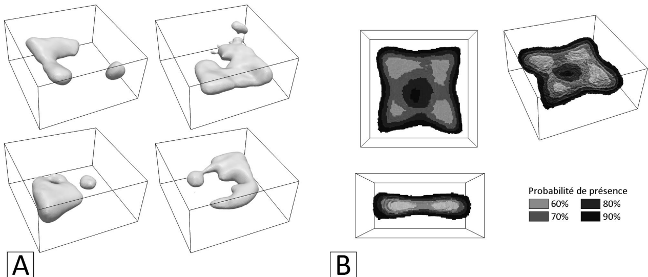
FIGURE 1.10 – Étude de la morphologie des macropores par segmentation de micro-tomographies X (annexe A). A : Quelques exemples. B : Localisation moyenne et enveloppes de probabilité de présence.
