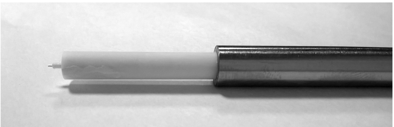
FIGURE 3.24 – Effecteur utilisé lors d'essais de push-out afin de pousser des bundles de 200µm.
