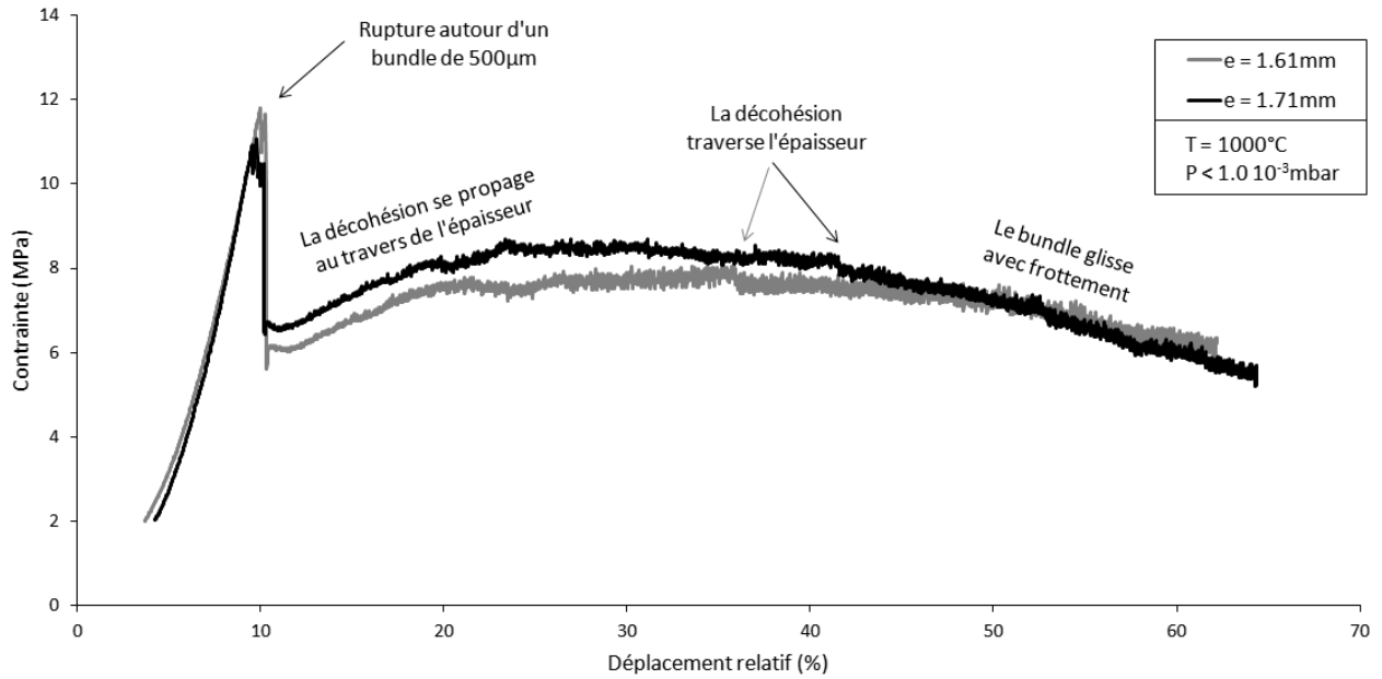
FIGURE 3.14 – Essais de push-out sur baguette Z à 1000°C. Ces essais n'ont pas permis de dégager une baguette Z mais un bundle de 500µm.
