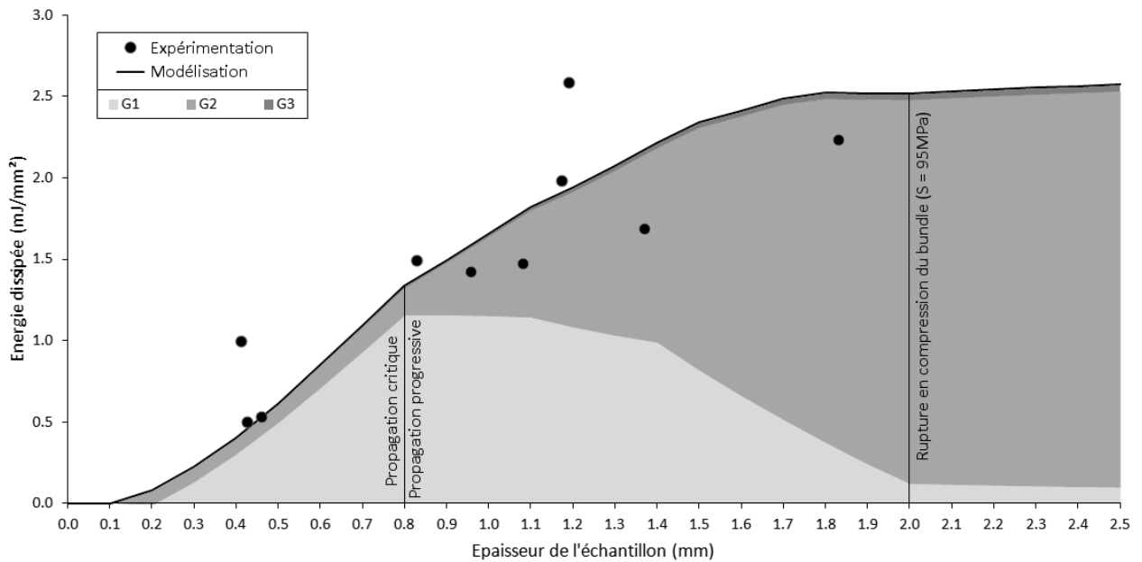
FIGURE 3.34 – Calcul de l'énergie dissipée totale d'après le modèle et confrontation aux valeurs expérimentales.
