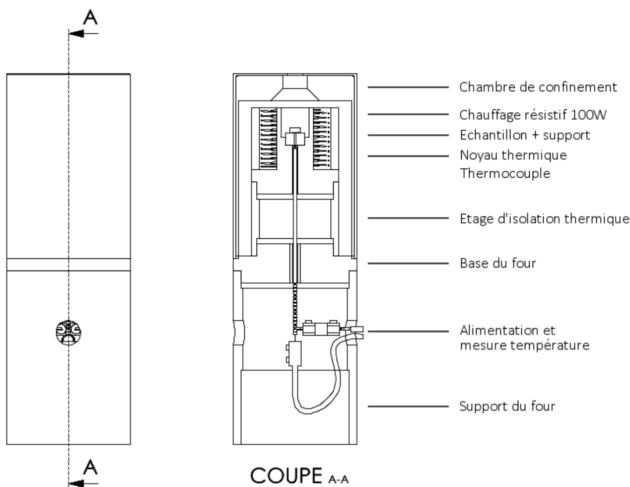
FIGURE C.6 – Vue en coupe du four, annotée du nom de ses constituants.
