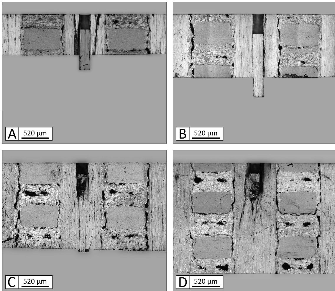
FIGURE 3.27 – Coupes transverses des échantillons après essais de push-out sur bundles de 200µm à différentes épaisseurs. A : e=0.788\text{mm} , B : e=1.17\text{mm} , C : e=1.65\text{mm} et D : e=2.08\text{mm} .
