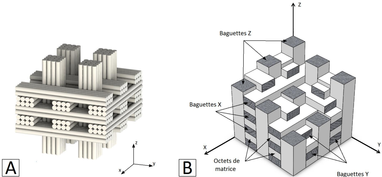
FIGURE 5 – Structure et composition du 3D C/C. A : la préforme avant la densification. B : la structure et les méso-constituants du composite 3D C/C.
