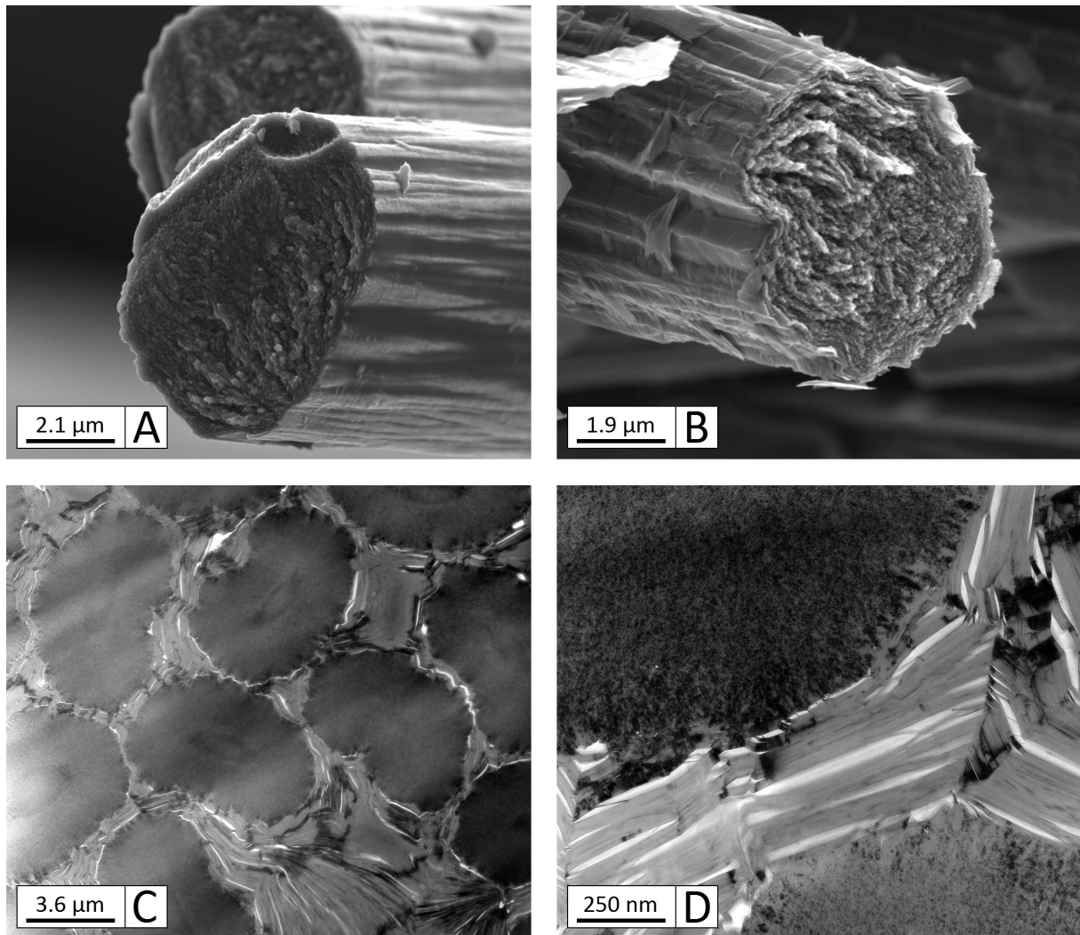
FIGURE 3.2 – A,B : micrographies MEB de fibres M40, respectivement brutes et extraites d'une baguette. C,D : images MET fond clair d'une tranche de baguette [Lachaud, 2006].
