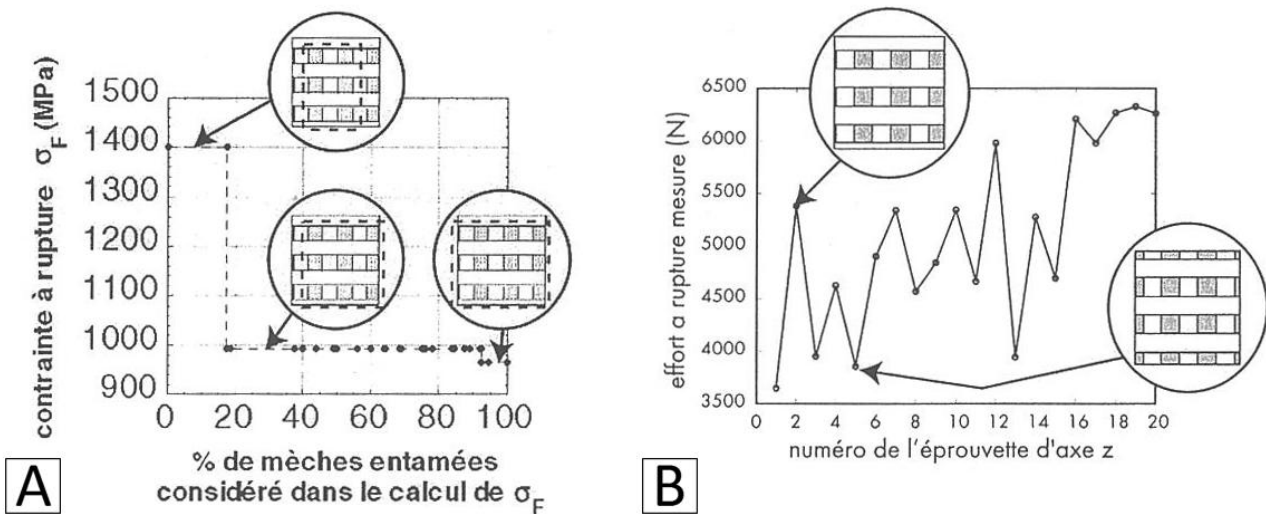
FIGURE 2.7 – A : Influence de la section de l'éprouvette sur la contrainte à rupture. B : Disparités des contraintes à rupture et section des éprouvettes [Davy, 2001].
