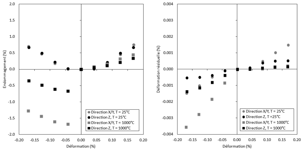
FIGURE 4.26 – Endommagement et déformation résiduelle extraits des simulations d’essais de traction/compression cyclés suivant X/Y et Z, à différentes températures.
