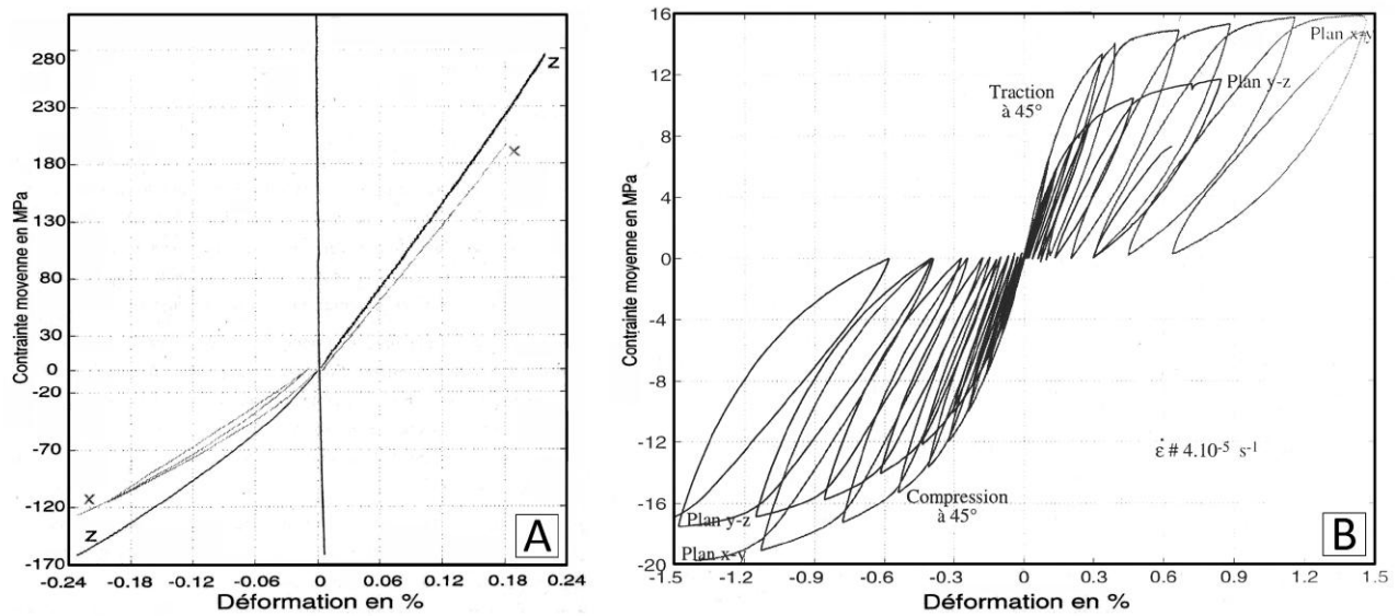
FIGURE 2.8 – Essais macroscopiques sur le C/C BLOC300 [Gratton, 1998]. A : Tractions/compressions suivant les axes de tissage. B : Tractions/compressions en dehors des axes de tissage.
