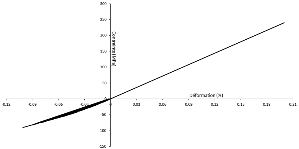
FIGURE 2.1 – Essais de traction et de compression cyclés sur le composite 3D C/C et suivant les axes de tissage [Poss, 1982]
