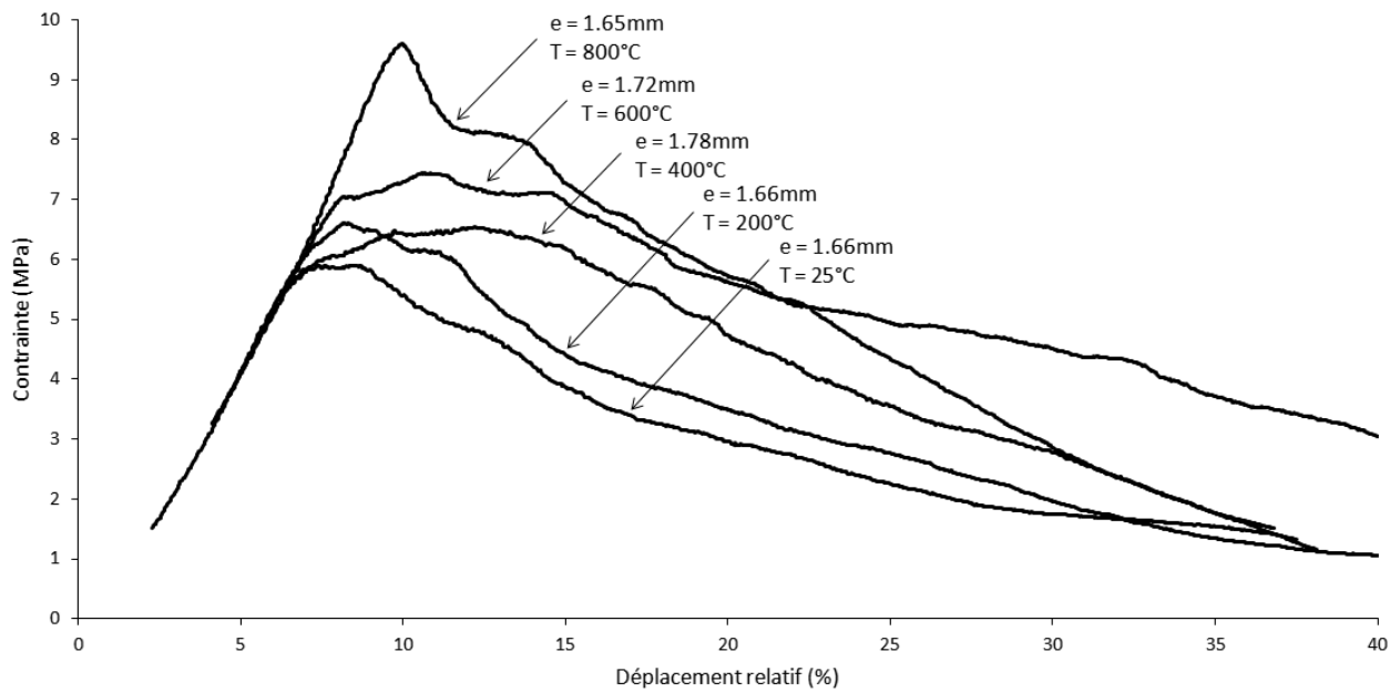
FIGURE 3.13 – Influence de la température sur les essais de push-out sur baguettes Z.
