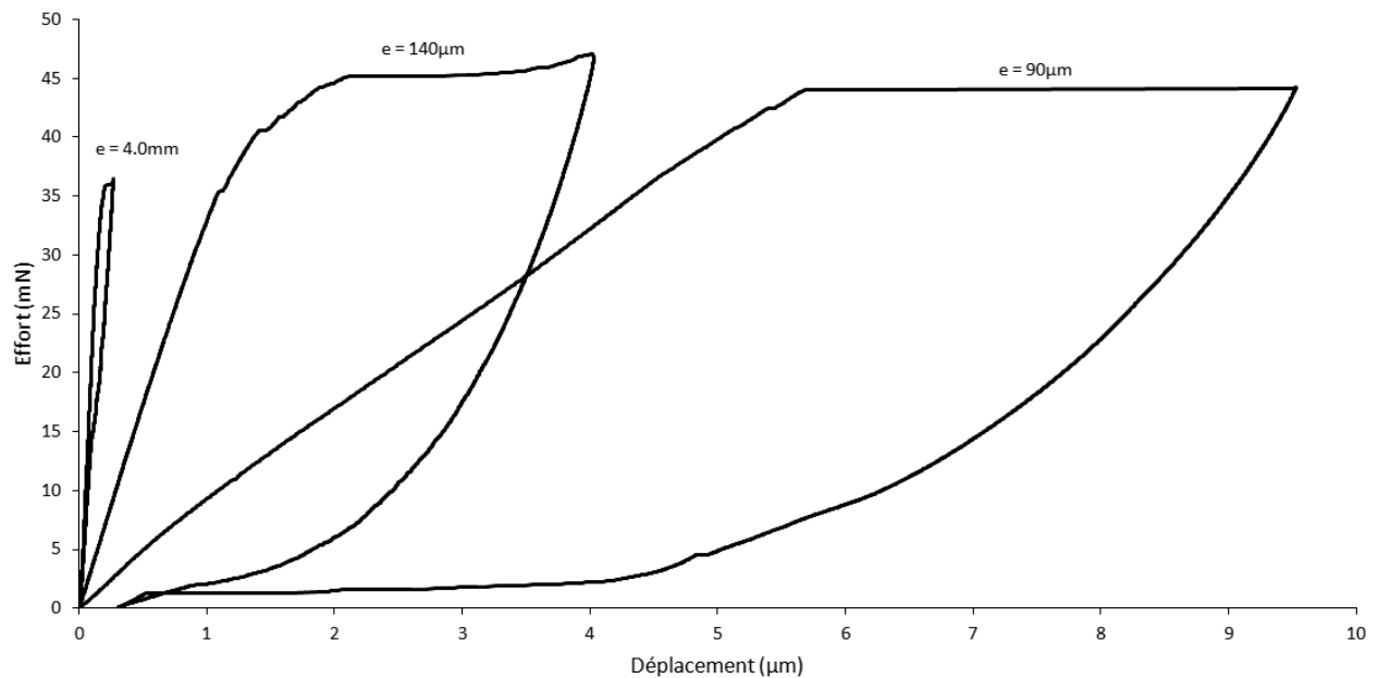
FIGURE 3.22 – Essais de push-in sur des échantillons d'épaisseurs de 0.090mm, 0.140mm et 4.0mm.
