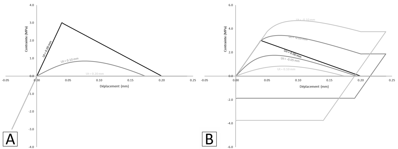
FIGURE G.4 – Effet du couplage sur le comportement du modèle cohésif en modes I (A) et II (B).
