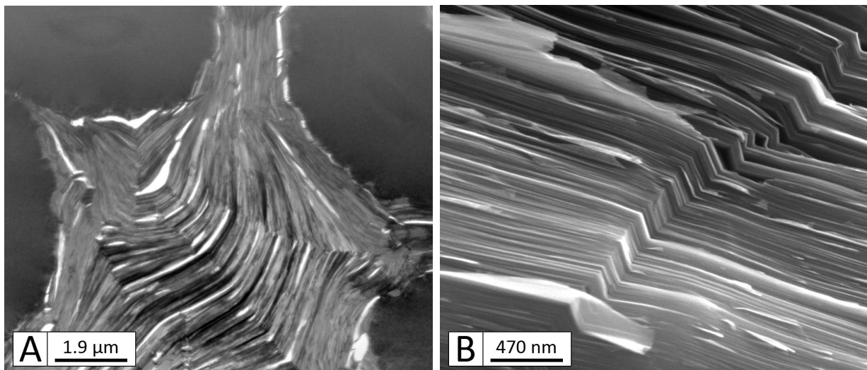
FIGURE 1.7 – A : Image issue d’un microscope électronique à transmission (MET, annexe A) en mode fond clair [Lachaud, 2006]. B : image MEB (électrons secondaires) d’un faciès de rupture de la matrice au sein des baguettes.
