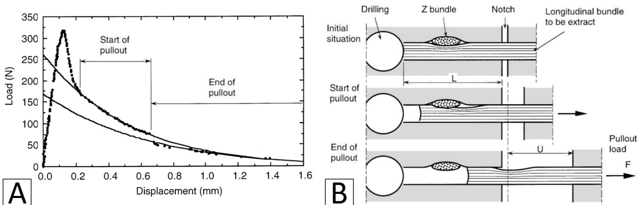
FIGURE 3.18 – Essais de pull-out à l'ambiante sur des renforts d'un 2.5D C/C [Valette et al., 2002]. A : Courbe effort-déplacement. B : Mécanismes de déverrouillage.
