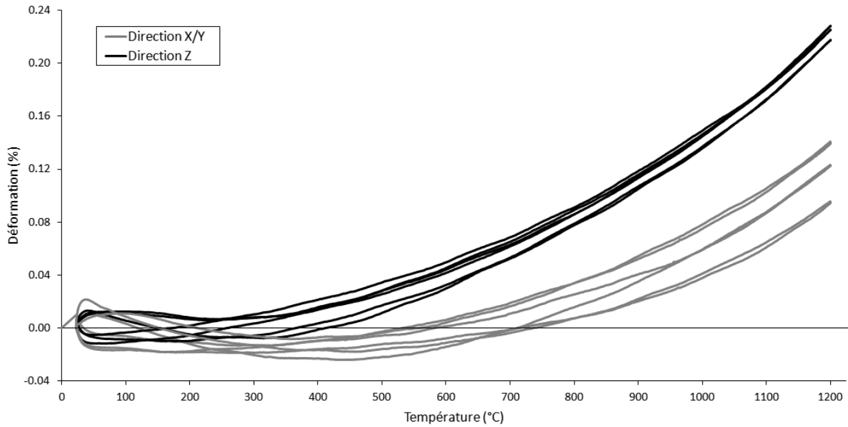
FIGURE 2.23 – Dilatation thermique du composite : mesures sur un échantillon de 6mm.
