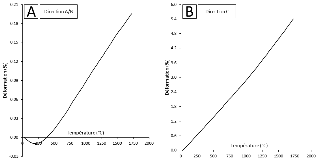
FIGURE 2.28 – Expansion thermique du graphite monocristallin dans les directions a/b (A) et c (B) [Fitzer and Manocha, 1999].
