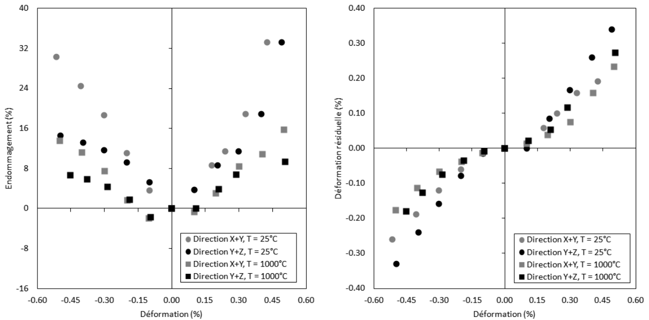
FIGURE 4.34 – Endommagement et déformation résiduelle extraits des simulations d’essais de traction/compression cyclés suivant X+Y et Z+X/Y+Z, à différentes températures.
