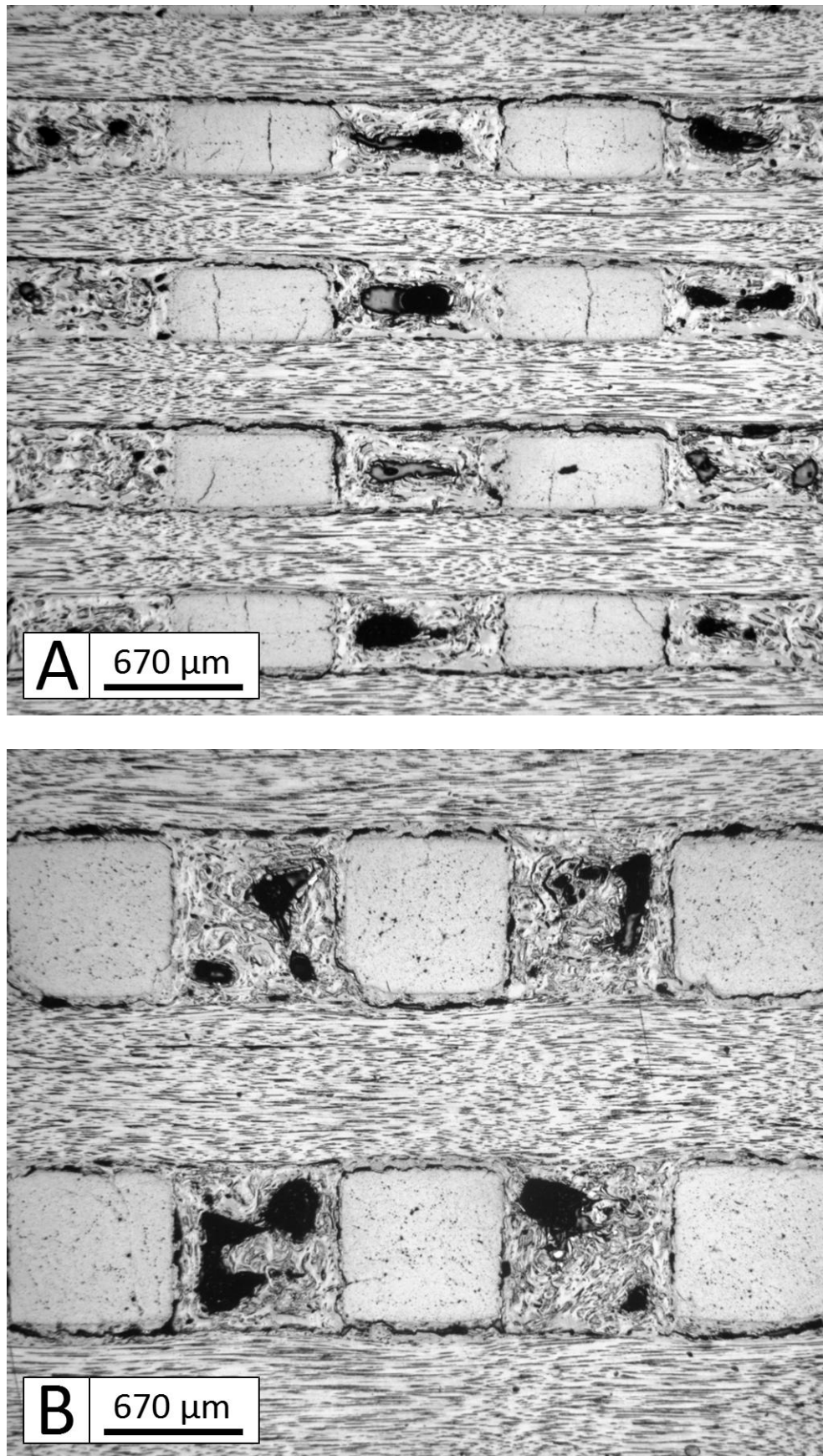
FIGURE 1.1 – Micrographies optiques d'un échantillon poli mécaniquement. A : Coupe normale aux baguettes X, passant par le milieu des baguettes Y. B : Coupe normale aux baguettes Z, passant par le milieu des baguettes X.
