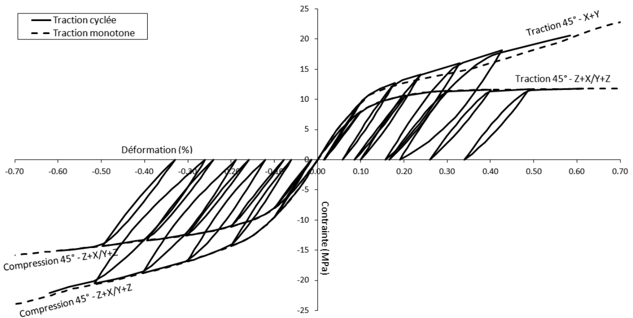
FIGURE 4.35 – Rassemblement des simulations d’essais de traction/compression en dehors des axes de tissage sur le 3D C/C à l’ambiante, cyclés et monotones.
