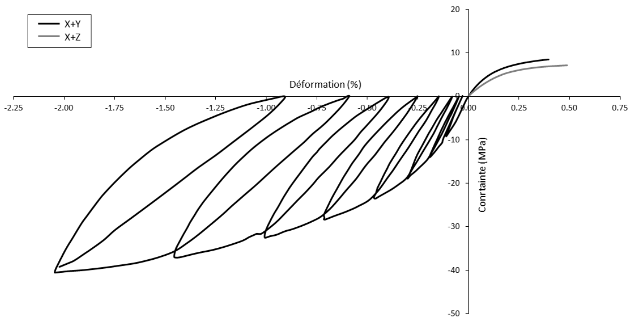
FIGURE 2.2 – Essais de traction et de compression cyclés sur le composite 3D C/C et en dehors des axes de tissage [Poss, 1982].
