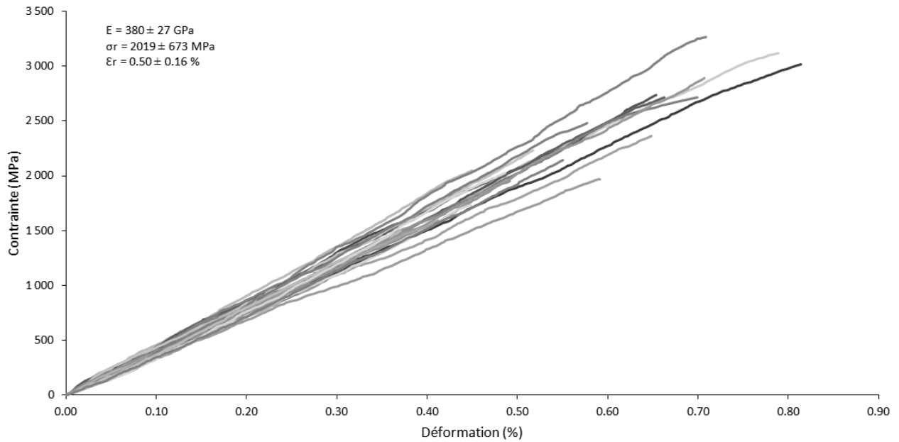
FIGURE 2.12 – Essais de traction sur fibres à l’ambiante [Carpier, 2015, Benezech, 2016].
