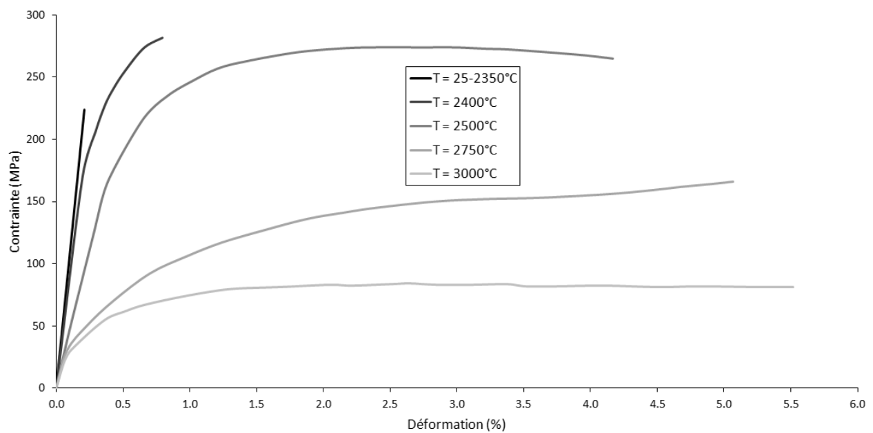
FIGURE 2.17 – Essais de traction Z à haute température sur le composite 3D C/C. [CEA, 2004]
