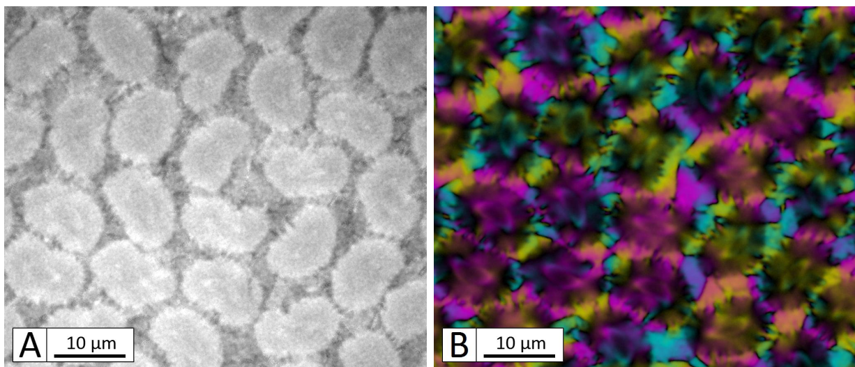
FIGURE G.8 – Micrographie (A) et cartographie d'anisotropie et d'orientation (B) issues d'analyses sous lumière polarisée des fibres et de la matrice au sein des baguettes. Des légendes sont fournies en annexe A.
