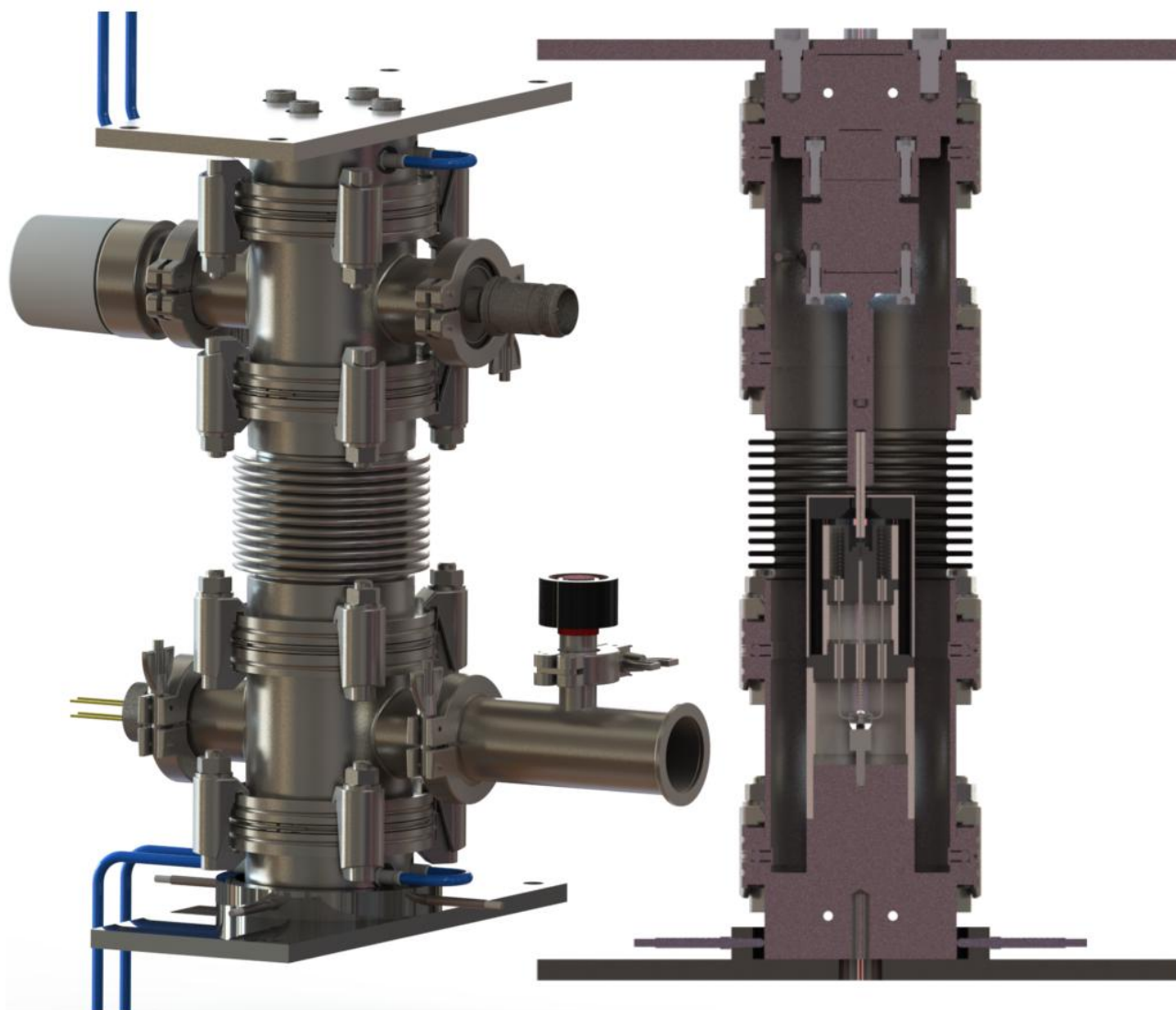
FIGURE C.2 – Vue d'ensemble du dispositif de push-out à haute température.
