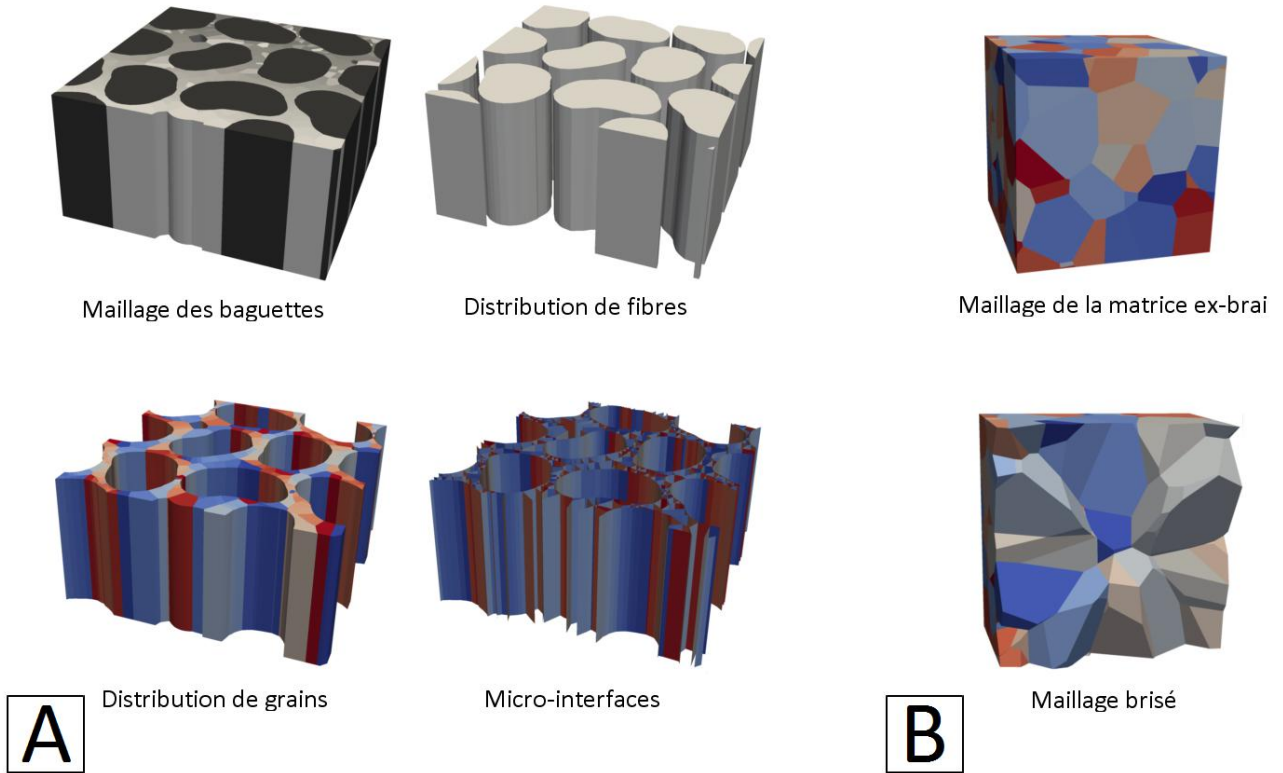
FIGURE 5.49 – Les différents modèles microscopiques proposés. A : Pour les baguettes, avec les fibres et la matrice. B : Pour les octets avec la matrice.
