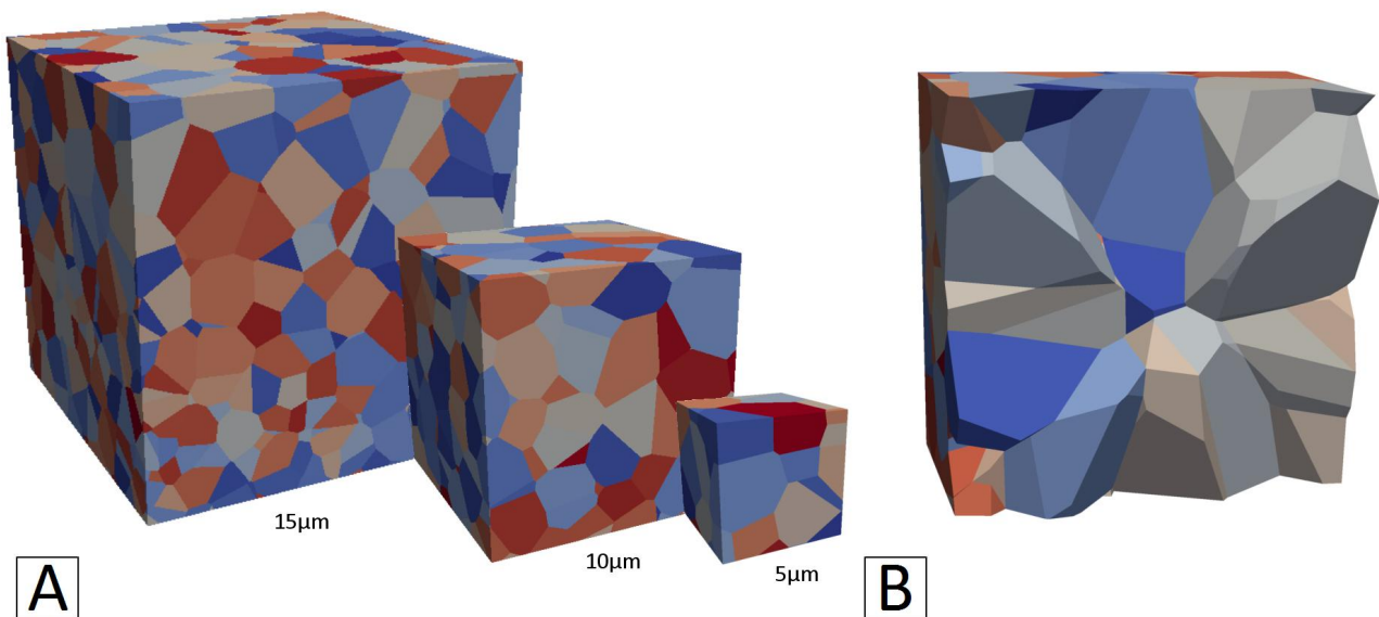
FIGURE G.6 – Proposition de maillages représentant de la morphologie de la matrice ex-brai. A : Différentes tailles de maillages. B : Vue brisée présentant les grains.
