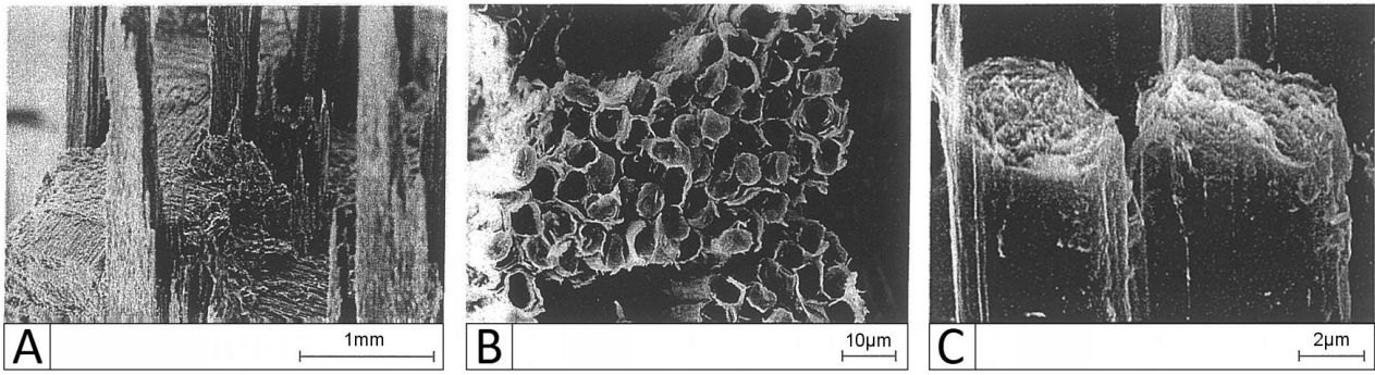
FIGURE 2.5 – Faciès de rupture après traction suivant Z [Davy, 2001]. Observations à l'échelle du composite (A), des baguettes (B) et des fibres (C).
