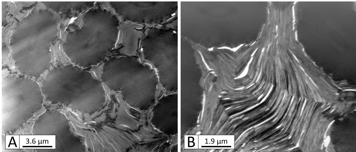
FIGURE G.7 – Images MET des baguettes montrant la texture des fibres et de la matrice [Lachaud, 2006], à faible (A) et fort (B) grossissement.
