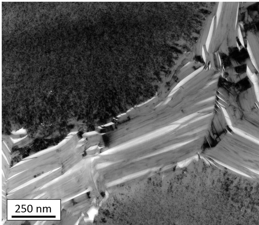
FIGURE G.1 – Observation au MET de l'interface fibre/matrice.
