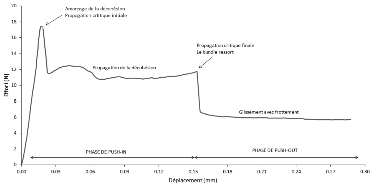
FIGURE 3.28 – Push-out sur bundles de 200µm avec un échantillon de 1.7mm d'épaisseur.
