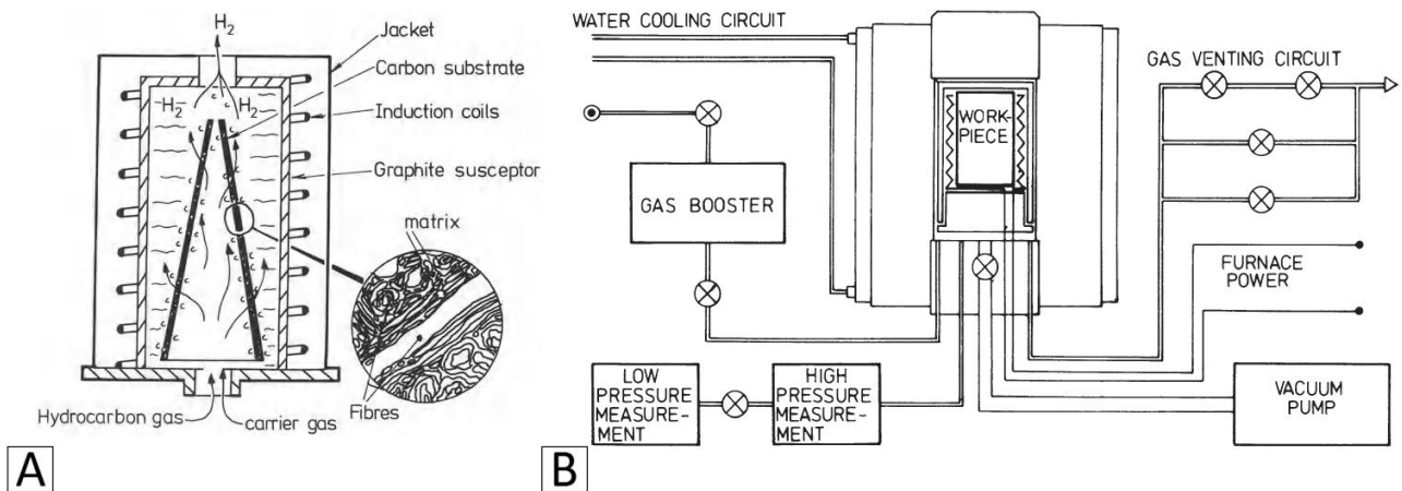
FIGURE 4 – Schéma des dispositifs de densification pour les principales voies de densification des C/C, la CVD/CVI (ici isotherme, A) et la PIP (B) [Savage, 1993].
