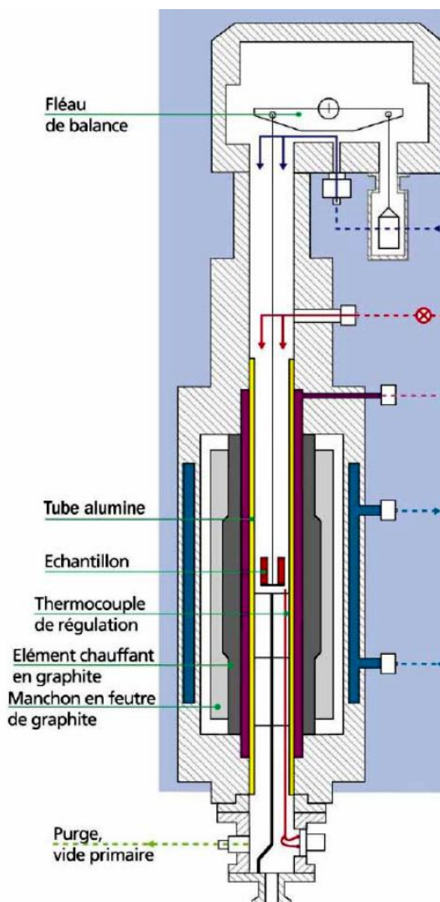
FIGURE D.1 – Le dispositif Setsys 2400 permettant de mesurer la dilatation d'échantillons.
