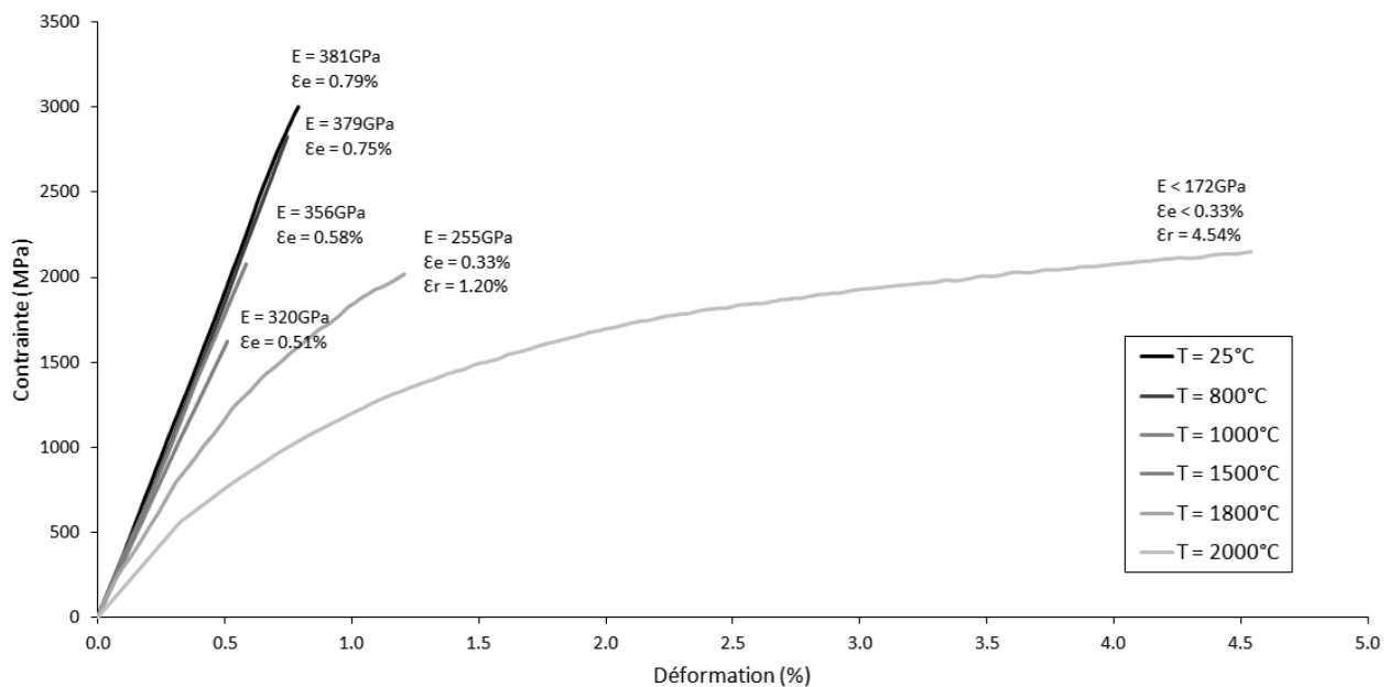
FIGURE 2.20 – Essais de traction sur fibres à haute température [Carpier, 2015, Benezech, 2016].
