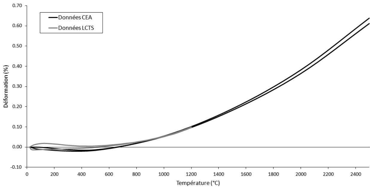
FIGURE 2.24 – Dilatation thermique du composite : mesures fournies par le CEA.
