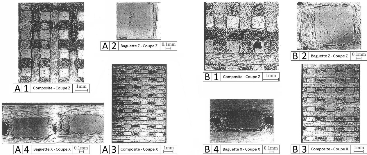
FIGURE 2.6 – Micrographies de coupes polies d'éprouvettes ante-mortem (A) et post-mortem (B) [Davy, 2001].
