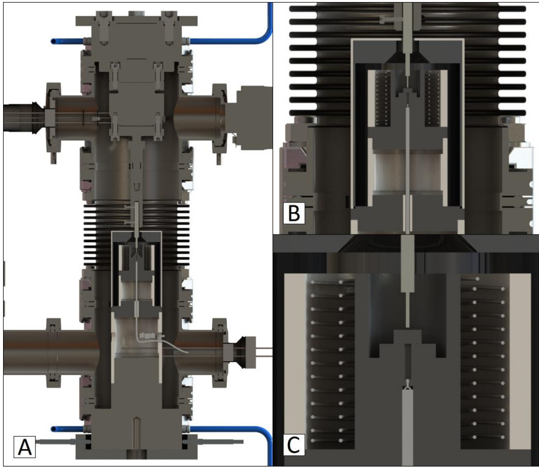
FIGURE 3.12 – Dispositif de push-out HT. A : Le système complet composé de l'effecteur, du système de chauffe et de l'enceinte à vide. B : Un agrandissement sur le four. C : Un agrandissement sur la zone d'essai.
