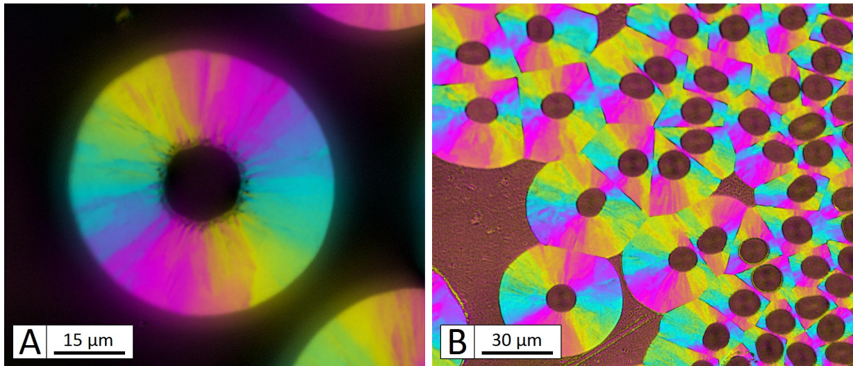
FIGURE G.14 – Cartographies d'anisotropie et d'orientation issues d'analyses sous lumière polarisée d'un dépôt CVI de pyrocarbone laminaire rugueux sur préforme tissée de fibres de carbone, à fort (A) et à faible (B) grossissement. Des légendes sont fournies en annexe A.
