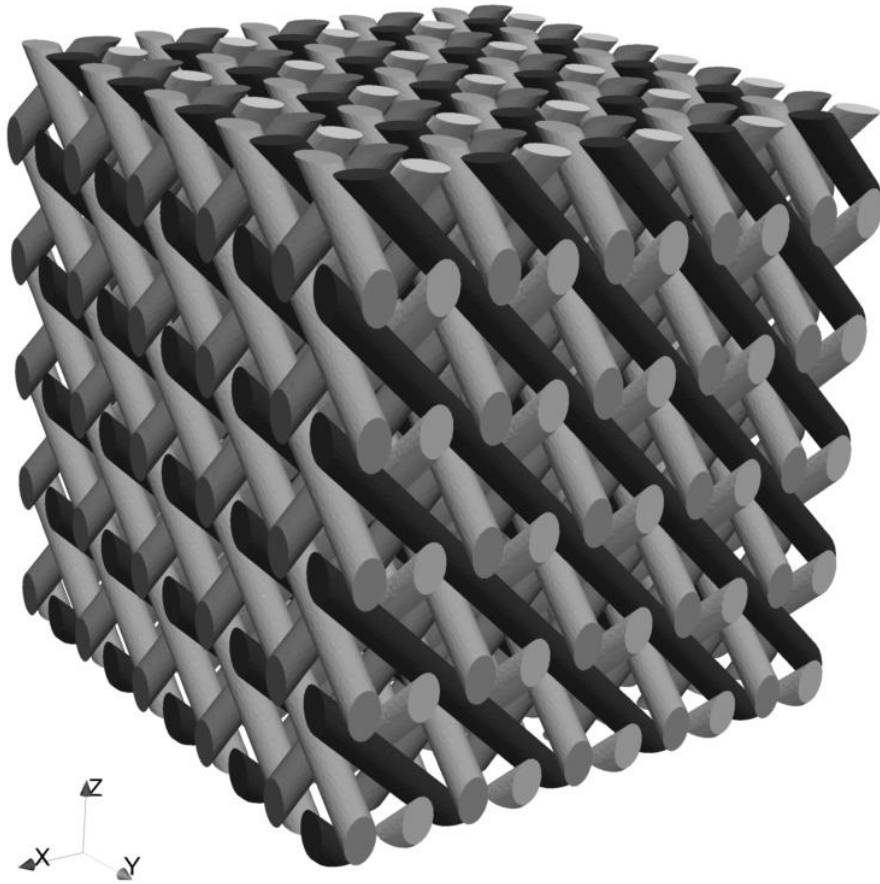
FIGURE E.1 – Maillage des renforts (baguettes) du modèle EF macroscopique pour le composite 4D C/C.
