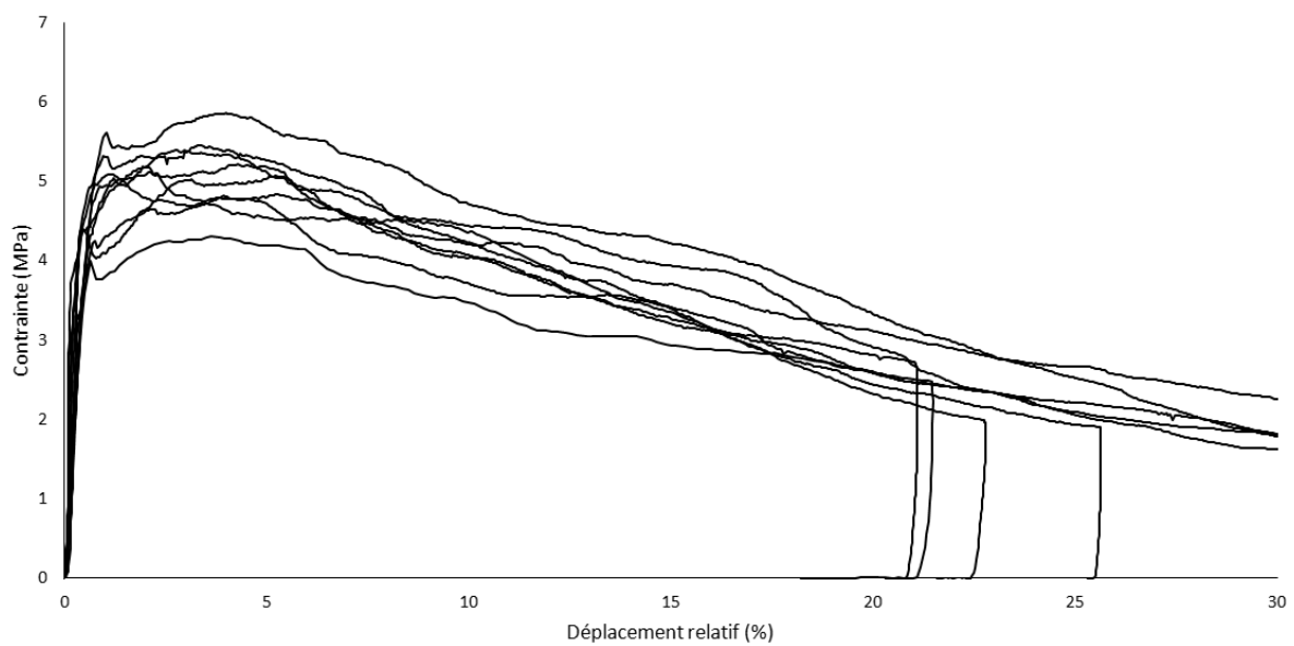
FIGURE 3.9 – Quelques courbes issues d'essais représentatifs de push-out sur baguettes Z.
