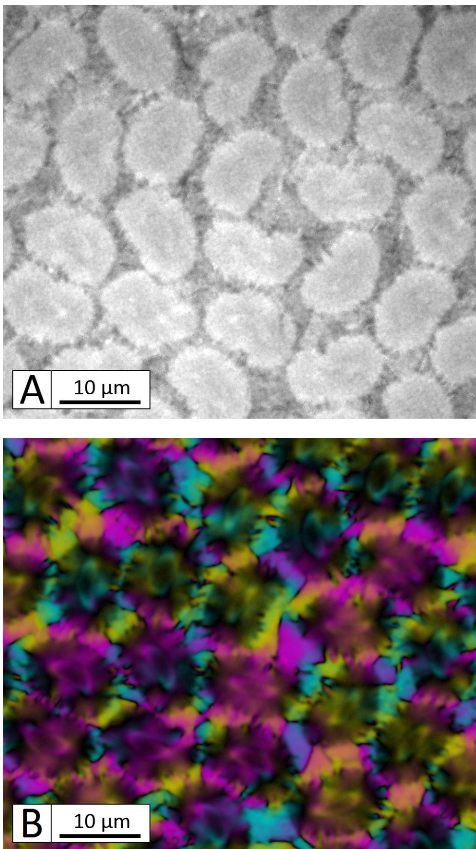
FIGURE 1.4 – Analyse de micrographies optiques sous lumière polarisée (annexe A) d'une coupe normale à une baguette Z. A : Microscopie classique. B : Cartographie d'anisotropie et d'orientation.
