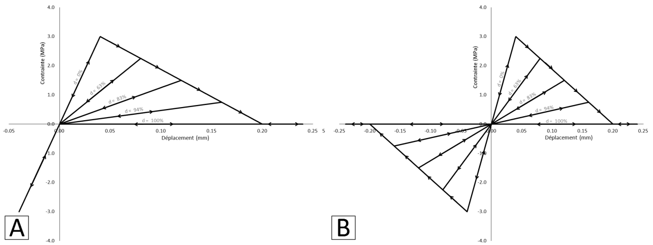
FIGURE G.3 – Comportement endommageable du modèle cohésif en modes I (A) et II (B) purs.
