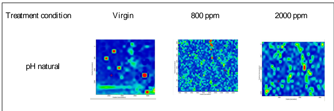
(d): H_{880}/H_{1185}
