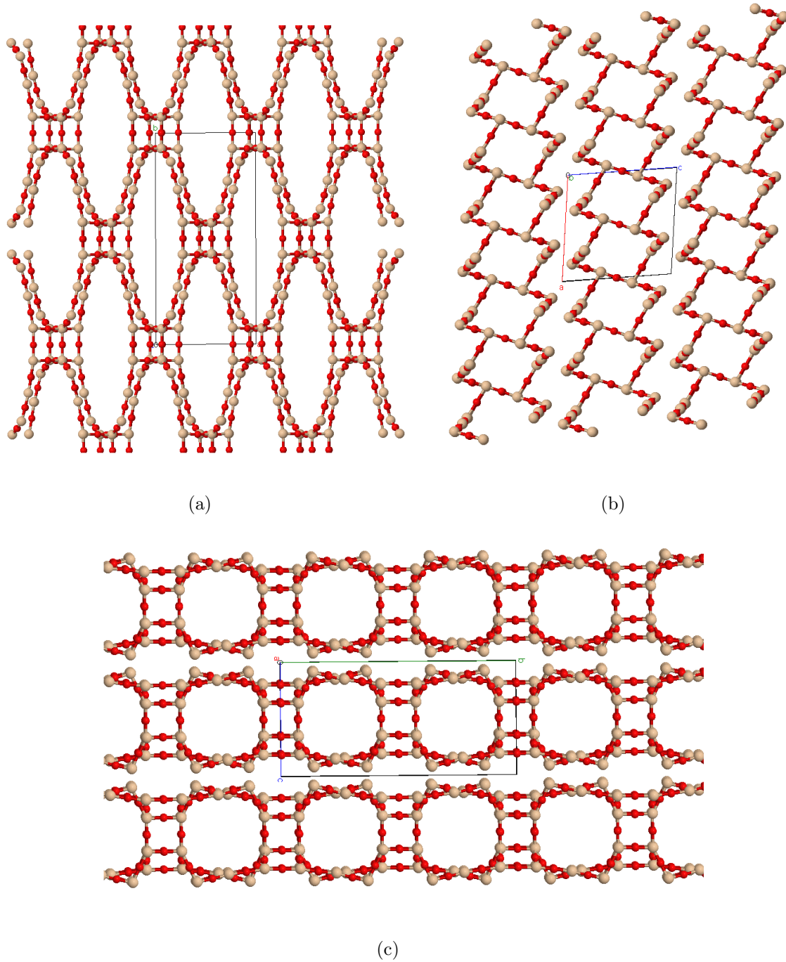
FIGURE 4.26 – Cinquième topologie sélectionnée avec MEGA-HZ et la formulation 2 à partir des paramètres de RTH avant la minimisation (UFF) et avant l'optimisation (BS).
