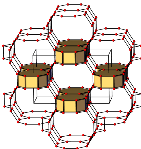
FIGURE 4.16 – La deuxième nouvelle topologie HZM\#2 trouvée par P-GHAZ après minimisation (UFF) et après optimisation (BS). Les CBU d4r sont absents entre les unités d8r par rapport à la première topologie inconnue décrite ci-dessus. Les atomes d'oxygène ont été omis pour des raisons de clarté.
