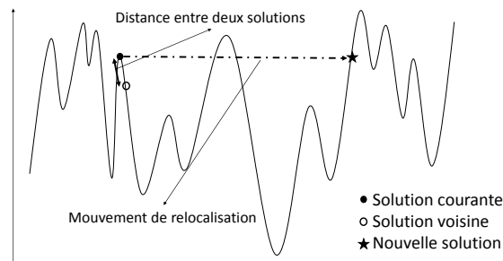
FIGURE 3.2 – Mouvement de relocalisation en utilisant la distance
